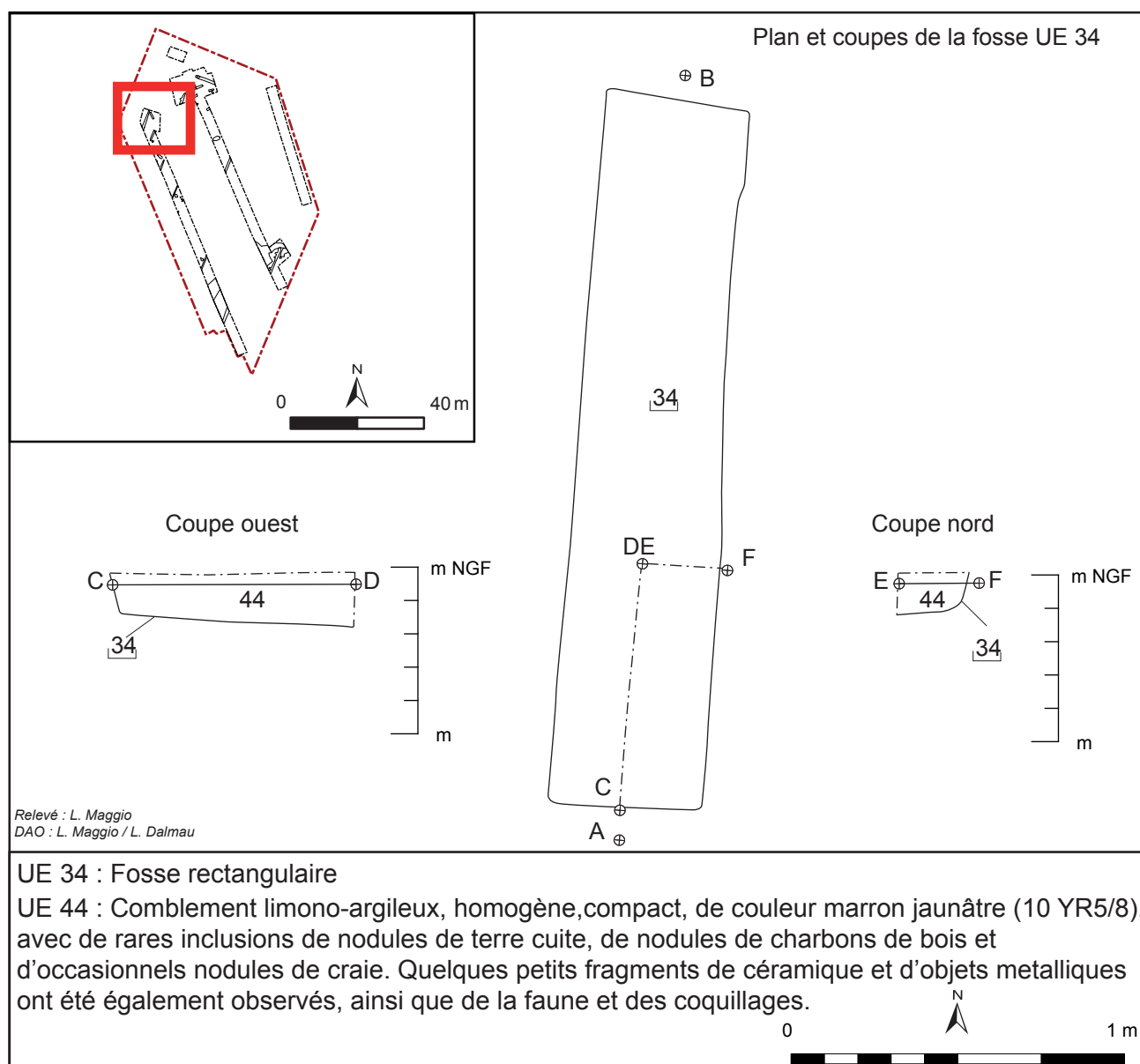
Fig. 17 : Achicourt, "la briqueterie" - rue Louise Michel : Plan et coupes de la fosse UE 34, L. Dalmau - CDA CG62.
