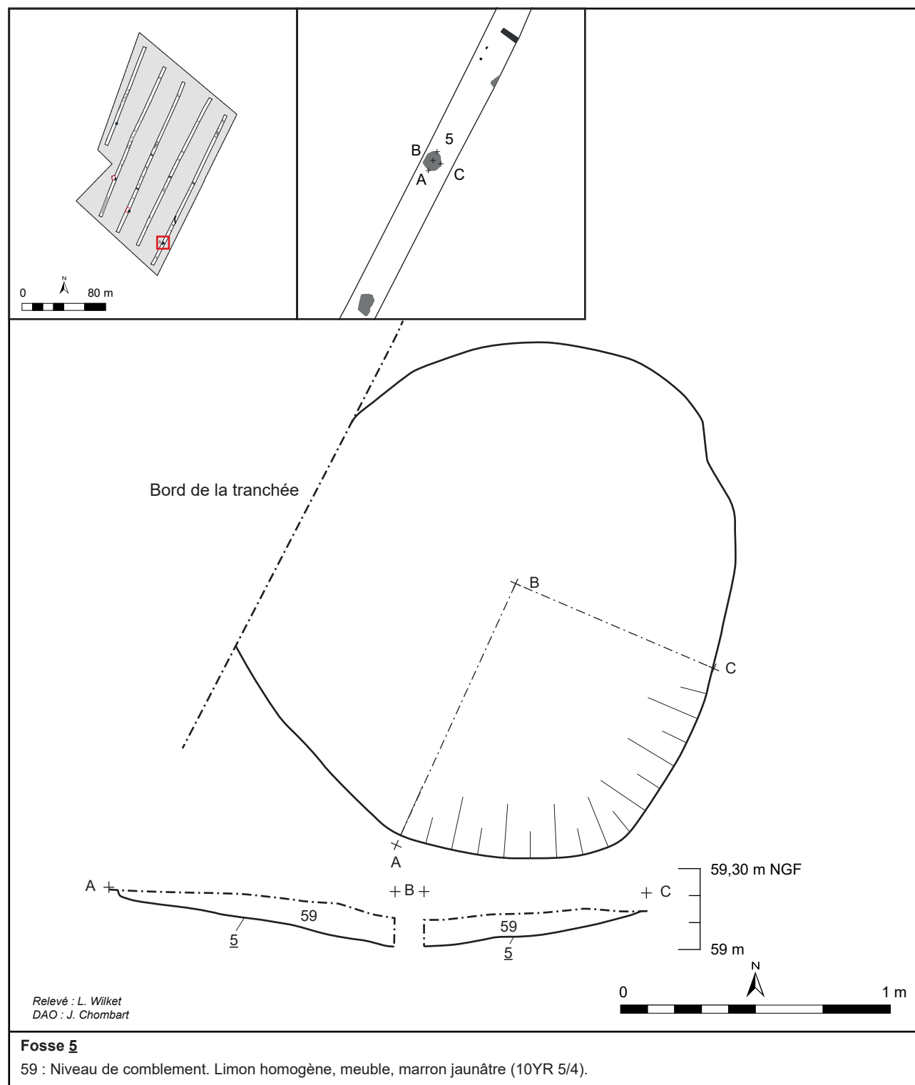
Fig. 14 : Bully-les-Mines, «ZAC du Chemin des Hirondelles (secteur 2)», plan et coupes de la fosse 5, J. Chombart - DA, CD 62.
