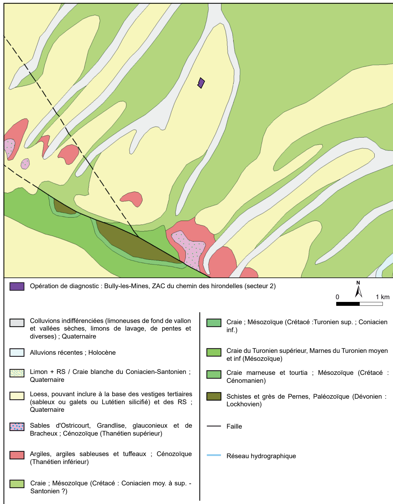
Fig. 5 : Bully-les-Mines, «ZAC du Chemin des Hirondelles (secteur 2)», extrait de la carte géologique au 1/50 000e harmonisée (Lacquement et al. 2004 ; BRGM-Infoterre 2021), J. Chombart - DA, CD 62.
