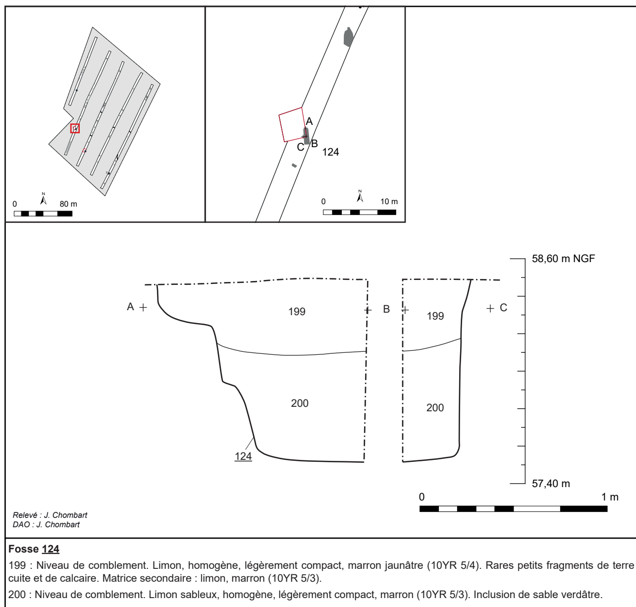
Fig. 15 : Bully-les-Mines, «ZAC du Chemin des Hirondelles (secteur 2)», coupes de la fosse 124, J. Chombart - DA, CD 62.
