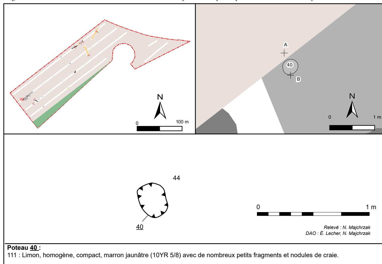
Fig. 19 : Dainville, ZAC Dainville-Achicourt-le Picotin, plan et coupe du poteau 40, DAO : N. Majchrzak - DA, D 62..
