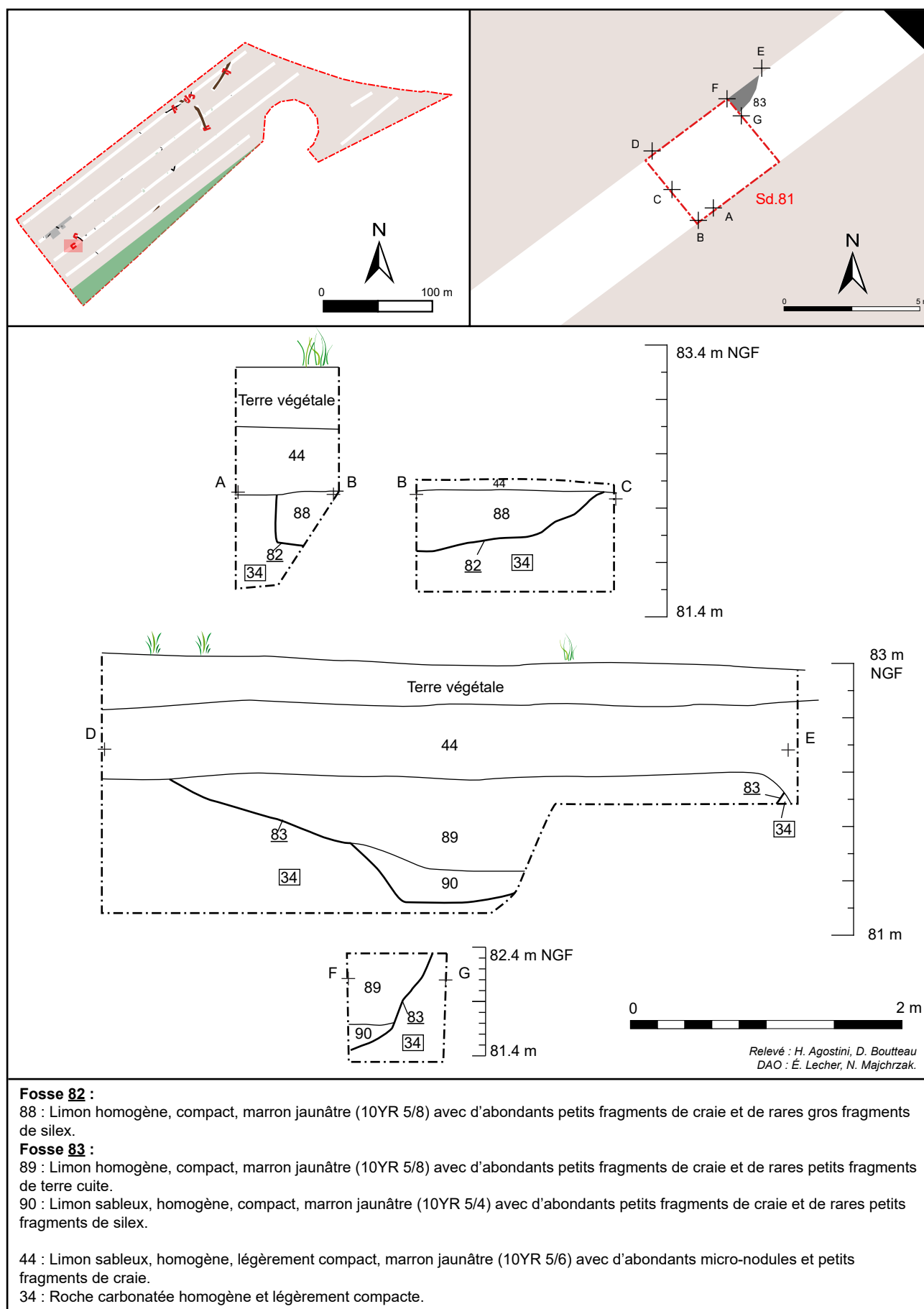
Fig. 21 : Dainville, ZAC Dainville-Achicourt-le Picotin, Coupe des fosses 82 et 83, DAO : N. Majchrzak - DA, D 62.
