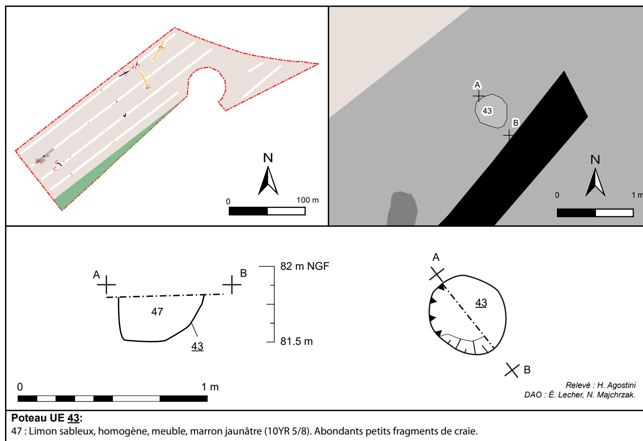
Fig. 20 : Dainville, ZAC Dainville-Achicourt-le Picotin, Plan et coupe du poteau 43, DAO : N. Majchrzak - DA, D 62.
