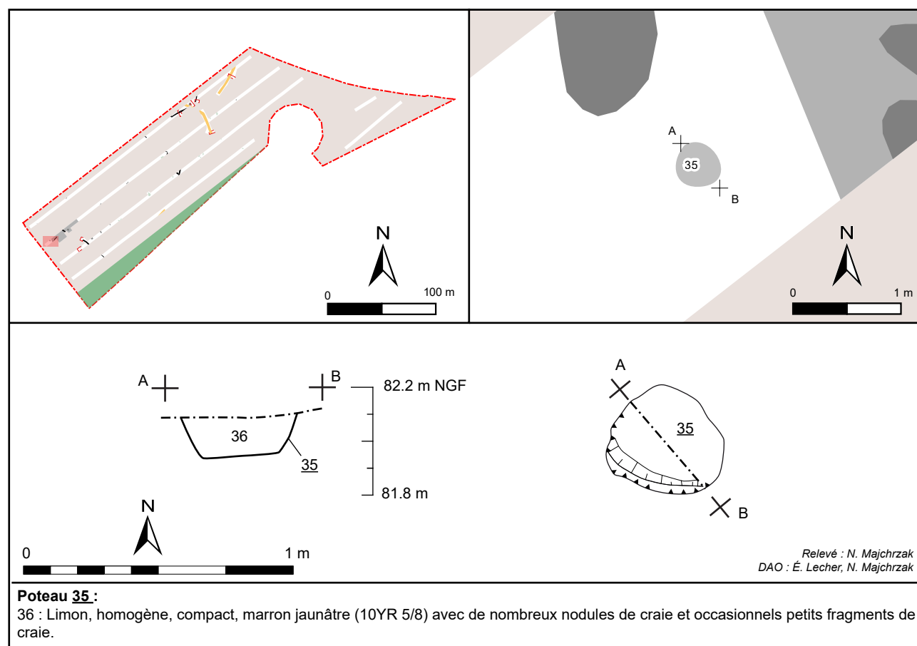
Fig. 18 : Dainville, ZAC Dainville-Achicourt-le Picotin, plan et coupe du poteau 35, DAO : N. Majchrzak - DA, D 62..
