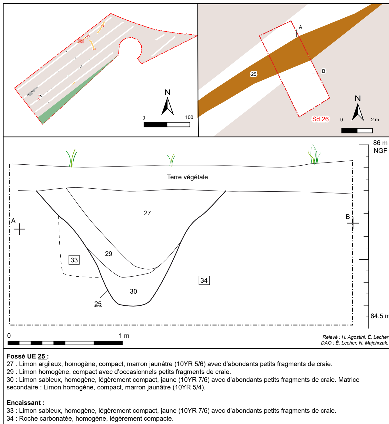
Fig. 10 : Dainville, ZAC Dainville-Achicourt-le Picotin, plan et coupe du fossé 25, sd 26, DAO : N. Majchrzak - DA, CD 62.
