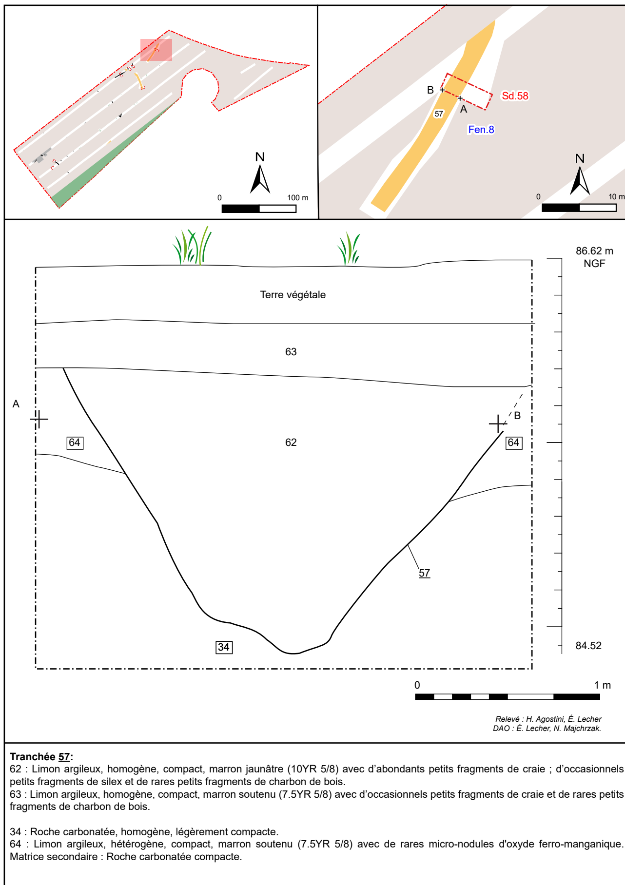
Fig. 30 : Dainville, ZAC Dainville-Achicourt-le Picotin, Coupe de la tranchée 57, DAO : N. Majchrzak - DA, D 62.
