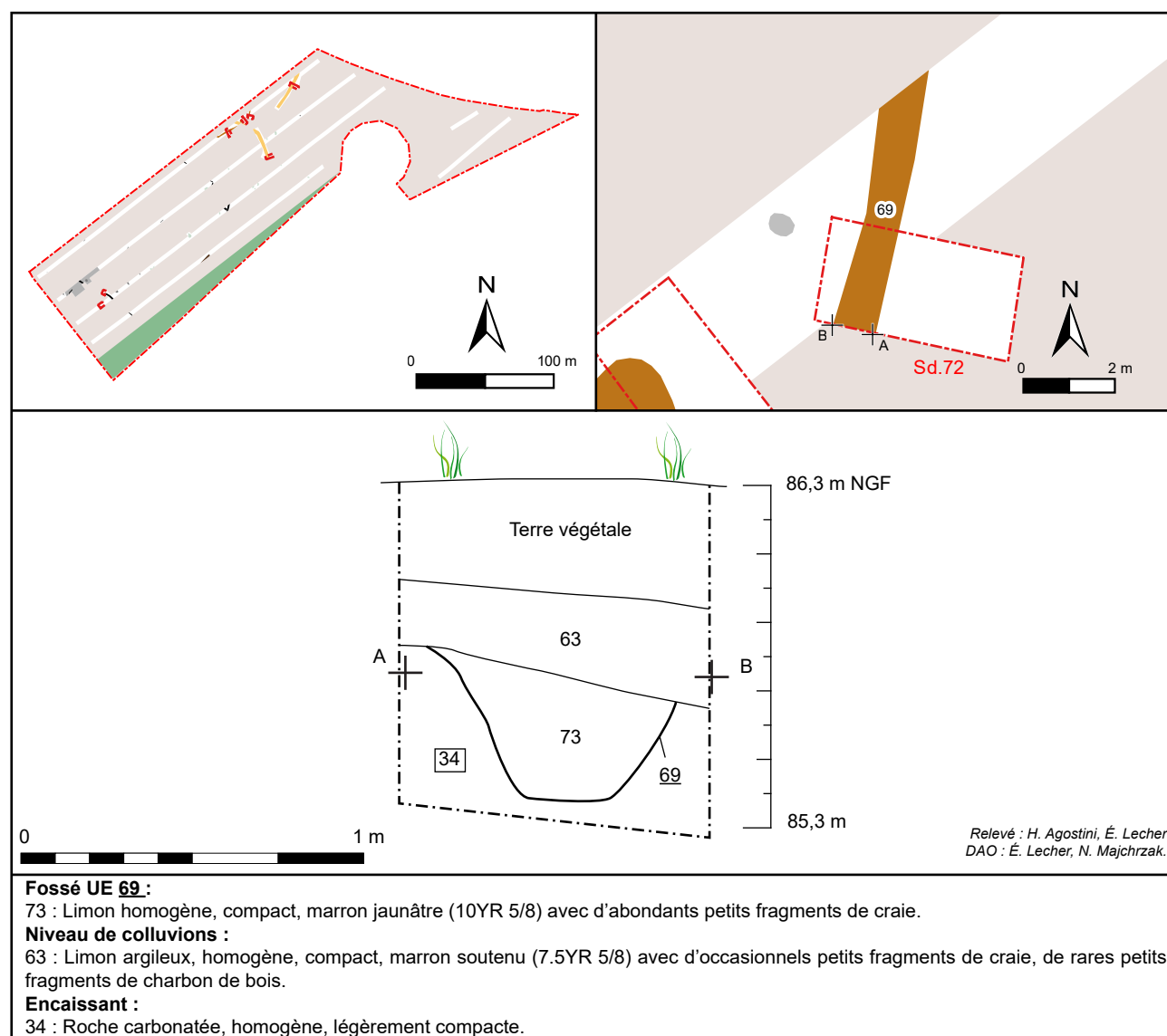
Fig. 11 : Dainville, ZAC Dainville-Achicourt-le Picotin, plan et coupe du fossé 69, sd 72, DAO : N. Majchrzak - DA, CD 62.
