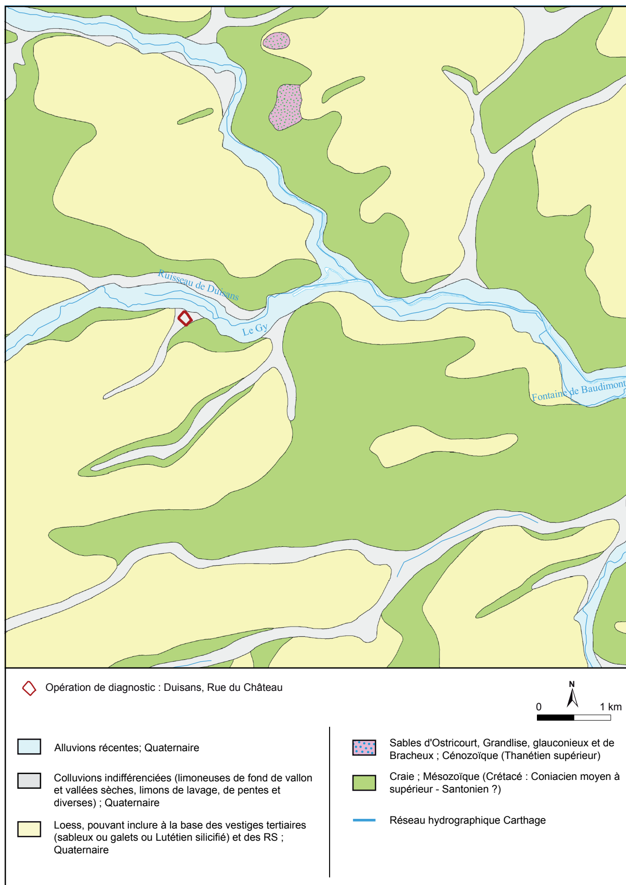
Fig. 5 : Duisans, Rue du Château, Carte sur l'environnement géologique de la fouille, L. Wilket - DA, CD 62.
