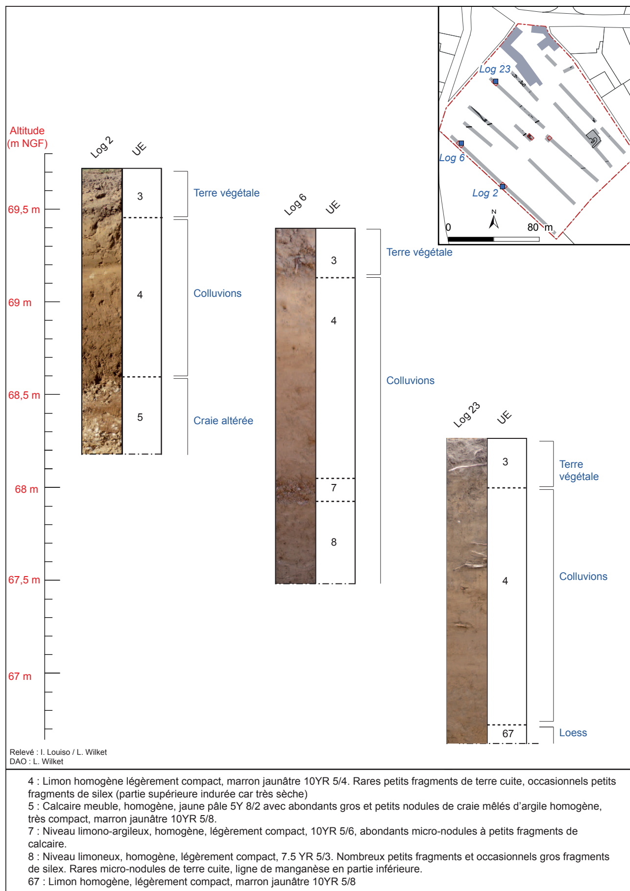
Fig. 6 : Duisans, Rue du Château, les observations géologiques in situ , L. Wilket - DA, CD 62.
