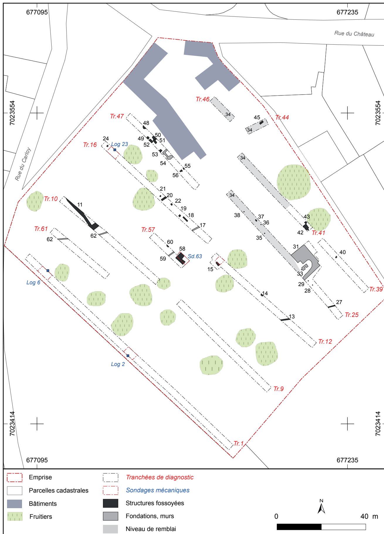
Fig. 9 : Duisans, Rue du Château, plan général, L. Wilket - DA, CD 62
