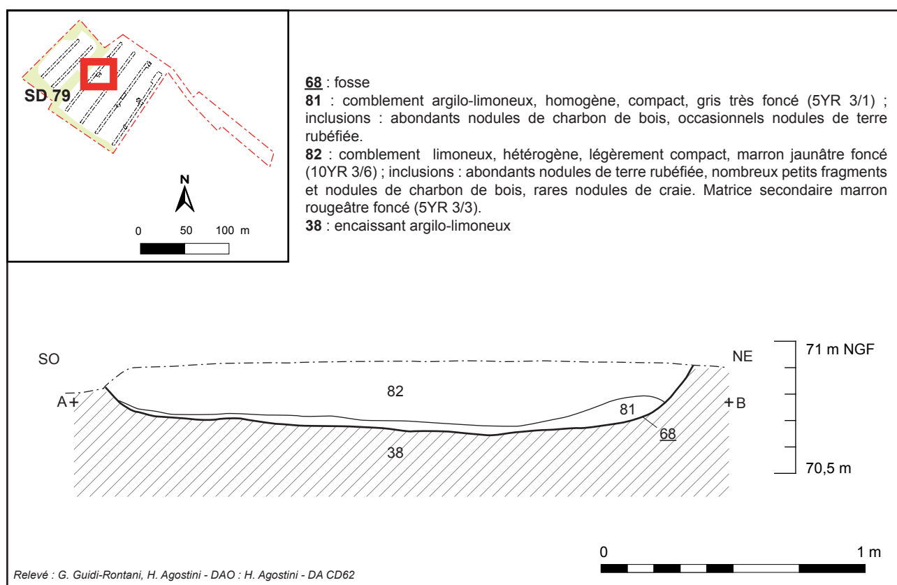
Fig. 22 : Dury, Rue des Hallots, coupe de la fosse 68, G. Guidi-Rontani - DA, CD 62
