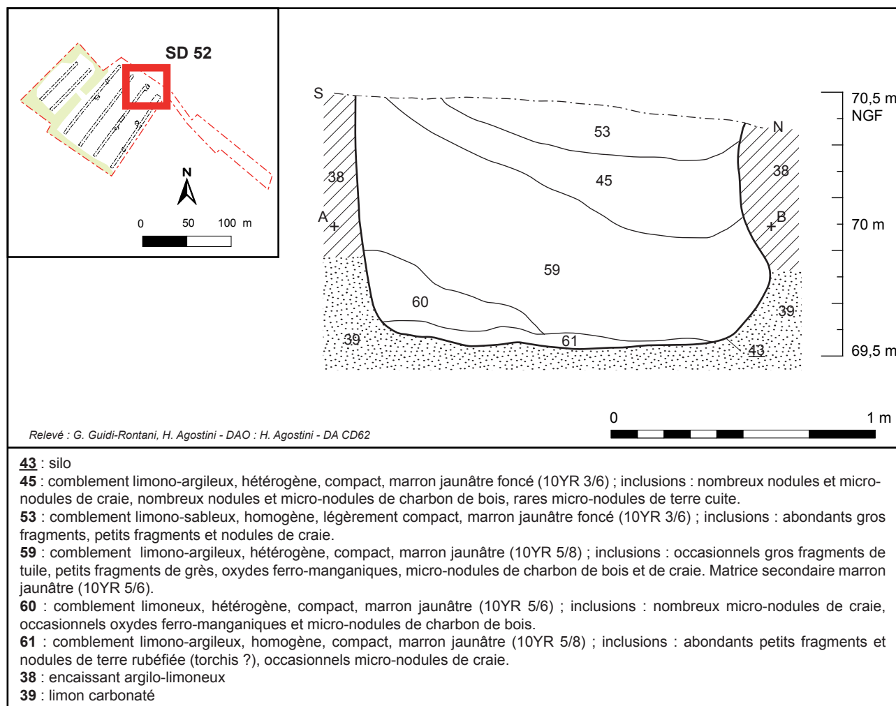
Fig. 12 : Dury, Rue des Hallots, relevé de coupe de la fosse 43, H. Agostini - DA, CD 62
