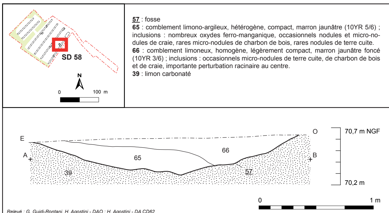
Fig. 14 : Dury, Rue des Hallots, relevé de coupe de la fosse 57, H. Agostini - DA, CD 62
