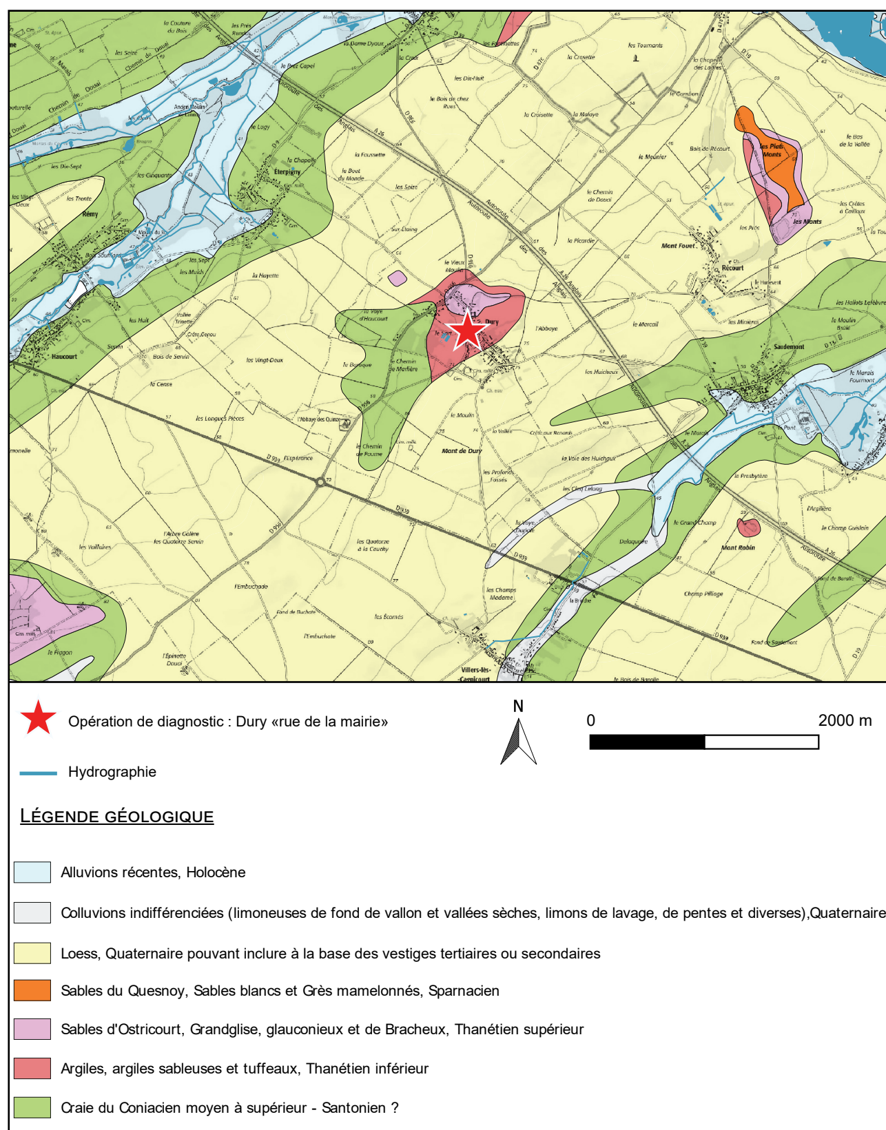
Fig. 6 : Dury, rue de la Mairie, localisation de l'opération dans le contexte géologique local (extrait de la carte géologique au 1/50 000 harmonisée (Lacquement et al. 2004 ; BRGM-Infoterre 2019), A Beauchamp - DA, CD 62.
