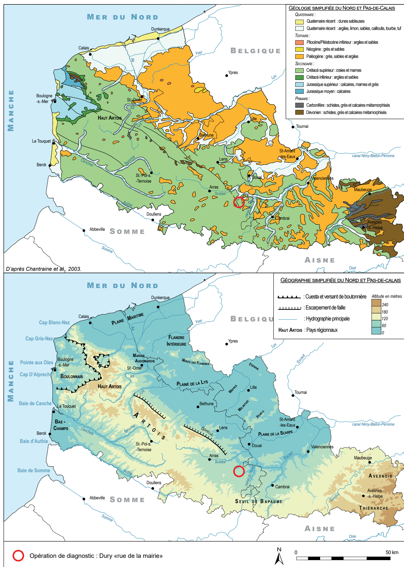
Fig. 5 : Dury, rue de la Mairie, localisation de l'opération dans le contexte géologique et géographique régional, A Beauchamp - DA, CD 62.
