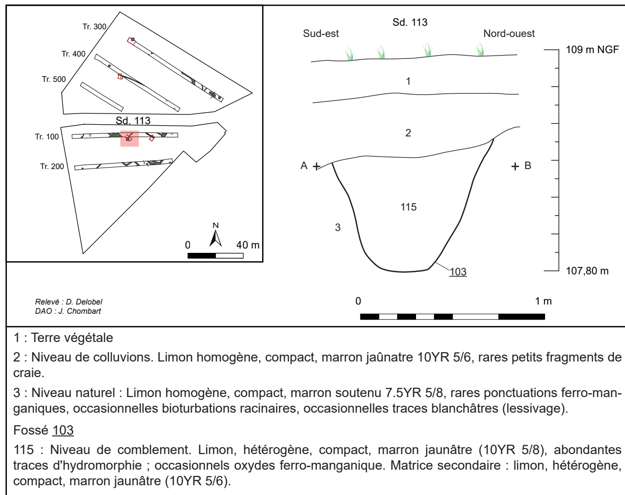
Fig. 14 : Ervillers, rue de l'Église, coupe du fossé 103 au 1/20 e , J. Chombart - DA, CD 62.
