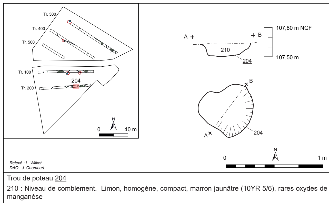
Fig. 20 : Ervillers, rue de l'Église, coupe et plan du trou de poteau 204 au 1/20 e , J. Chombart - DA, CD 62.
