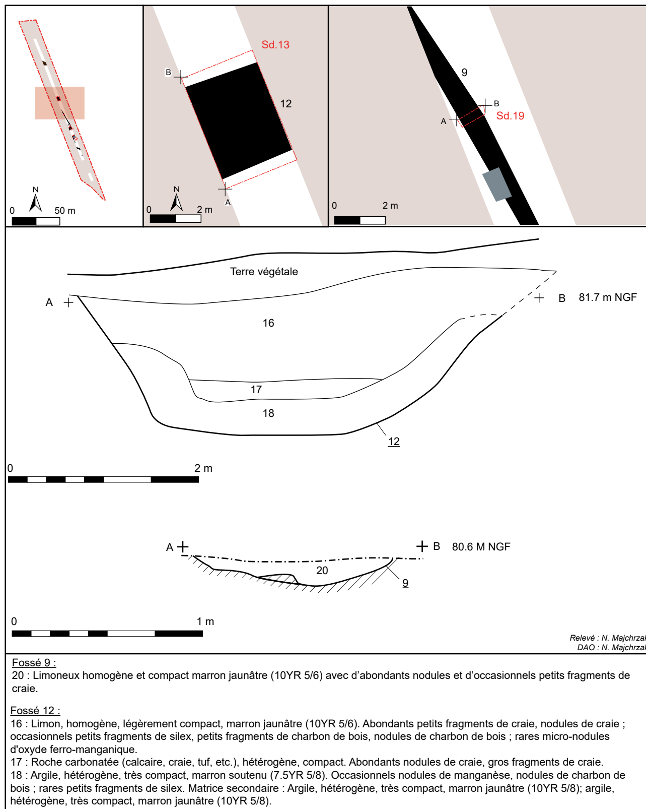
Fig. 15 : Étrun, 18 rue du Mont César, coupes des fossés 9 et 12, N. Majchrzak - DA 62.
