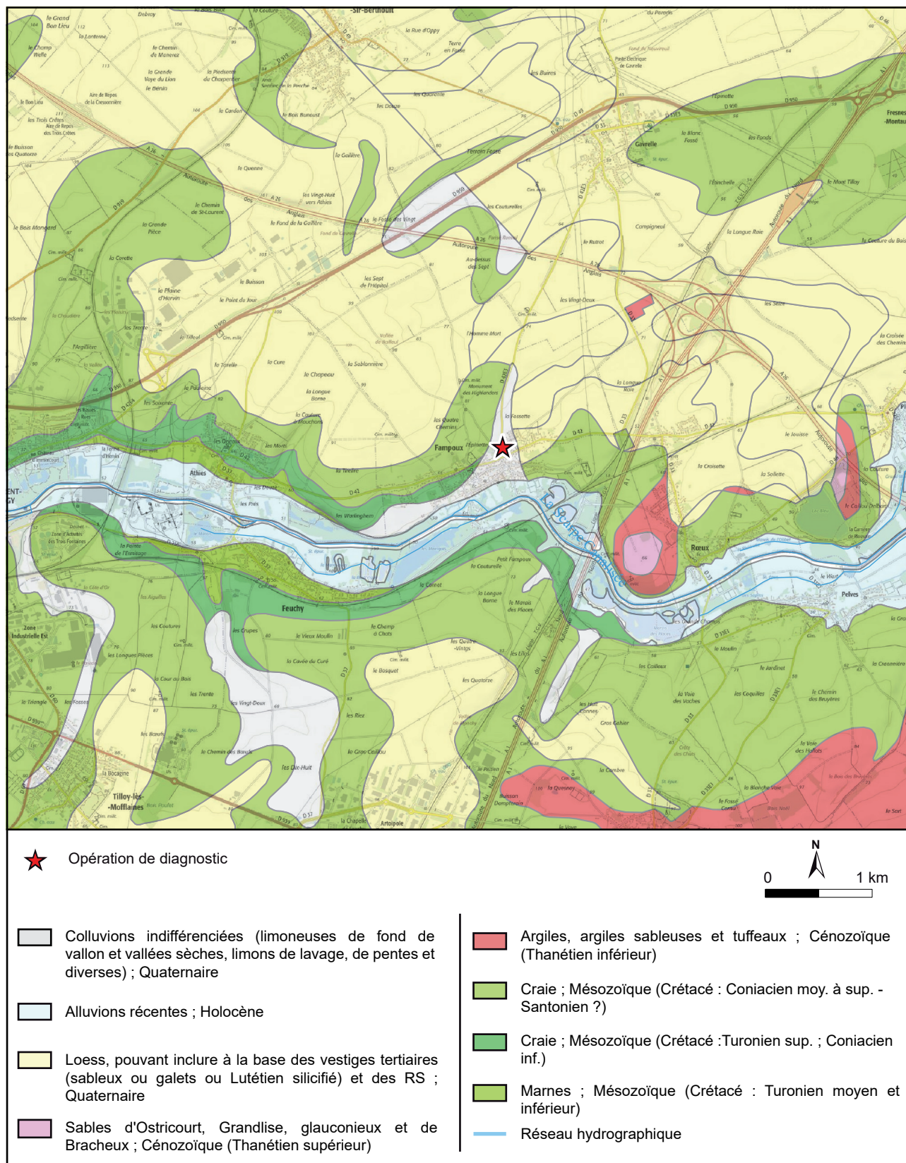
Fig. 6 : Fampoux, Rue des Étangs, extrait de la carte géologique au 1/50 000 harmonisée (Lacquement et al. 2004 ; BRGM-Infoterre 2020), M. Meurisse-Fort - DA, CD 62.
