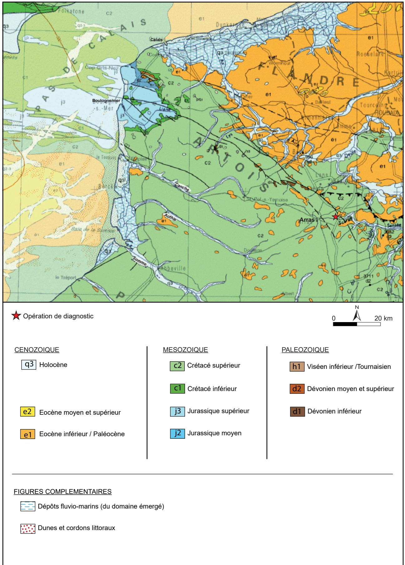
Fig. 5 : Fampoux, Rue des Étangs, extrait de la carte géologique au millionième (Chantraine et al. 1996 ; BRGM-Infoterre 2020), M. Meurisse-Fort - DA, CD 62.
