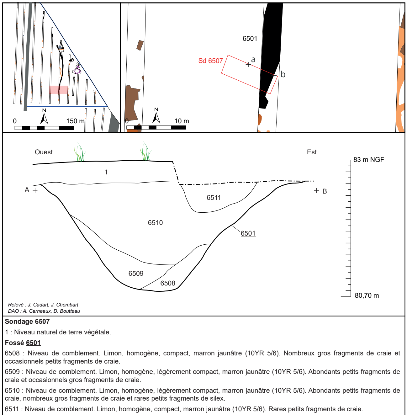
Fig. 126 : Feuchy, Saint-Laurent-Blangy, Tilloy-lès-Mofflaines, Extension de la ZI Est, relevé de coupe du fossé 6501, sondage 6507, dessin J. Cadart et J. Chombart / DAO A. Carneaux et D. Bouteau - DA, CD 62.
