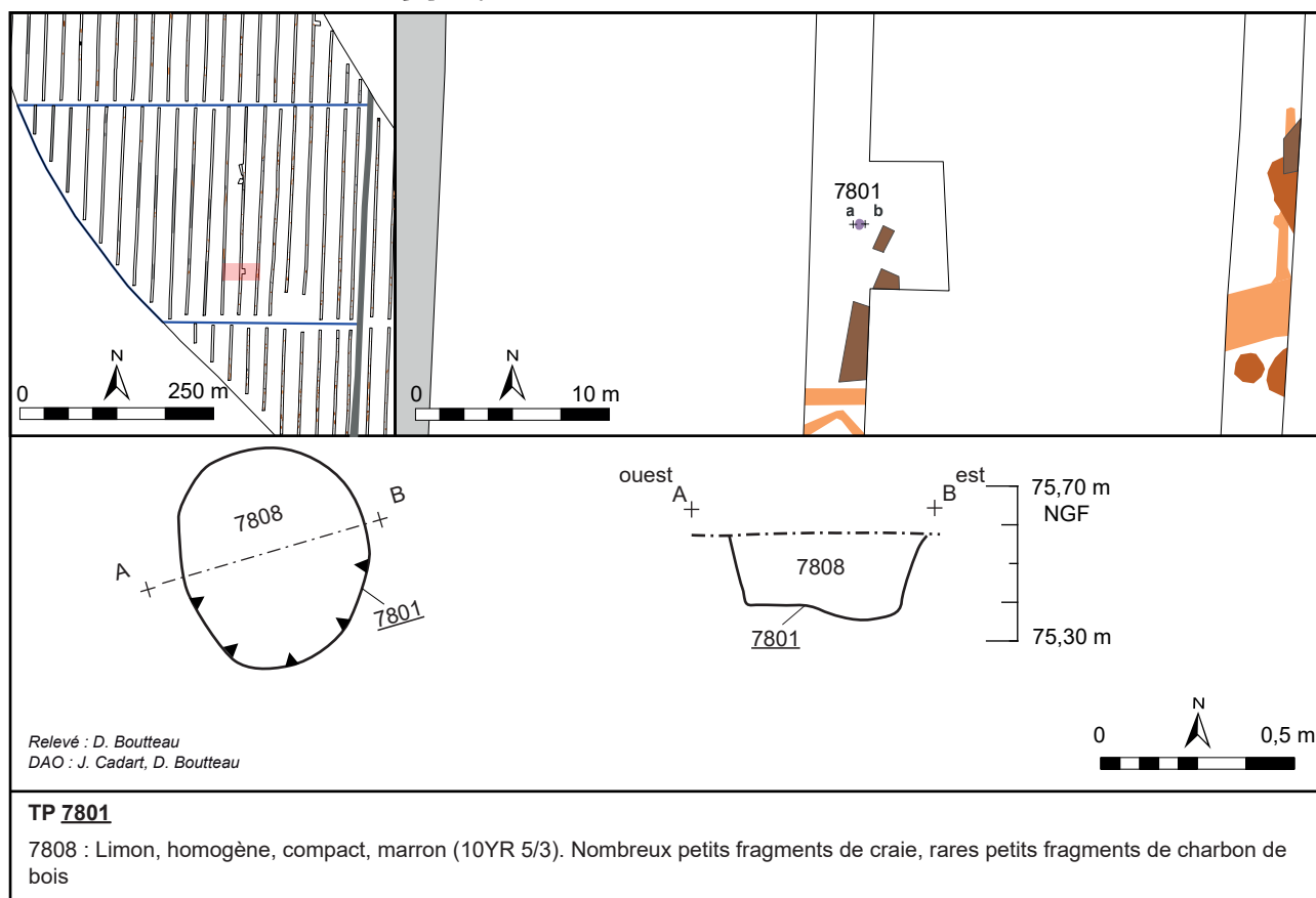
Fig. 144 : Feuchy, Saint-Laurent-Blangy, Tilloy-lès-Mofflaines, Extension de la ZI Est, coupe du trou de poteau 7801, dessin D. Boutteau / DAO J. Cadart et D. Boutteau - DA, CD 62.
