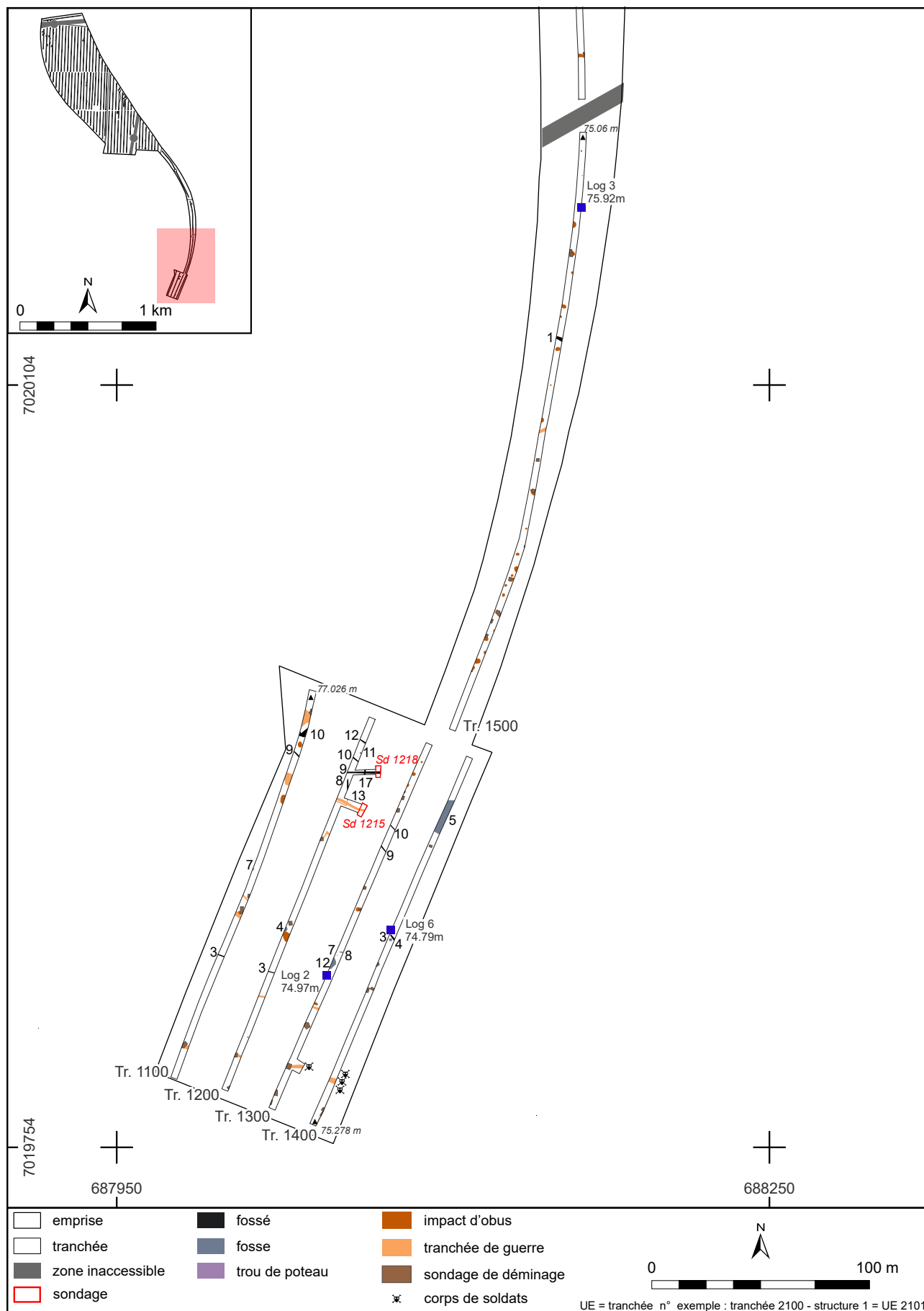
Fig. 22 : Feuchy, Saint-Laurent-Blangy, Tilloy-lès-Mofflaines, Extension de la ZI Est, plan de la zone 1 au 1/2 500°, C. Costeux - DA, CD 62.
