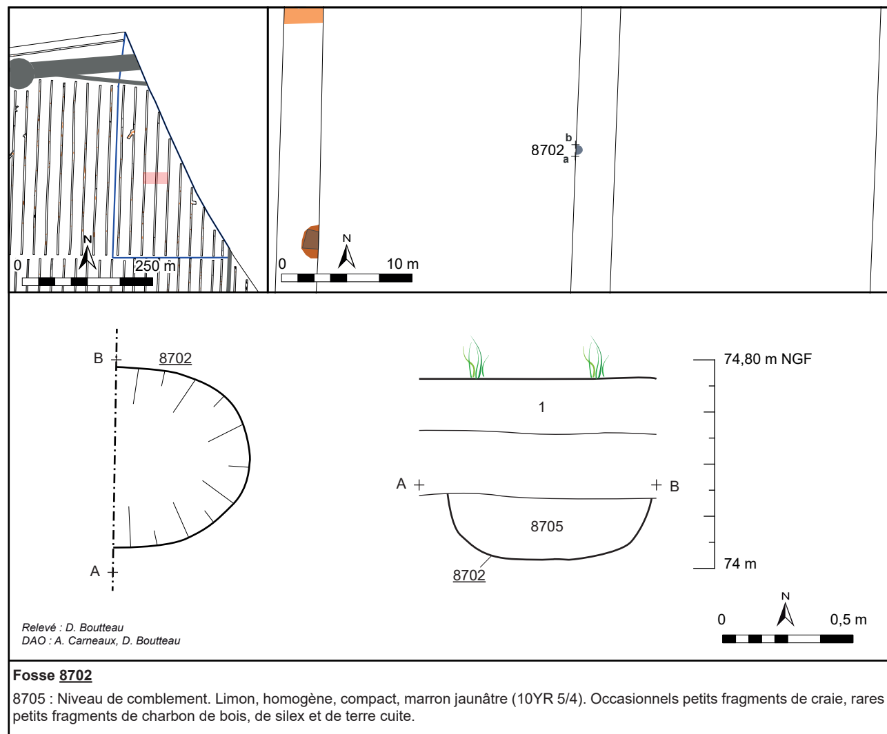
Fig. 156 : Feuchy, Saint-Laurent-Blangy, Tilloy-lès-Mofflaines, Extension de la ZI Est, plan et coupe de la fosse 8302, dessin D. Boutteau / DAO A. Carneaux et D. Boutteau - DA, CD 62.
