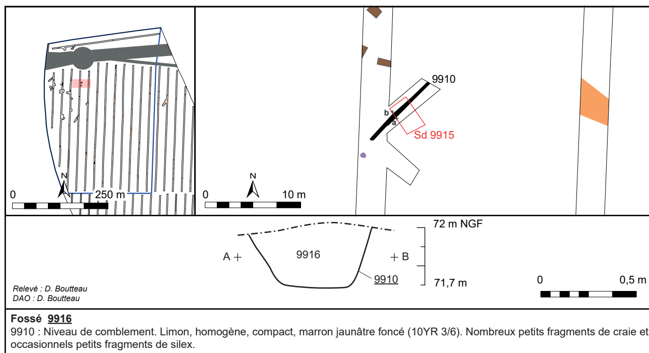
Fig. 206 : Feuchy, Saint-Laurent-Blangy, Tilloy-lès-Mofflaines, Extension de la ZI Est, coupe du fossé 9910, dessin et DAO D. Boutteau - DA, CD 62.
