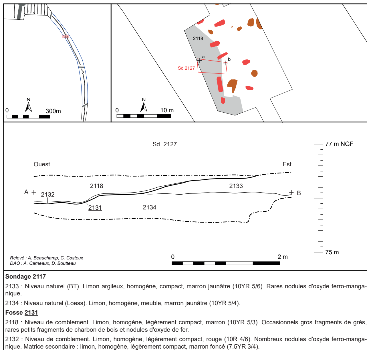
Fig. 42 : Feuchy, Saint-Laurent-Blangy, Tilloy-lès-Mofflaines, Extension de la ZI Est, coupe de la fosse 2131, dessin C. Costeux et A. Beauchamp / DAO A. Carneaux et D. Boutteau - DA, CD 62.
