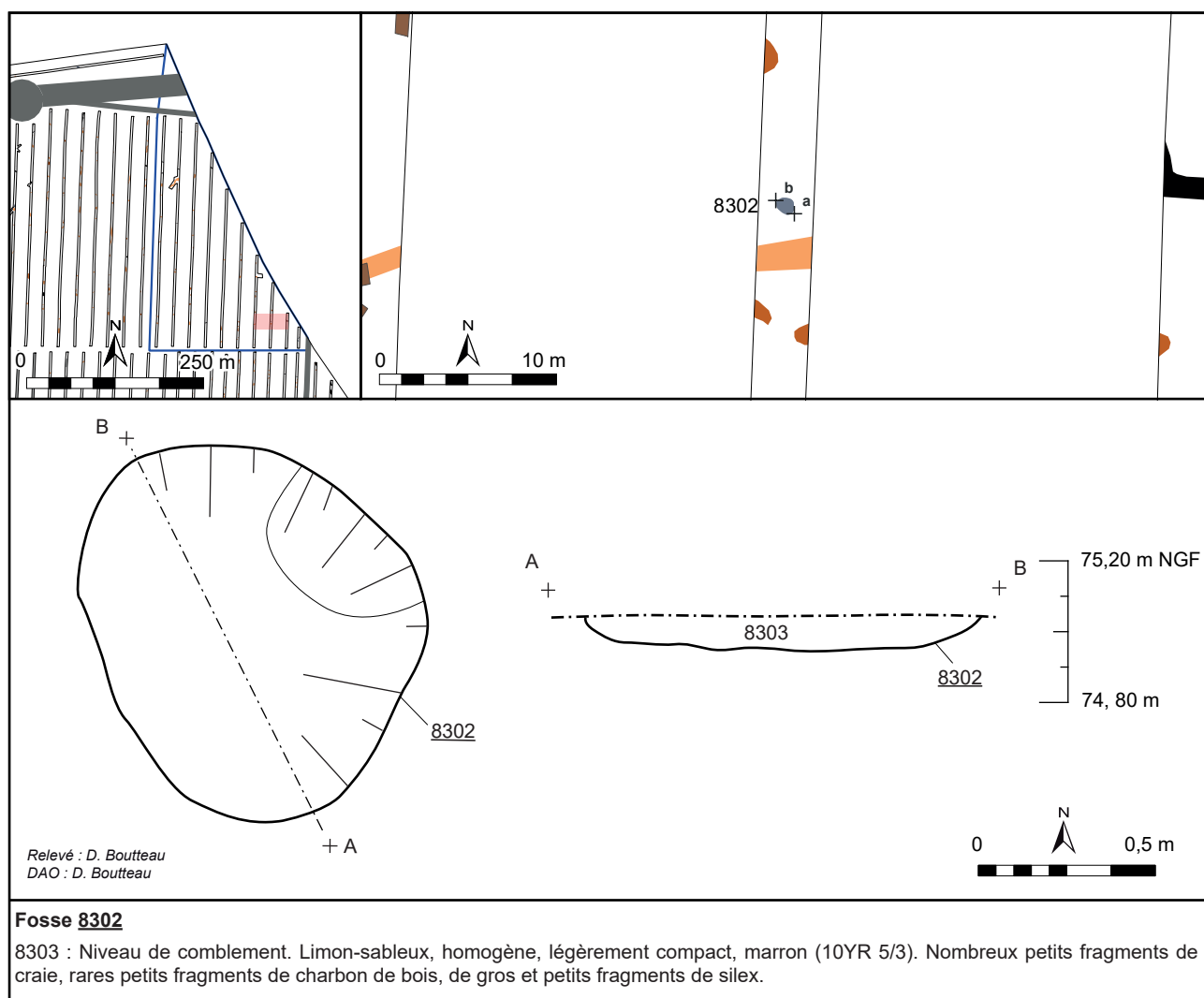
Fig. 153 : Feuchy, Saint-Laurent-Blangy, Tilloy-lès-Mofflaines, Extension de la ZI Est, plan et coupe de la fosse 8302, dessin et DAO D. Boutteau - DA, CD 62.
