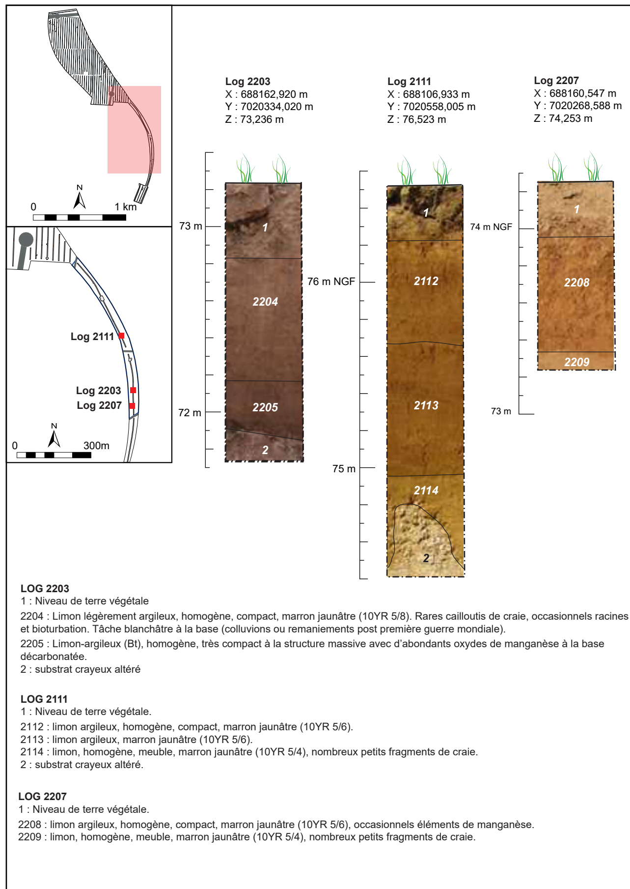
Fig. 40 : Feuchy, Saint-Laurent-Blangy, Tilloy-lès-Mofflaines, Extension de la ZI Est, logs stratigraphiques réalisés en zone 2, A. Beauchamp - DA, CD 62.
