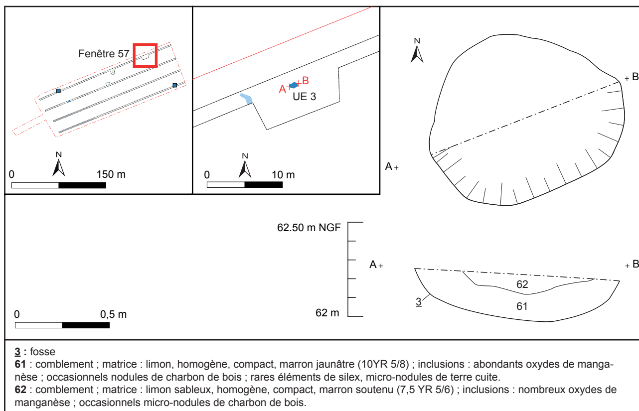
Fig. 12 : Givenchy-en-Gohelle, rue Degreaux - rue des Petits Champs, coupe et plan de la fosse 3 datée du Néolithique moyen II, dessin/DAO C. Costeux - DA, CD 62.
