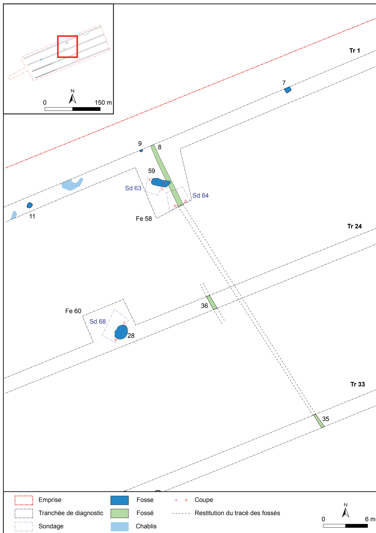
Fig. 16 : Givenchy-en-Gohelle, rue Degreaux - rue des Petits Champs, plan de détail des fenêtres 58 et 60, C. Costeux - DA, CD 62.
