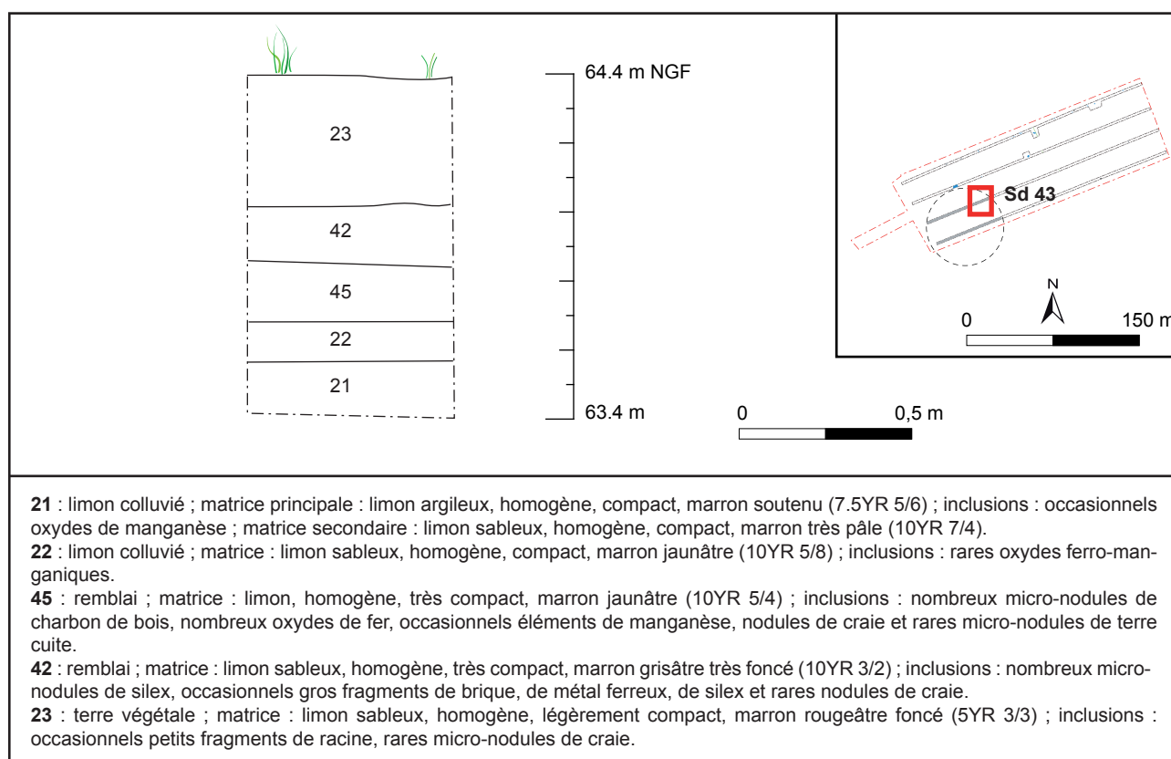
Fig. 20 : Givenchy-en-Gohelle, rue Degreaux - rue des Petits Champs, sondage de type log dans les remblais de la cuvette, dessin/DAO C. Costeux - DA, CD 62.
