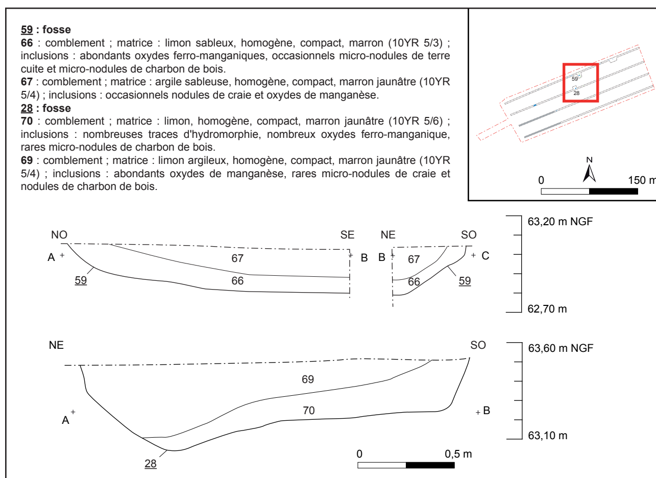
Fig. 17 : Givenchy-en-Gohelle, rue Degreaux - rue des Petits Champs, coupes des fosses 28 et 59, dessin/DAO C. Costeux - DA, CD 62.
