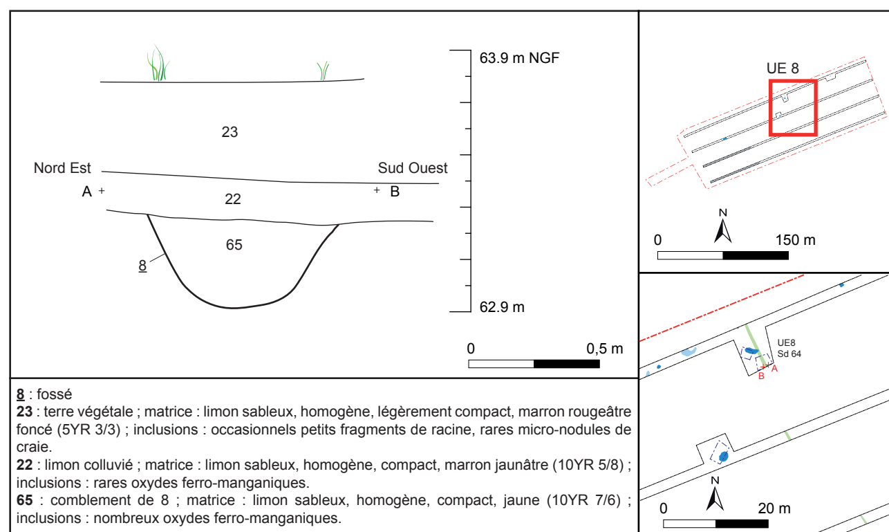
Fig. 18 : Givenchy-en-Gohelle, rue Degreaux - rue des Petits Champs, coupe du fossé 8, dessin/DAO C. Costeux - DA, CD 62.
