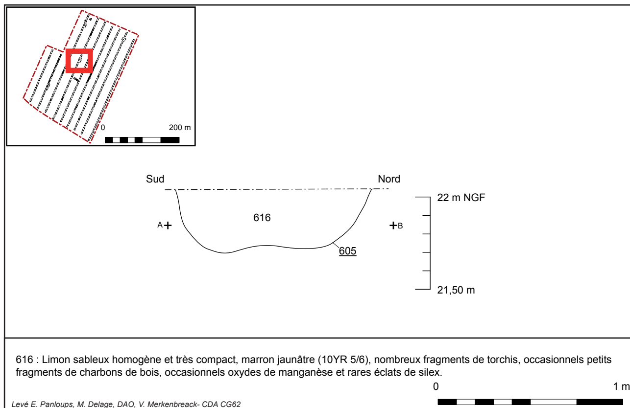
Fig. 29 : Guînes, RD 231, la Rue d'Ardres, coupe de la fosse 605, E. Panlouis, M. Delage - CDA-CG62.
