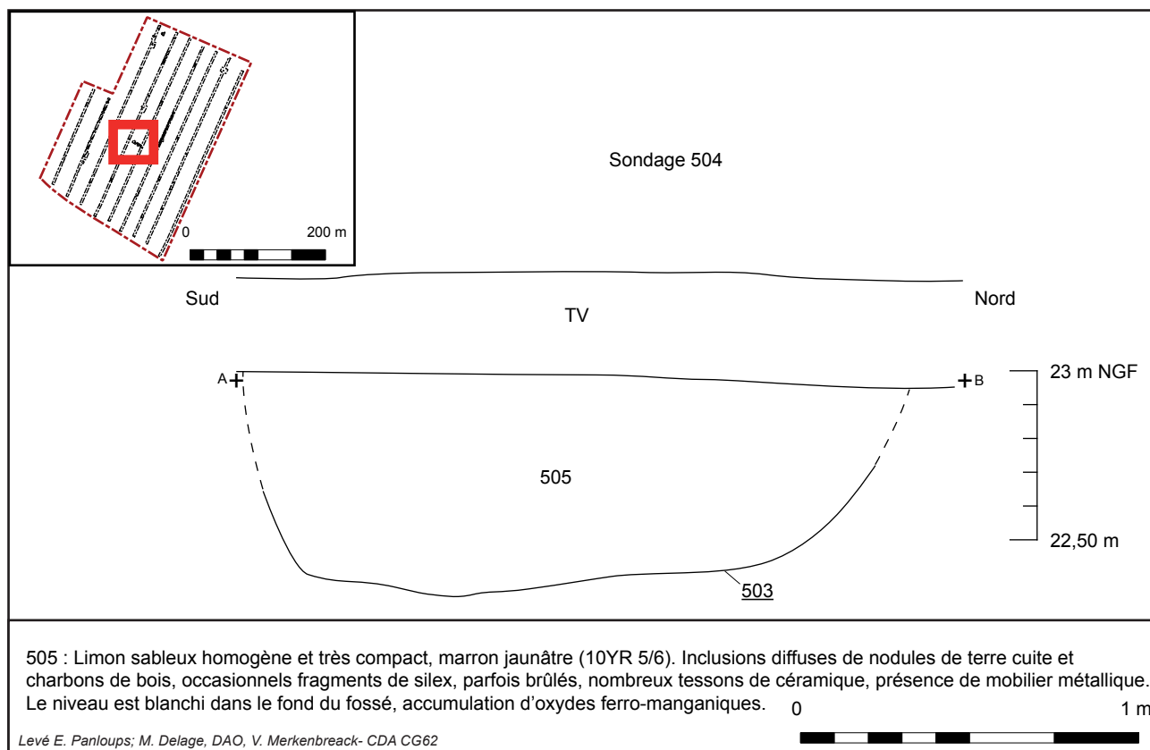
Fig. 28 : Guînes, RD 231, la Rue d'Ardres, coupe du fossé d'enclos 503, E. Panlouis, M. Delage - CDA-CG62.
