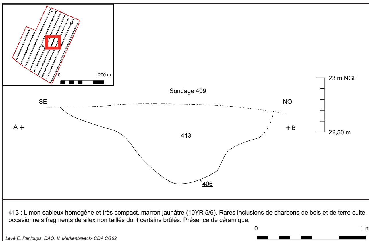
Fig. 23 : Guînes, RD 231, la Rue d'Ardres, coupe du fossé d'enclos 406, E. Panloup - CDA-CG62.
