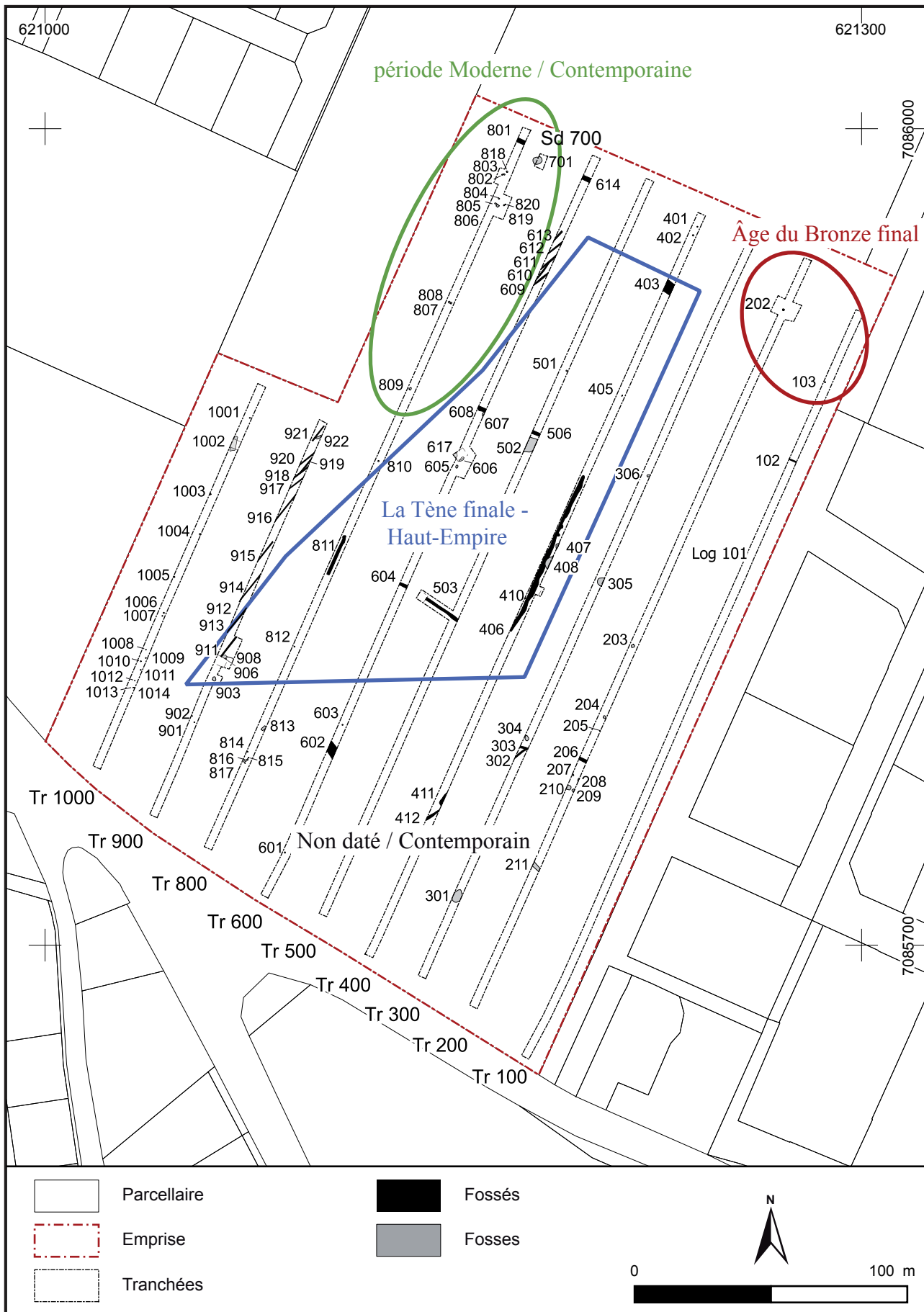
Fig. 10 : Guînes, RD 231, la Rue d'Ardres, emprise du diagnostic avec localisation des vestiges par périodes chronologiques, V. Merkenbreack - CDA-CG62 .
