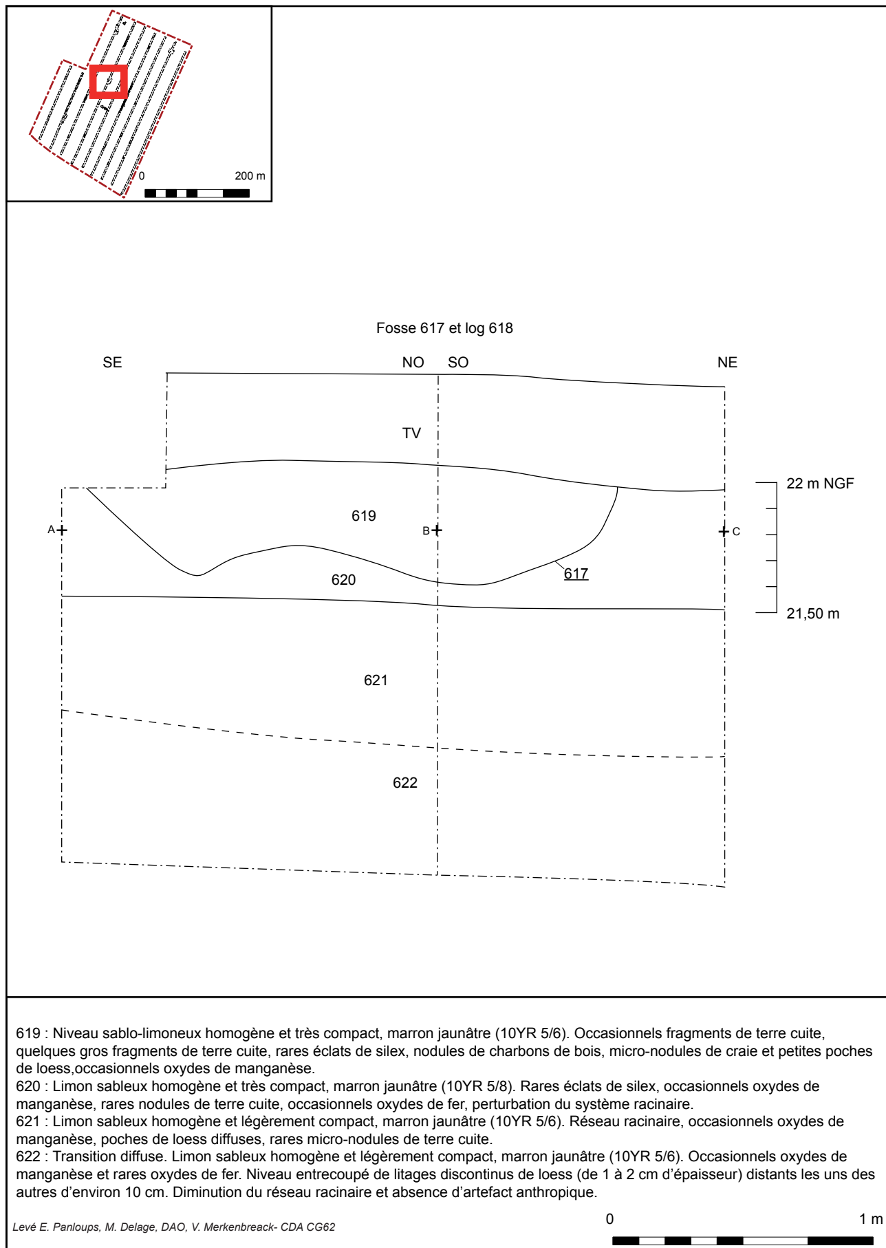
Fig. 32 : Guînes, RD 231, la Rue d'Ardres, coupe de la fosse 617, E. Panlouis, M. Delage - CDA-CG62.
