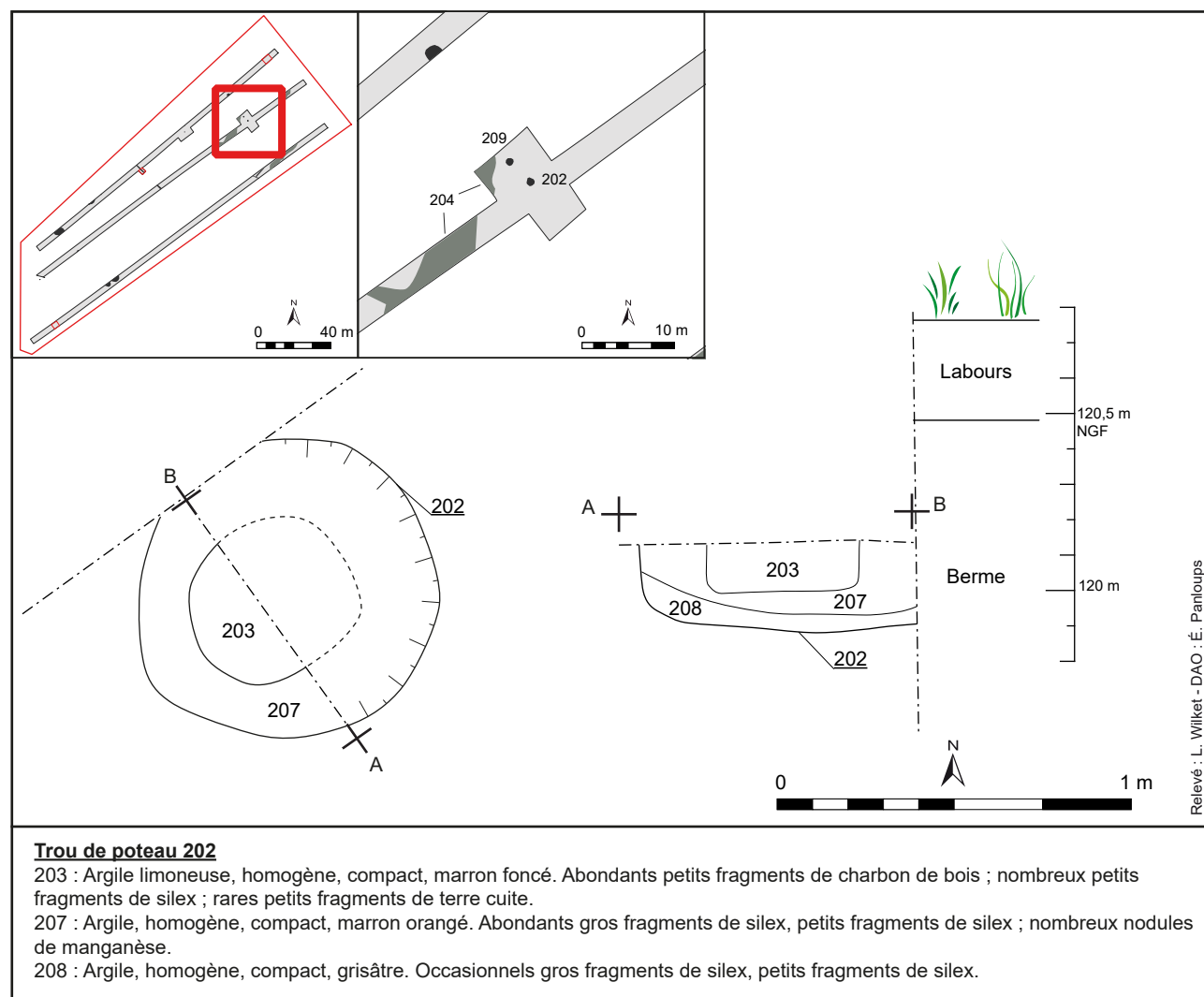
Fig. 23 : Hallines, Les Campagnes, plan et coupe du trou de poteau 202, relevé L. Wilket / DAO É. Panloup - DA, CD 62.
