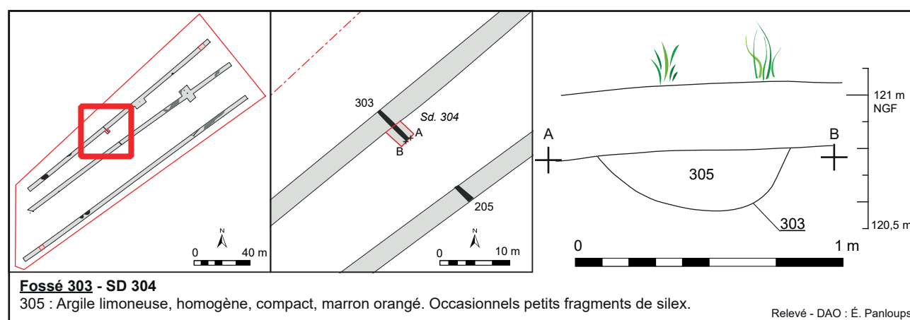
Fig. 19 : Hallines, Les Campagnes, coupe du fossé 303, relevé / DAO É. Panlouis - DA, CD 62.
