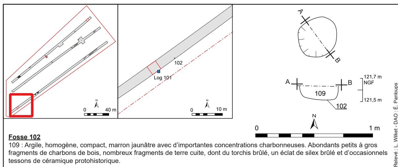
Fig. 14 : Hallines, Les Campagnes, plan et coupe de la fosse 102, relevé L. Wilket / DAO É. Panlouis - DA, CD 62.
