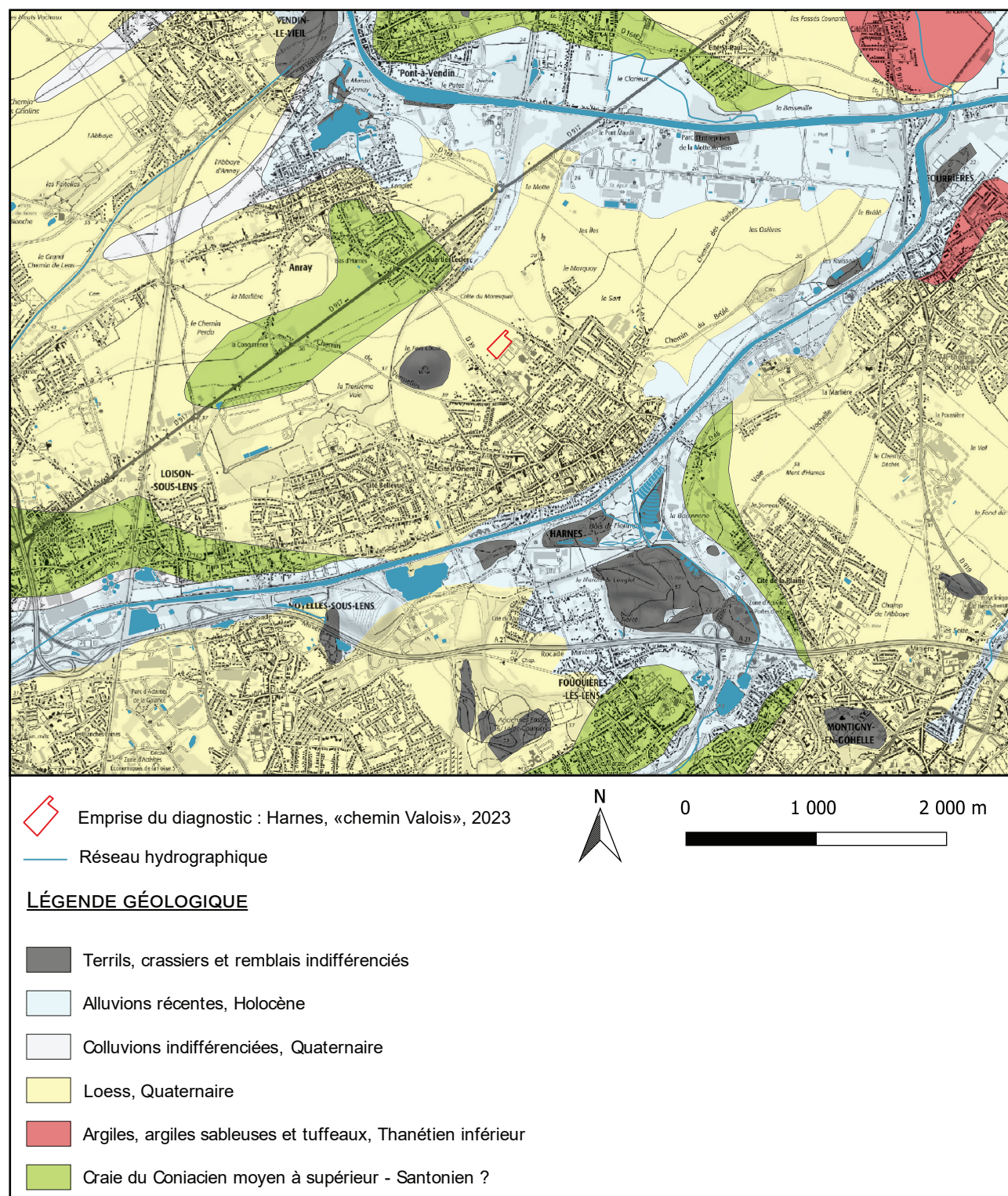
Fig. 7 : Harnes, 128 chemin Valois, extrait de la carte géologique au 1/50 000e harmonisée (BRGM-Infoterre 2023, Lacquement et al. 2004), A. Beauchamp - DA, CD 62.
