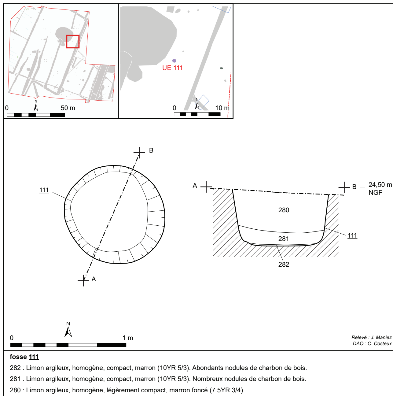
Fig. 25 : relevé de la fosse 111, C. Costeux - DA, CD 62.
