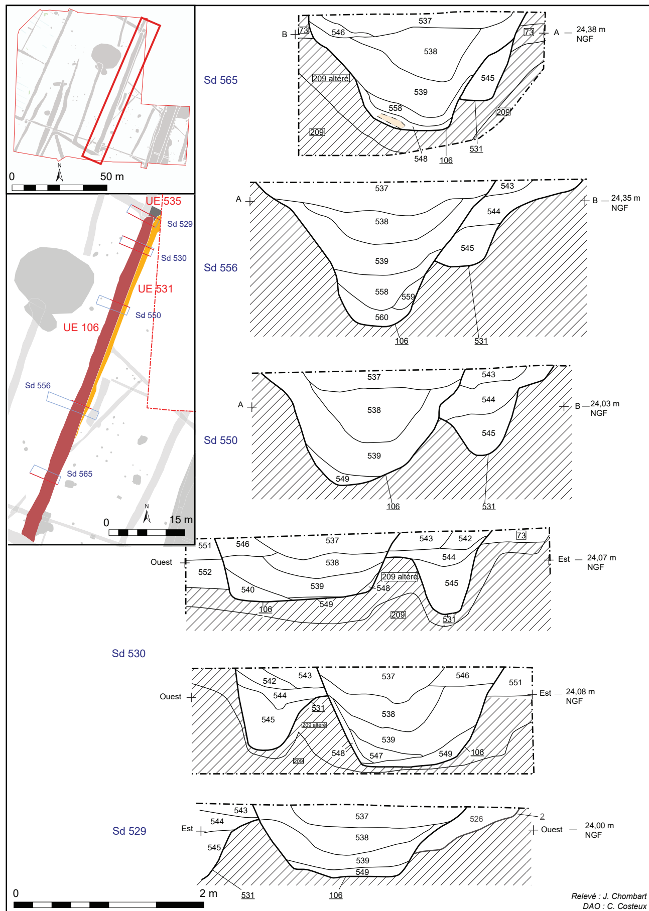
Fig. 76 : coupes du fossé 106, C. Costeux - DA, CD 62.
