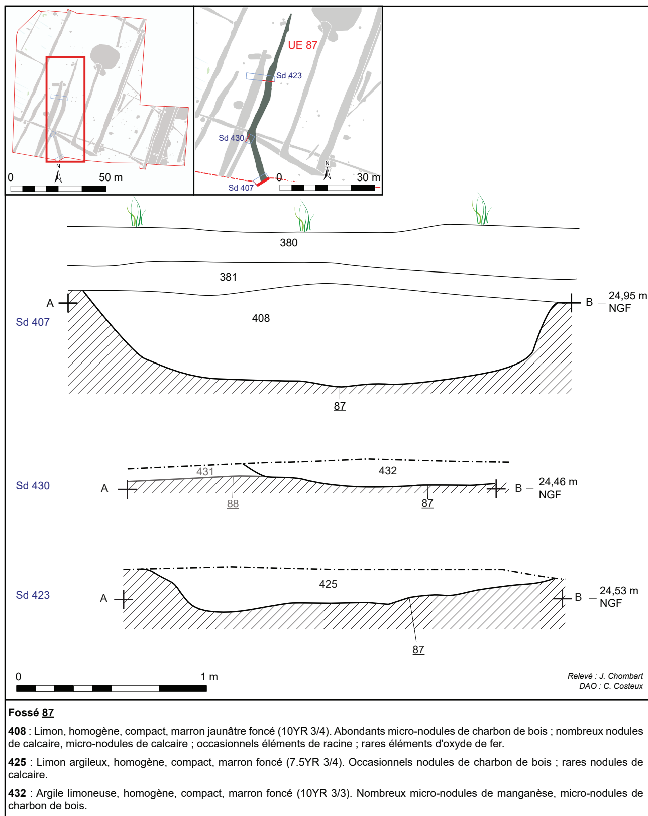
Fig. 108 : coupes du fossé 87, C. Costeux - DA, CD 62.
