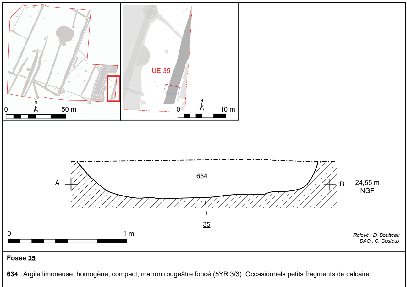
Fig. 111 : coupe du fossé 35 dans le sondage 633, C. Costeux - DA, CD 62.
