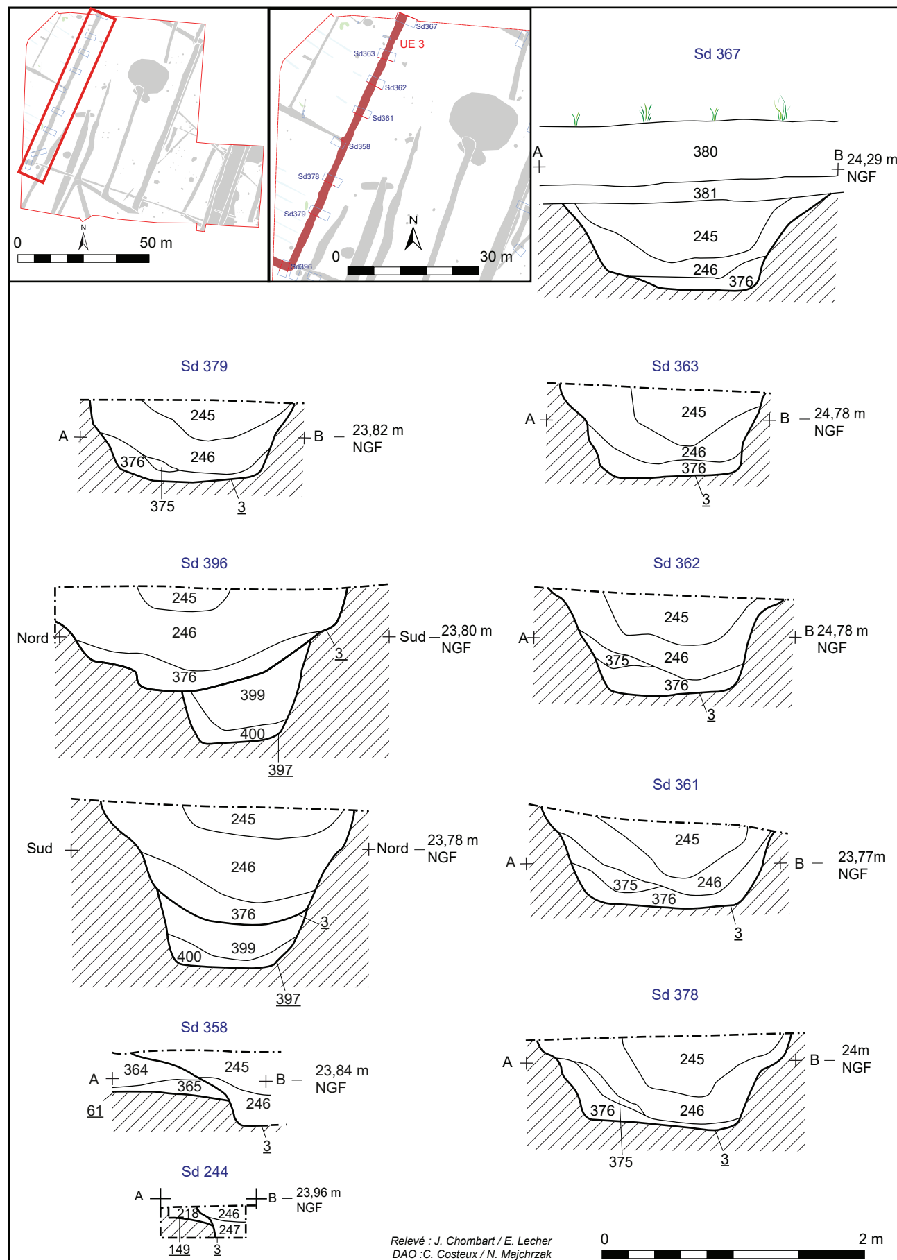
Fig. 72 : coupes du fossé 3, C. Costeux - DA, CD 62.
