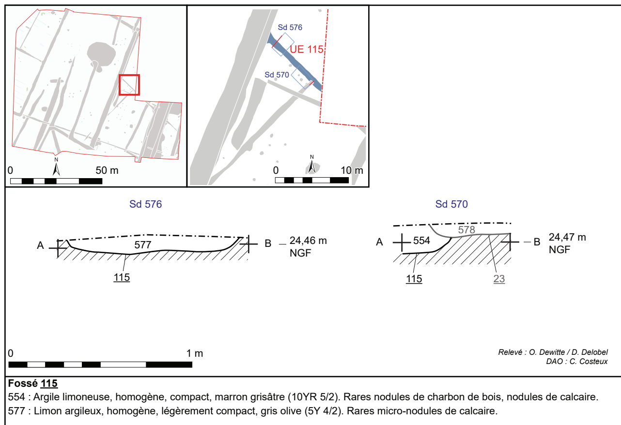
Fig. 50 : coupes du fossé 115, C. Costeux - DA, CD 62.
