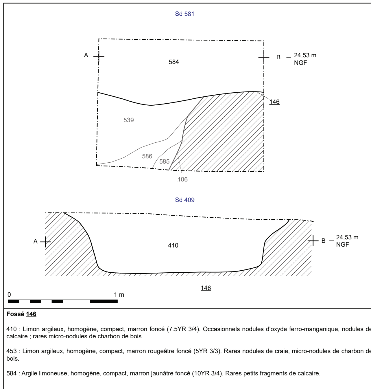
Fig. 84 : coupes du fossé 146, C. Costeux - DA, CD 62.
