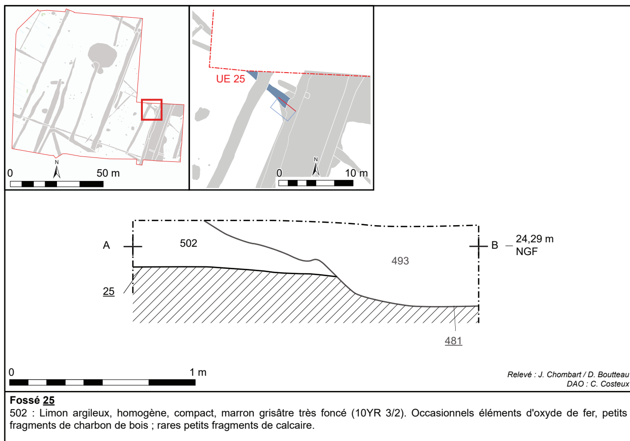
Fig. 48 : coupe longitudinale du fossé 25, cliché J. Chombart - DA, CD 62.
