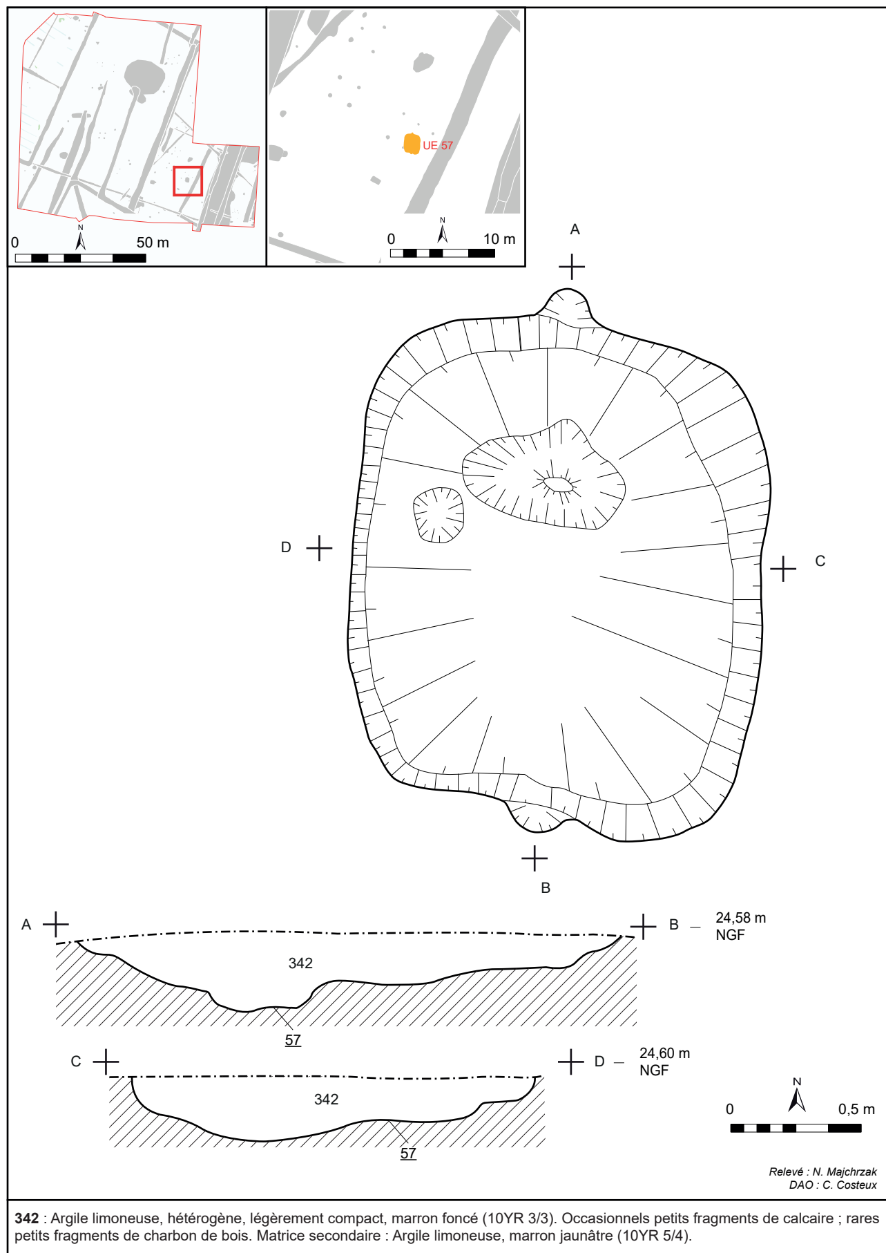
Fig. 94 : plan et coupe de la fosse 57, C. Costeux - DA, CD 62.
