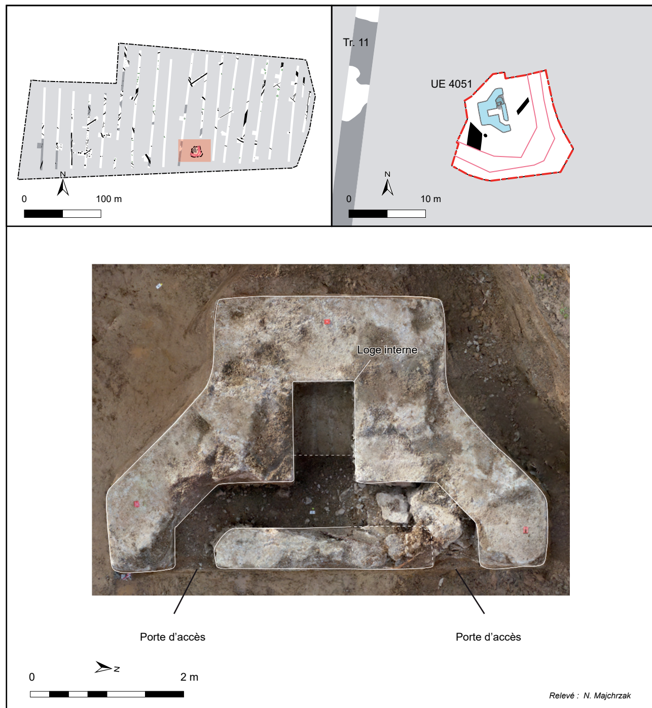
Fig. 44 : Harnes, ZAC de la Motte du Bois, vue du dessus du bunker 4051 sur la zone du lot 4, L. Wilket - DA, CD 62.
