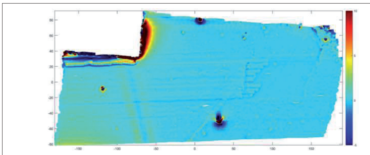
Fig. 8 : Harnes, ZAC de la Motte du Bois, Carte d'intensité des anomalies magnétiques sur le lot 4, Entreprise CARDEM .
