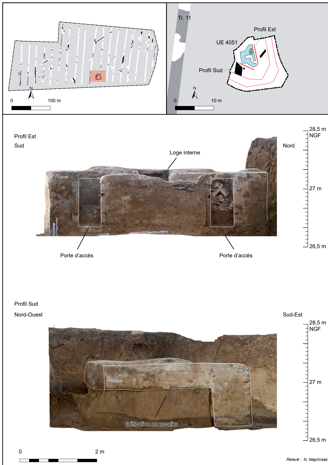
Fig. 45 : Harnes, ZAC de la Motte du Bois, vue de profil du bunker 4051 sur la zone du lot 4, L. Wilket - DA, CD 62.
