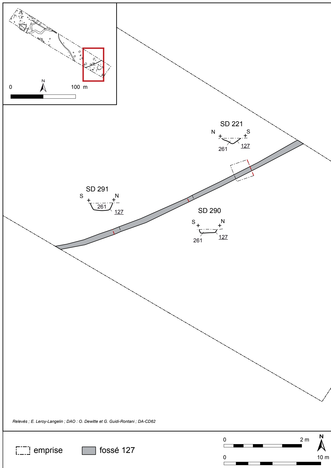
Fig. 110 : Haute-Avesnes, Les Tourtelottes, plan et coupes du fossé 127, O. Dewitte, G. Guidi Rontani - DA CD62.
