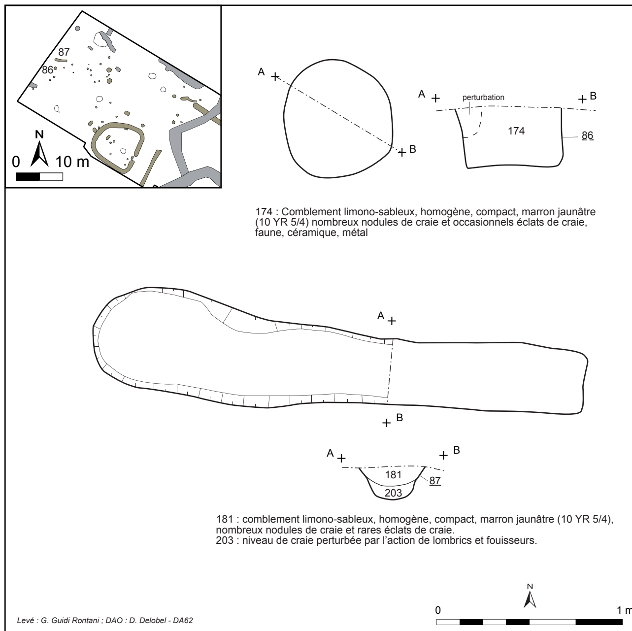
Fig. 50 : Haute-Avesnes, Les Tourtelottes, plans et coupes des structures 86 et 87, G. Guidi-Rontani, D. Delobel - DA CD62.
