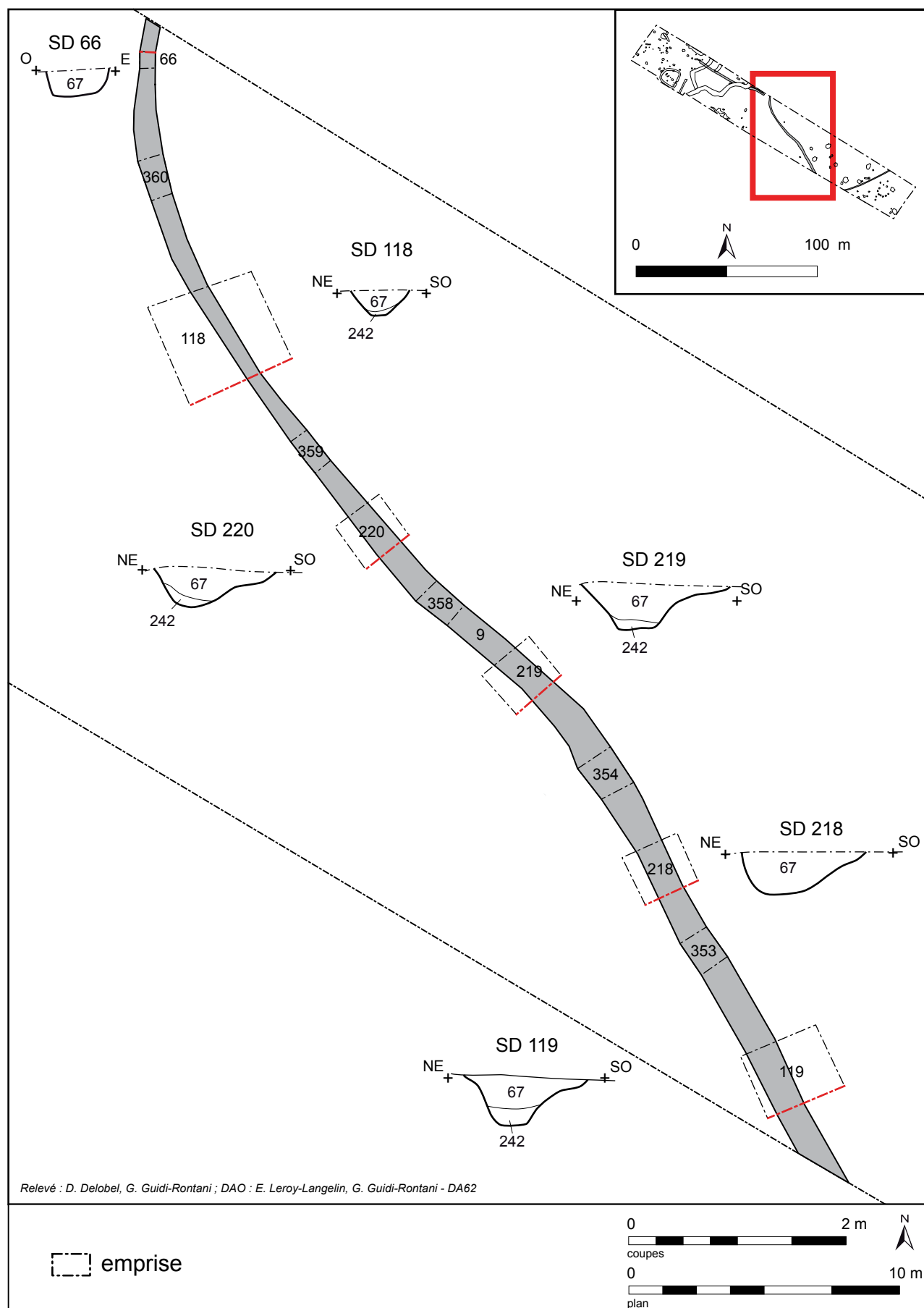
Fig. 104 : Haute-Avesnes, Les Tourtelottes, plan et coupes du fossé 9, E. Leroy Langelin, G. Guidi-Rontani - DA CD62.
