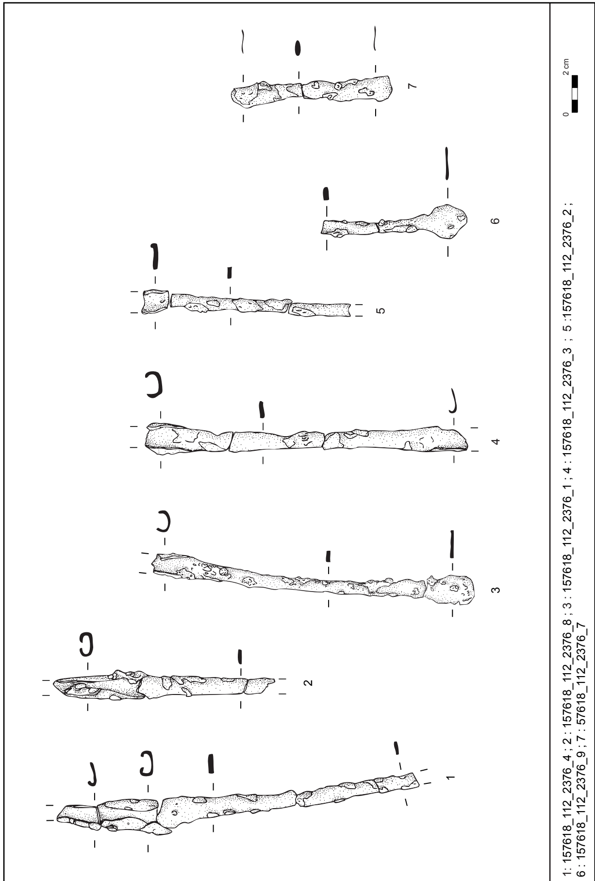
Fig. 68 : Haute-Avesnes, Les Tourtelottes, barres à douille conique en fer , dessins L. Dalmau - DA CD 62.
