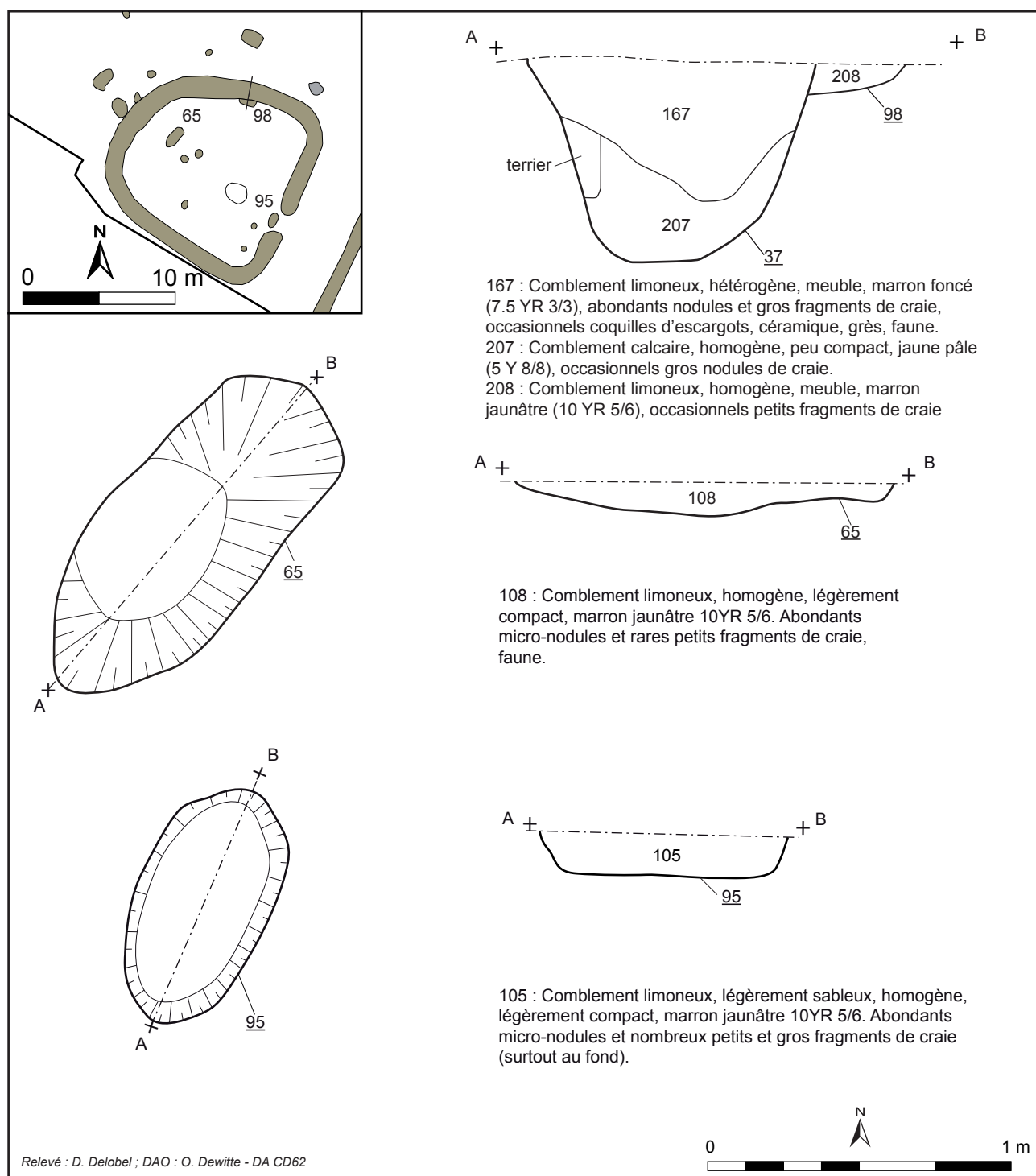
Fig. 120 : Haute-Avesnes, Les Tourtelottes, plan et coupes des structures 65, 95, 98, D. Delobel, O. Dewitte - DA CD62.
