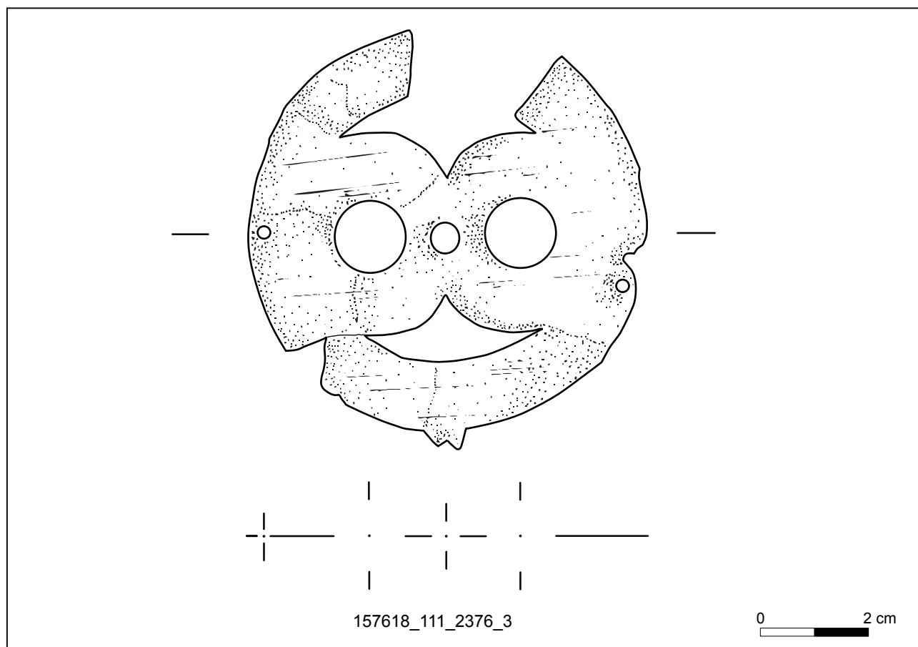
Fig. 80 : Haute-Avesnes, Les Tourtelottes, dessin de la plaque décorative en alliage cuivreux (157618_111_2376_3), dessin L. Dalmau - DA CD62.
