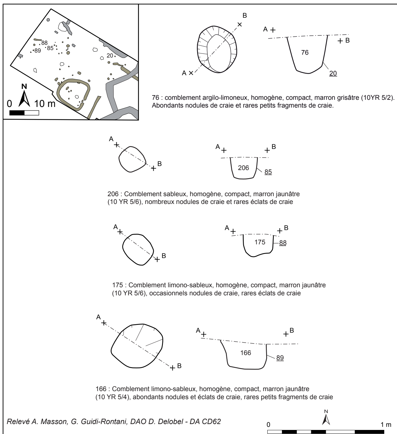
Fig. 118 : Haute-Avesnes, Les Tourtelottes, plan et coupes des structures 20, 85, 88 et 89, A. Masson, G. Guidi Rontani, D. Delobel - DA CD62.
