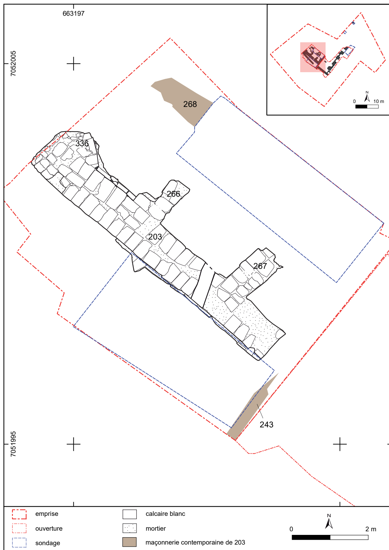
Fig. 44 : Lillers, place de l'Église, plan de la fondation 203 dans son environnement, relevé photogrammétrique O. Dewitte, DAO M. Haddad - DA, CD 62.
