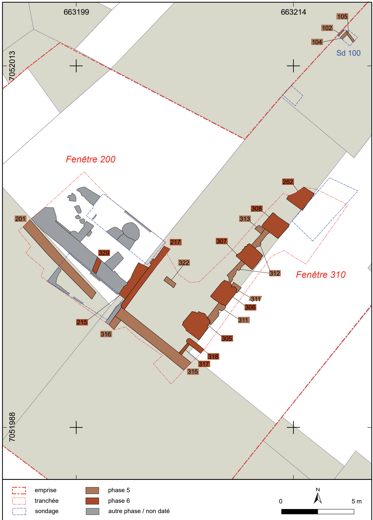
Fig. 65 : Lillers, place de l'Église, plan général des vestiges des phases 5 et 6 sur fond de plan tiré du cadastre contemporain avant les démolitions de 2018, O. Dewitte - DA, CD 62.
