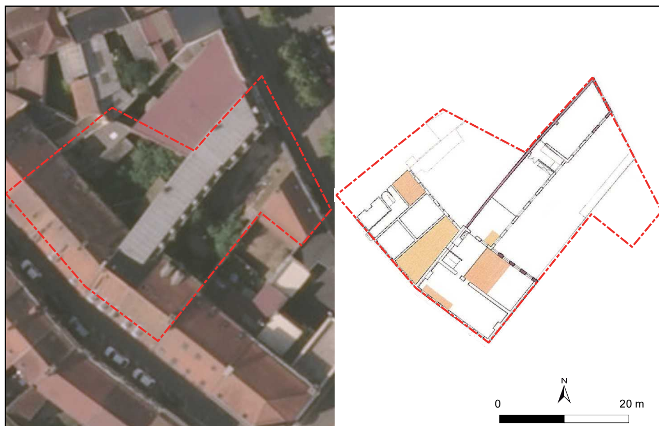
Fig. 14 : Lillers, place de l'Église, emprise du diagnostic, sur l'orthophotographie du Nord-Pas-de-Calais de 2015, et emprise du diagnostic sur le plan de l'école établi par EURL Angez, Cabinet d'architecte, O. Dewitte - DA, CD 62
