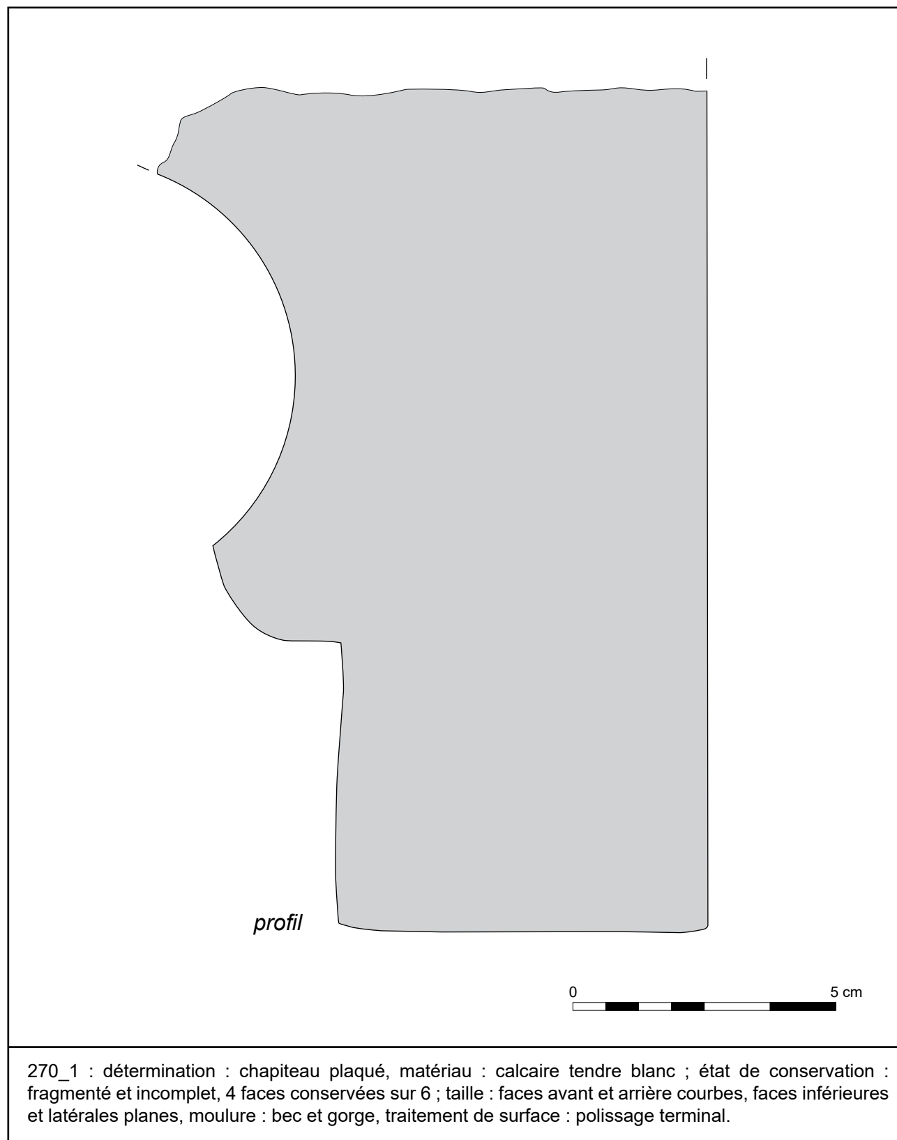
Fig. 42 : Lillers, place de l'Église, chapiteau issu du niveau de démolition 270, dessin/DAO H. Agostini - DA, CD 62.
