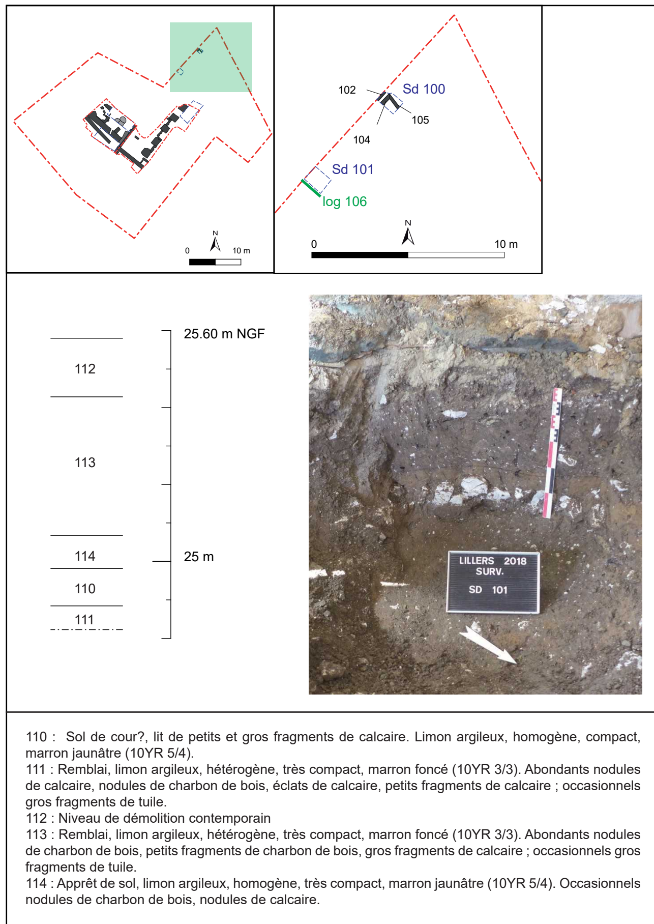
Fig. 63 : Lillers, place de l'Église, log stratigraphique dans le sondage 101, relevé/DAO J.-M. Willot - DA, CD 62.
