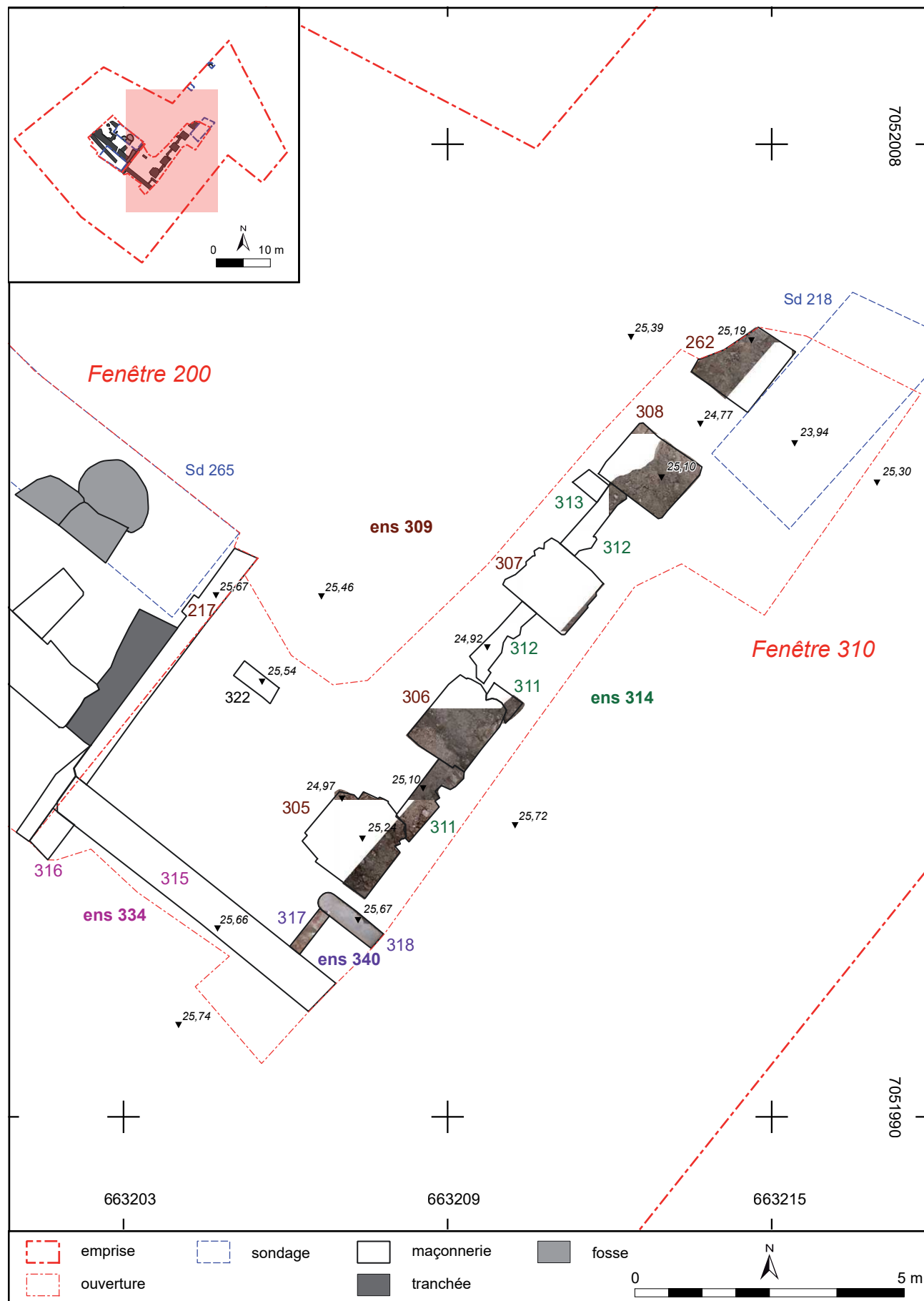
Fig. 46 : Lillers, place de l'Église, plan de la fenêtre 310, O. Dewitte - DA, CD 62.
