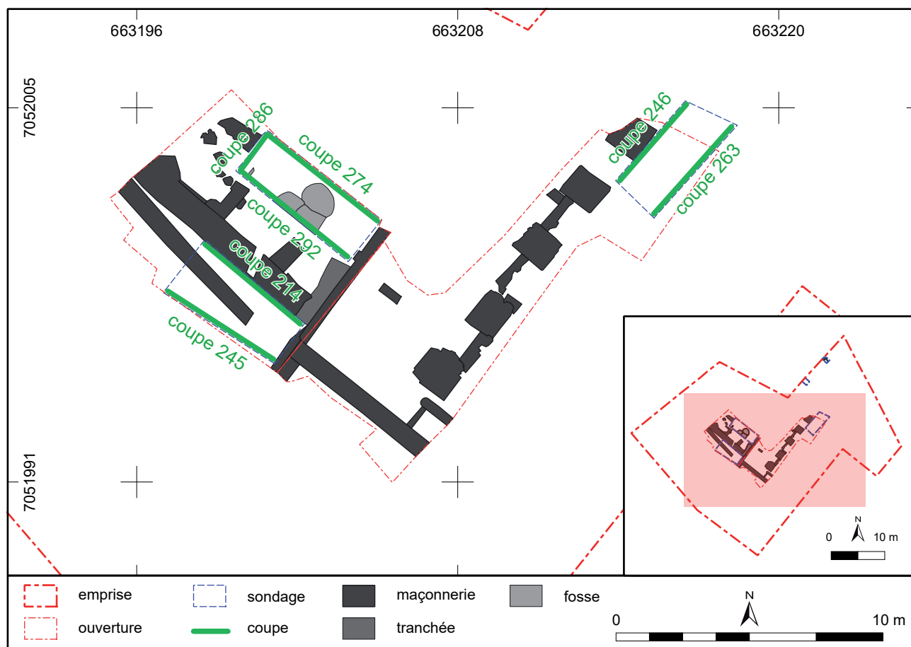
Fig. 19 : Lillers, place de l'Église, plan de localisation des coupes stratigraphiques, O. Dewitte - DA, CD 62.
