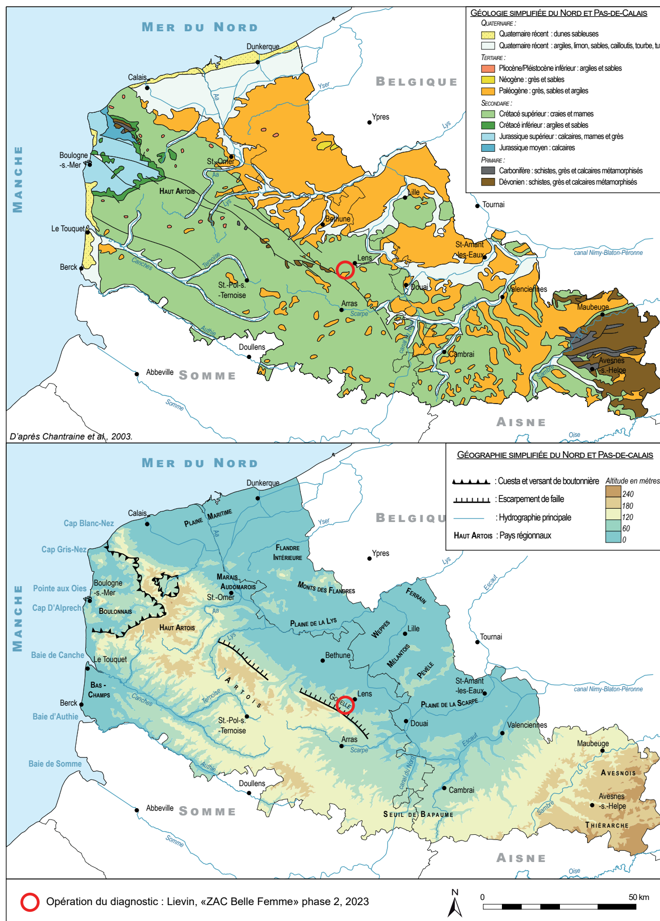
Fig. 7: Liévin, «ZAC de la Belle Femme», phase 2, le projet dans son environnement géologique, extrait de la carte géologique au millionième (Chantraine et al. 2003 ; BRGM-Infoterre 2019), A. Beauchamp- DA CD62.
