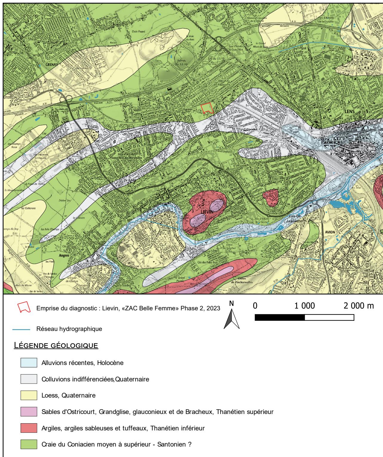
Fig. 8: Liévin, « ZAC de la Belle Femme », phase 2, le projet dans son environnement géologique, extrait de la carte géologique au 1/50 000 e harmonisée (Lacquement et al. 2004 ; BRGM-Infoterre 2023), A. Beauchamp - DA CD62.
