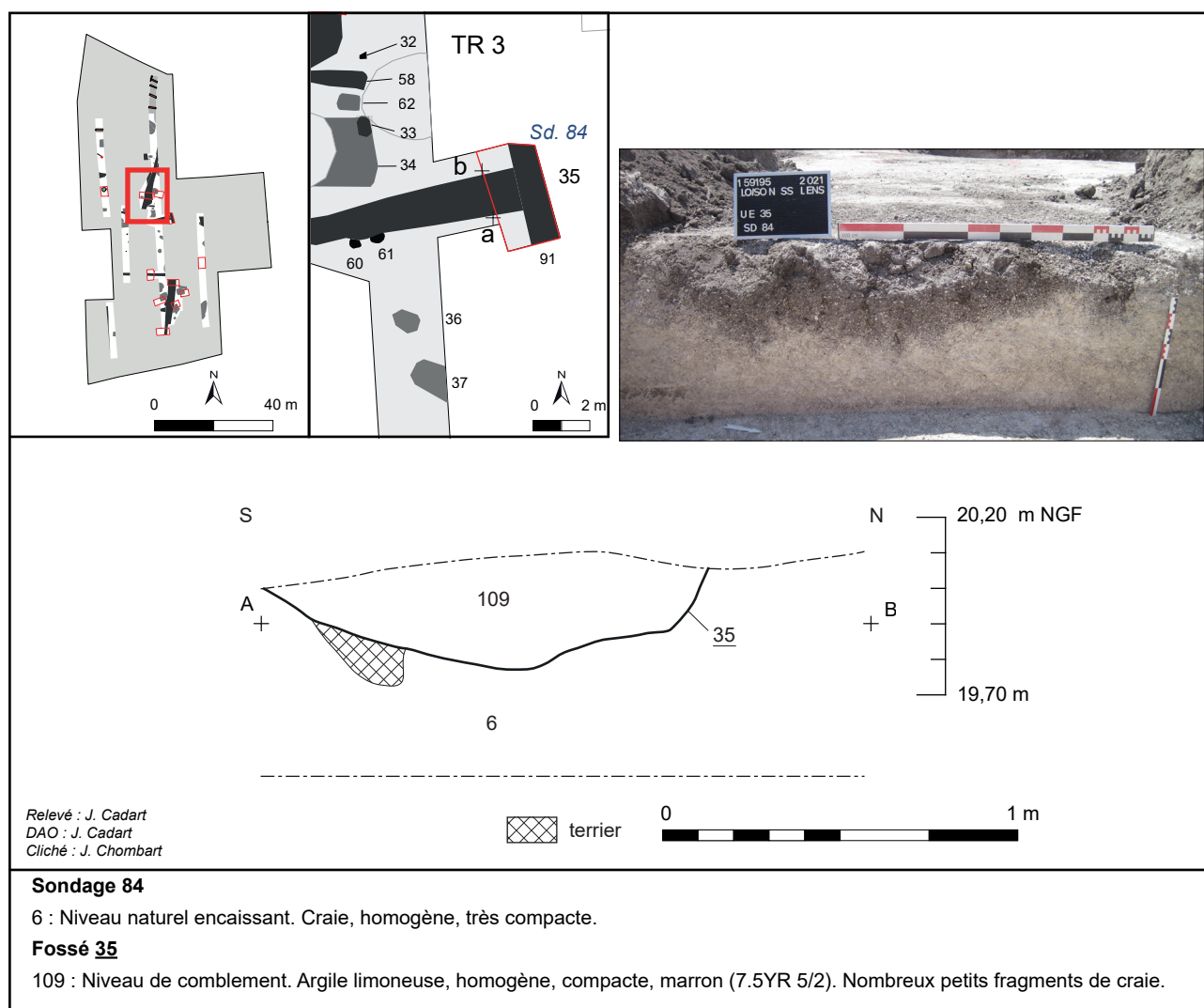
Fig. 31 : Loison-sous-Lens, Rue Léon Blum, vue et coupe du fossé 35, sondage 84, J. Cadart - DA, CD 62.
