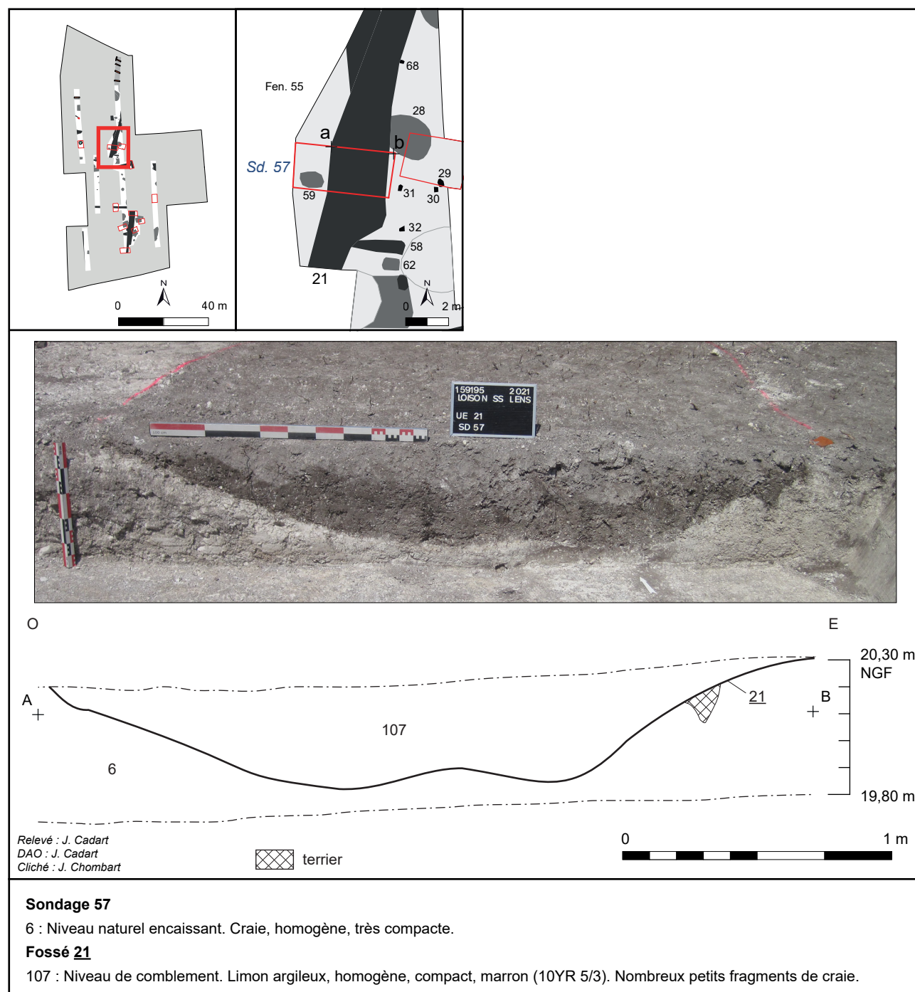
Fig. 21 : Loison-sous-Lens, Rue Léon Blum, vue et coupe du fossé 21, sondage 57, J. Cadart - DA, CD 62.
