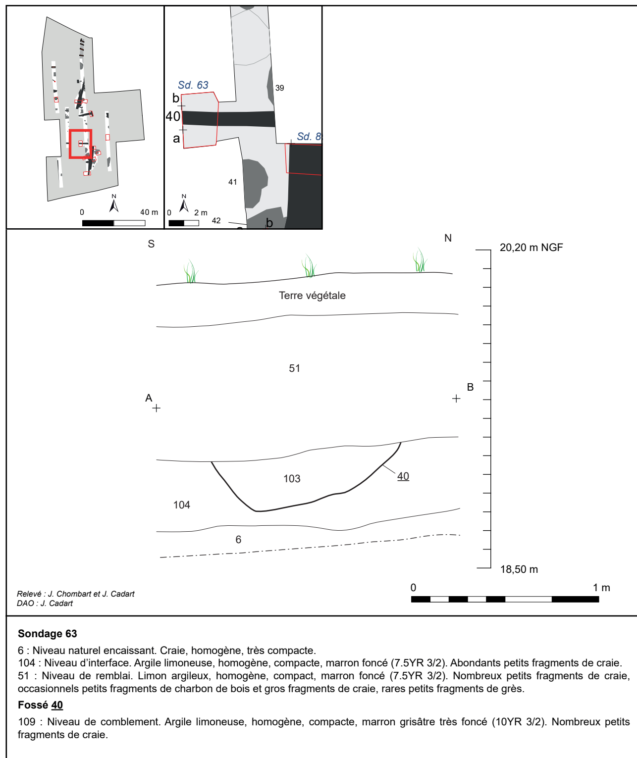
Fig. 25 : Loison-sous-Lens, Rue Léon Blum, coupe du fossé 40, sondage 63, J. Cadart - DA, CD 62.
