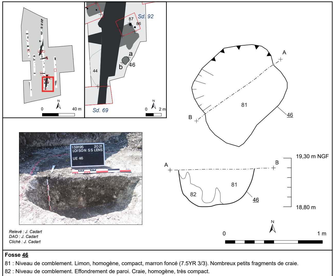
Fig. 33 : Loison-sous-Lens, Rue Léon Blum, vue, plan et coupe de la fosse 46, J. Cadart - DA, CD 62.
