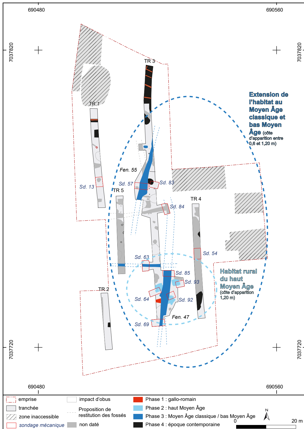
Fig. 37 : Loison-sous-Lens, Rue Léon Blum, plan de synthèse au 1/600e, J. Chombart - DA, CD 62.
