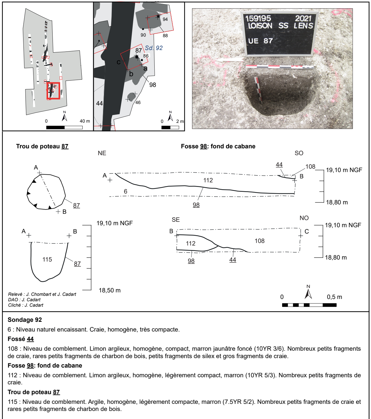
Fig. 20 : Loison-sous-Lens, Rue Léon Blum, coupes de la fosse 88 et vue, plan et coupe du poteau 94, sondage 92, J. Cadart - DA, CD 62.
