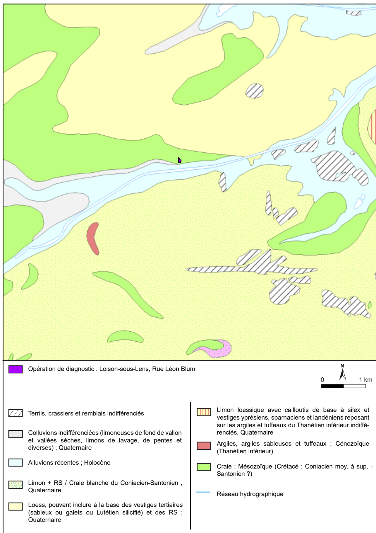
Fig. 8 : Loison-sous-Lens, Rue Léon Blum, extrait de la carte géologique au 1/50 000 harmonisée (Lacquement et al. 2004 ; BRGM-Infoterre 2021), M. Meurisse-Fort et J. Chombart- DA, CD 62.
