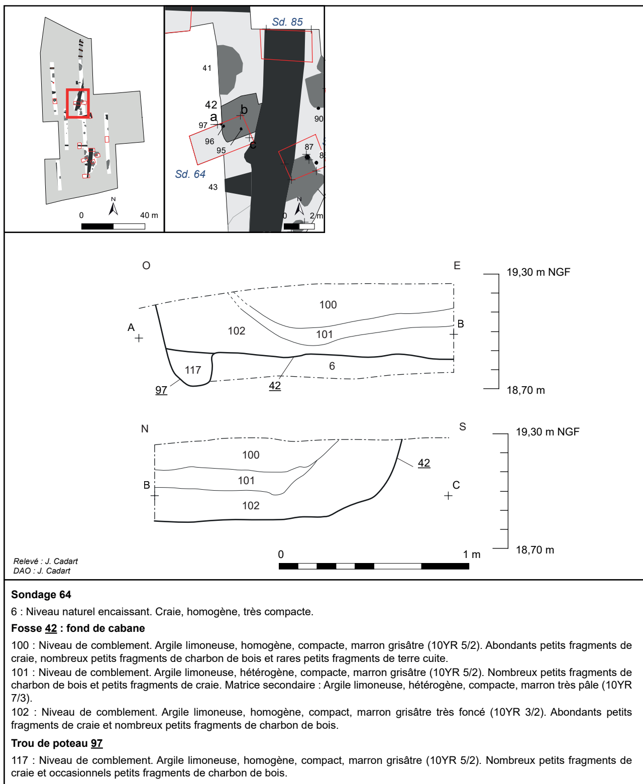
Fig. 16 : Loison-sous-Lens, Rue Léon Blum, coupes de la fosse 42 et du poteau 97, sondage 64, J. Cadart - DA, CD 62.
