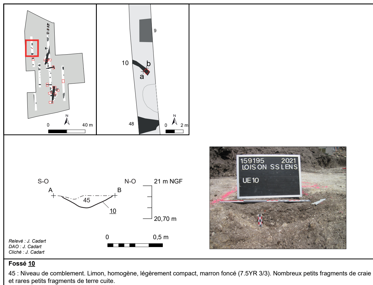
Fig. 30 : Loison-sous-Lens, Rue Léon Blum, vue et coupe du fossé 10, J. Cadart - DA, CD 62.
