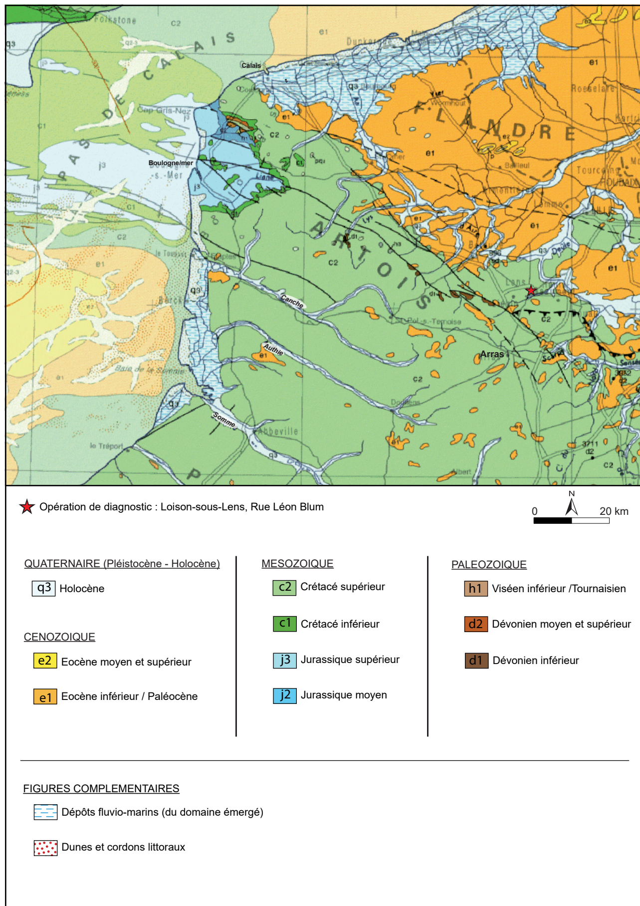
Fig. 7 : Loison-sous-Lens, Rue Léon Blum, extrait de la carte géologique au millionième (Chantraine et al. 1996 ; BRGM-Infoterre 2021), M. Meurisse-Fort - DA, CD 62.
