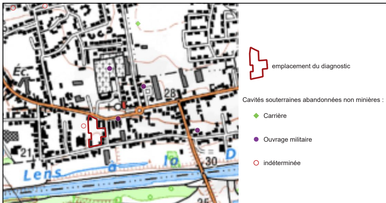
Fig. 6 : Loison-sous-Lens, Rue Léon Blum, extrait de la carte de l'aléa cavité (BRGM-Infoterre 2021) avec l'emplacement du diagnostic, J. Chombart - DA, CD 62.
