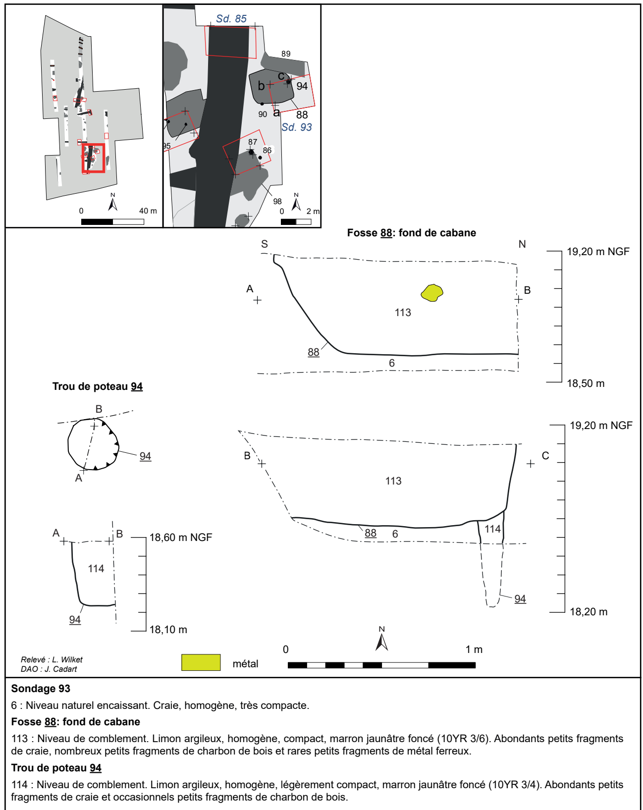
Fig. 18 : Loison-sous-Lens, Rue Léon Blum, coupes de la fosse 88 et plan et coupe du poteau 94, sondage 93, J. Cadart - DA, CD 62.
