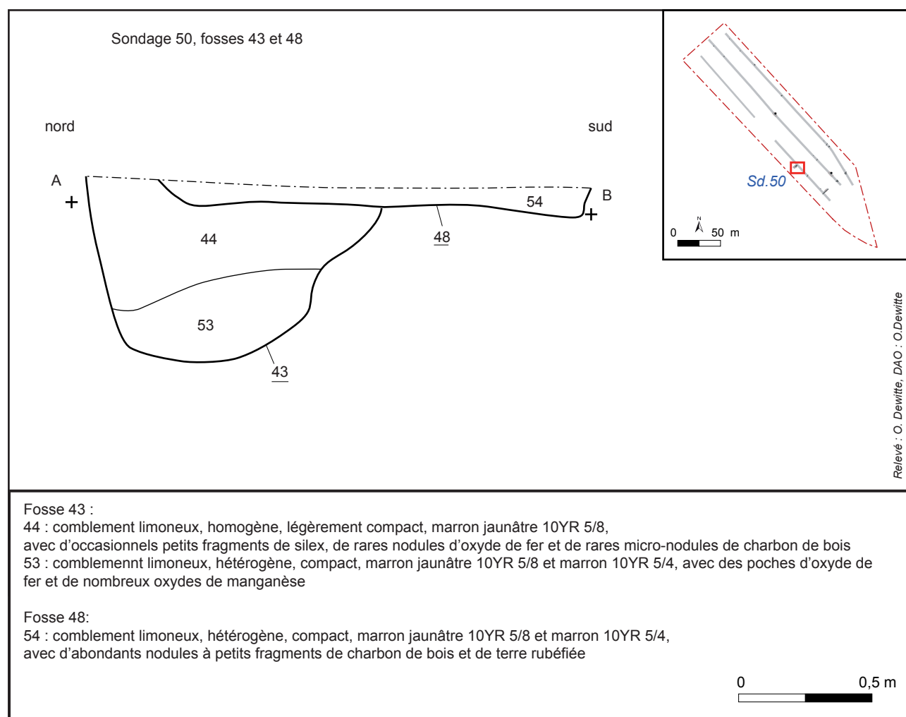
Fig. 17 : Longuenesse, rue Ambroise Paré, coupe des fosses 43 et 48, sondage 50, tranchée 3, O. Dewitte - DA, CD 62.
