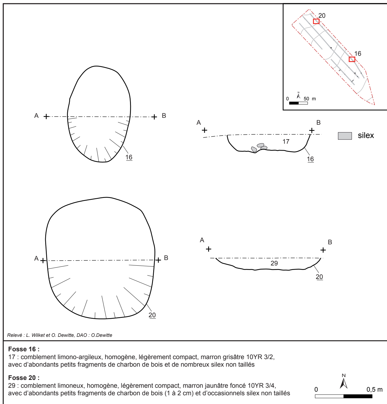
Fig. 12 : Longuenesse, rue Ambroise Paré, coupes et plans des fosses 16 et 20, O. Dewitte - DA, CD 62.
