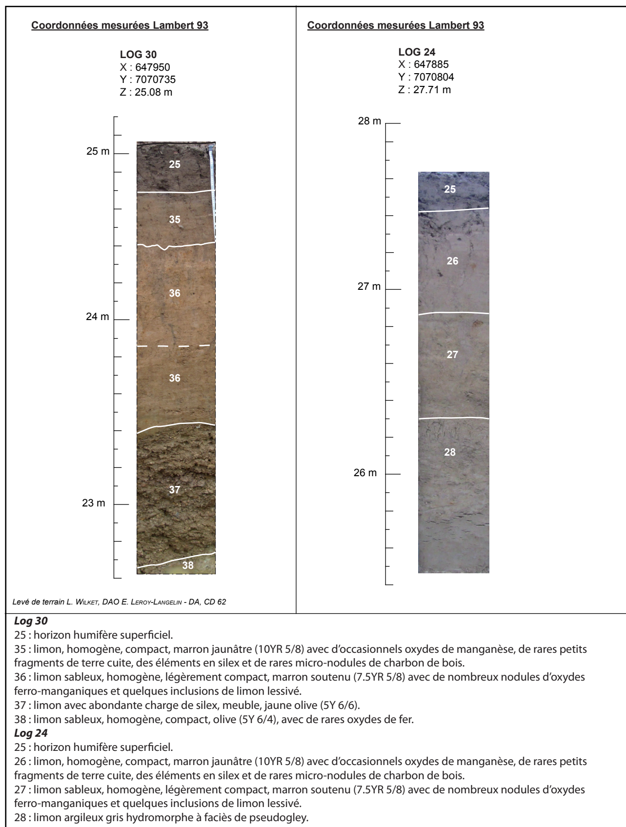
Fig. 11 : Longuenesse, rue Ambroise Paré, relevés des logs réalisés sur le diagnostic, E. Leroy-Langelin - DA, CD 62.
