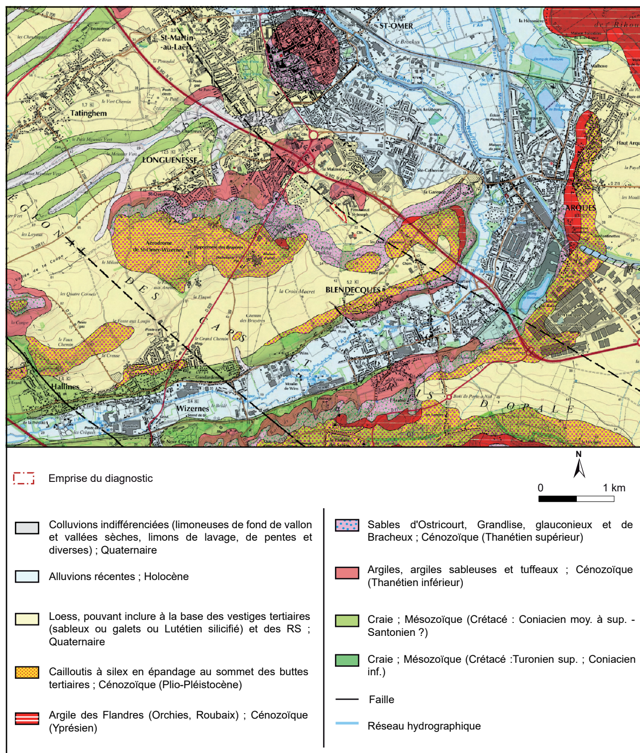
Fig. 7 : Longuenesse, rue Ambroise Paré, extrait de la carte géologique au 1/50 000 harmonisée (Lacquement et al. 2004 ; BRGM-Infoterre 2018)
