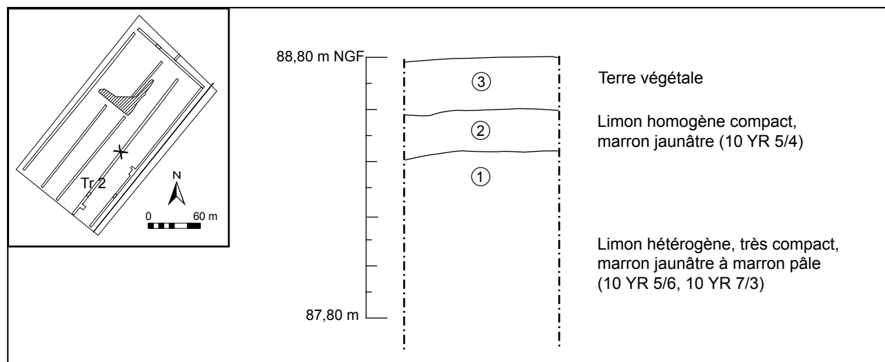
Fig. 5 : Maroeuil, ZAL Brunehaut, coupe de la couverture sédimentaire superficielle dans la tranchée 2 (voir photographie fig. 6).
