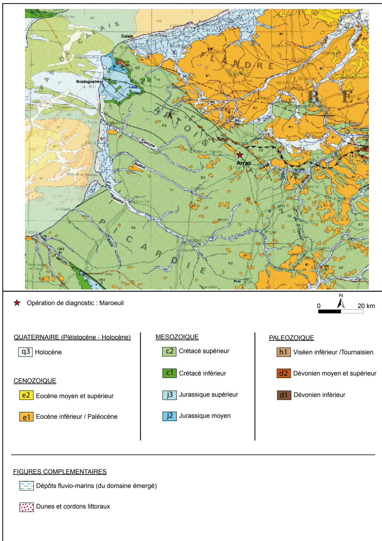
Fig. 7 : Maroeuil, ZAL Brunehaut, extrait de la carte géologique au millionième (BRGM-Infoterre 2009 ; Chanteraine et alii. 1996).
