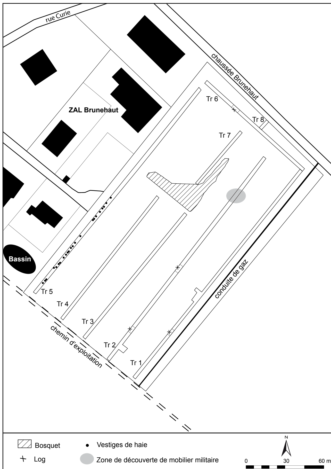
Fig. 8 : Maroeuil, ZAL Brunehaut, plan d'implantation des tranchées.
