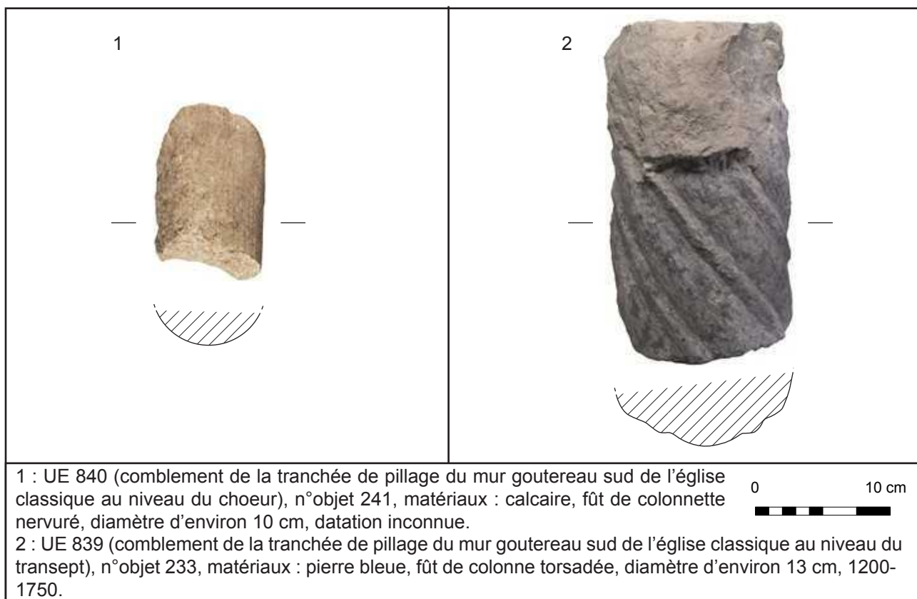
Fig. 120 : Mont-Saint-Eloi, support : colonnette appartenant au module de moins de 10 cm. et colonne appartenant au module de 12 - 13 cm. de diamètre.
