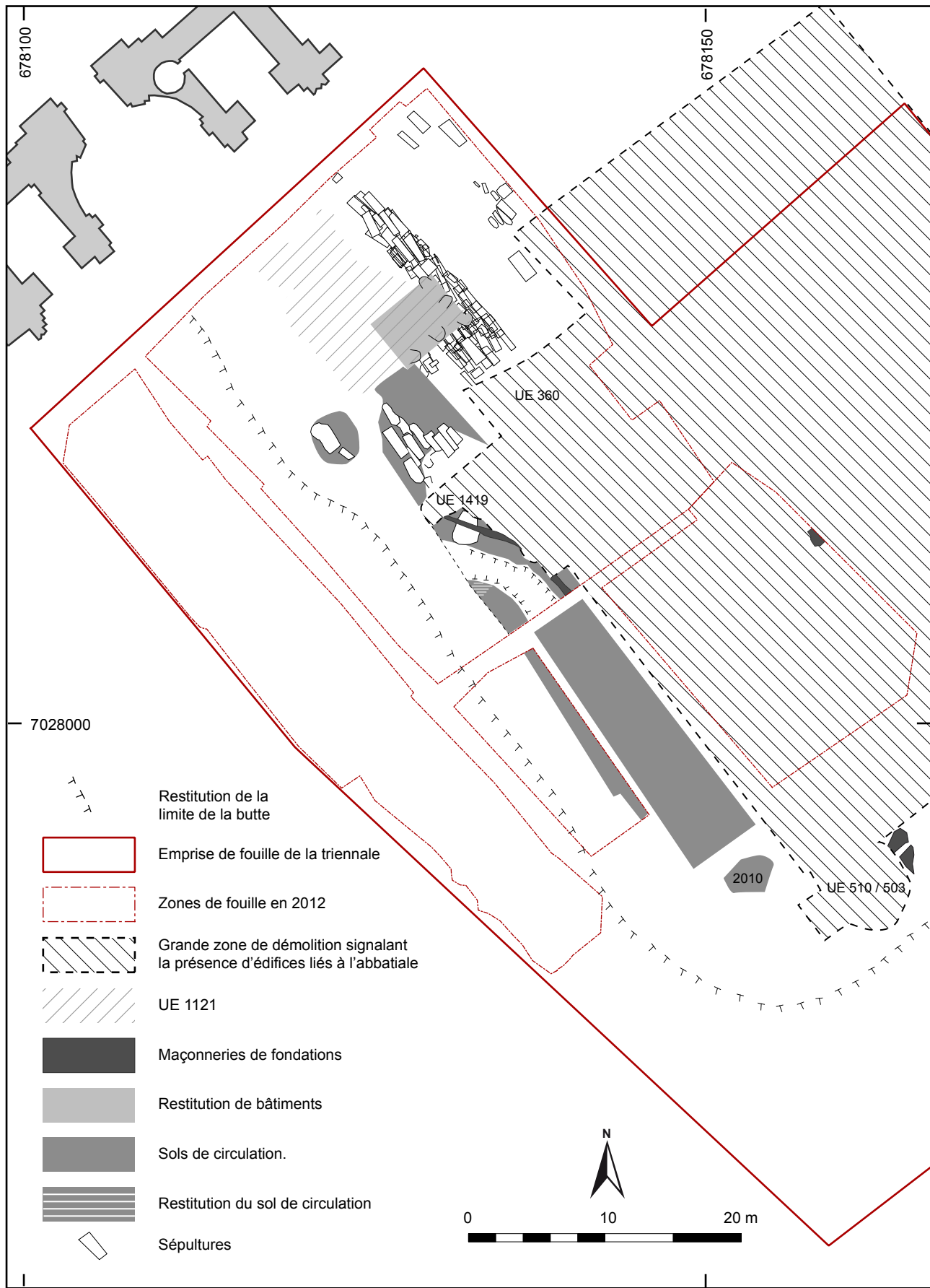
Fig. 45 : Mont-Saint-Eloi, plan général des vestiges appartenant à la période II-phase E-1.
