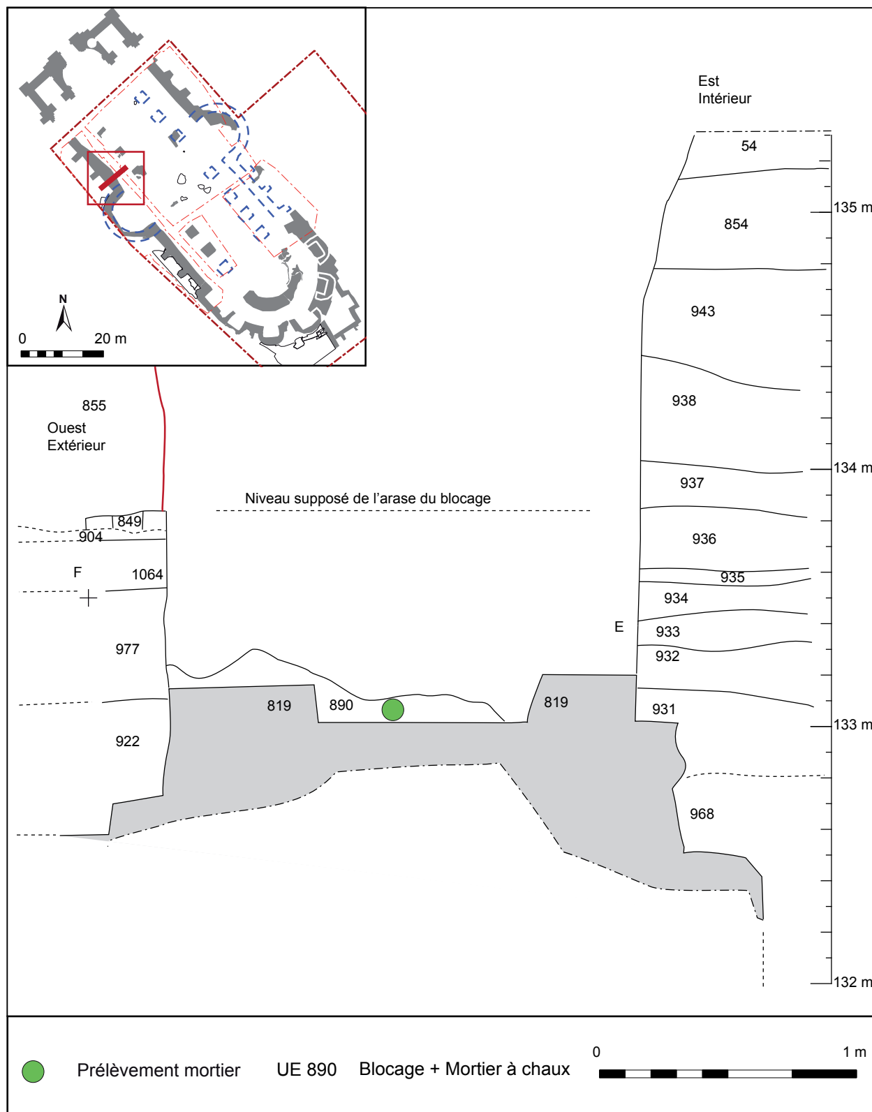
Fig. 107 : Mont-Saint-Eloi, relevé en coupe de la dalle de fondation du mur gouttereau et des niveaux de remblais déposés à l'intérieur et à l'extérieur de la collégiale.
