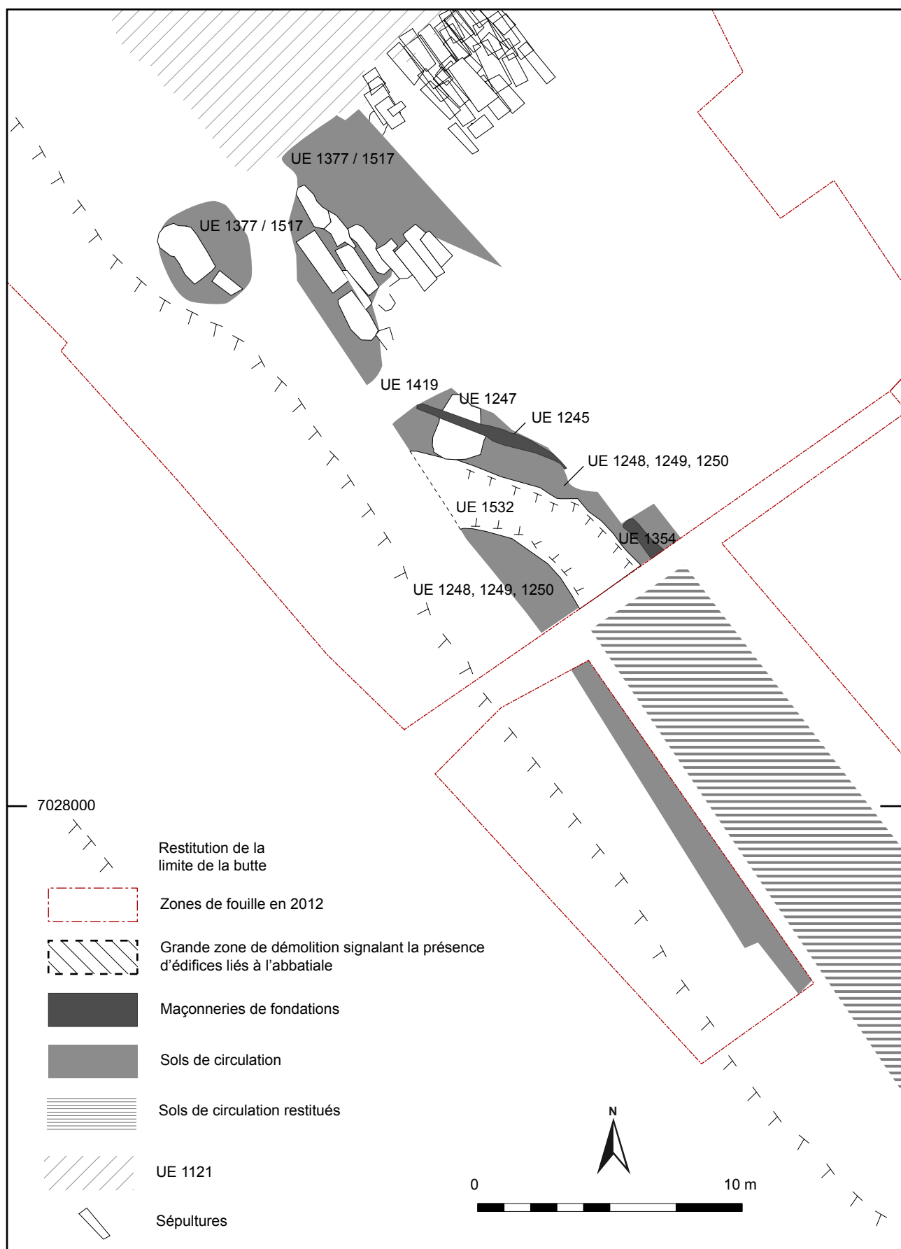
Fig. 49 : Mont-Saint-Eloi, plan de l'emplacement des sols de circulation appartenant à la période II-phase E-1.
