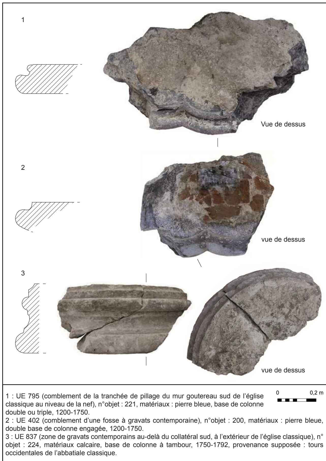
Fig. 124 : Mont-Saint-Eloi, support : bases de colonne.
