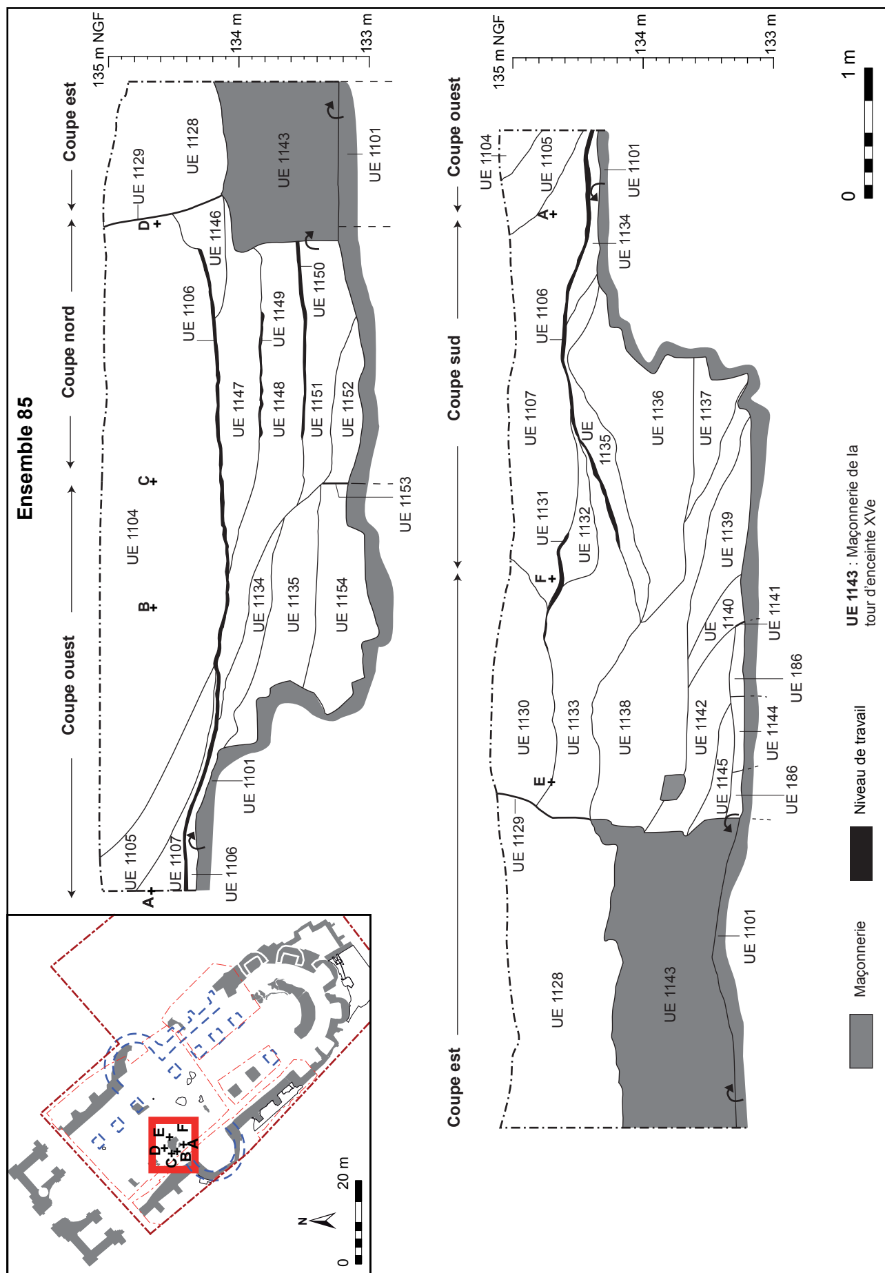
Fig. 116 : Mont-Saint-Eloi, relevé de la coupe du pilier 4 (UE 85).
