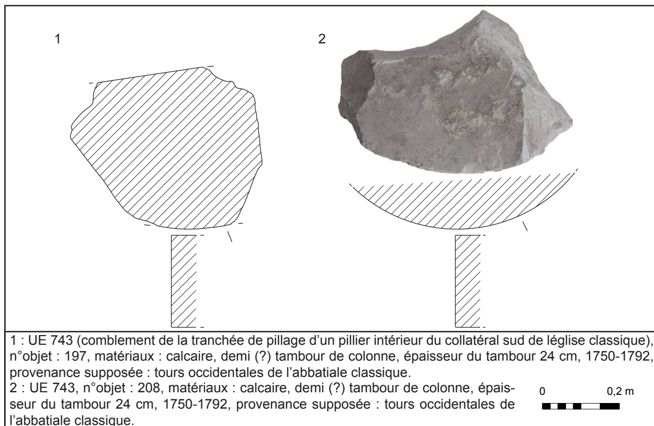
Fig. 122 : Mont-Saint-Eloi, support : tambour de colonne d'un diamètre de 78 cm.
