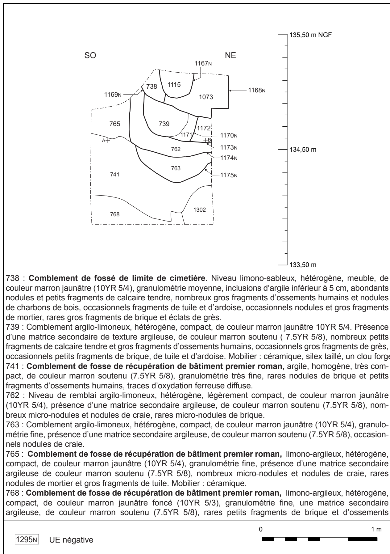
Fig. 42 : Mont-Saint-Eloi, relevé de la coupe ENS 1462 (localisation cf. fig. 40).
