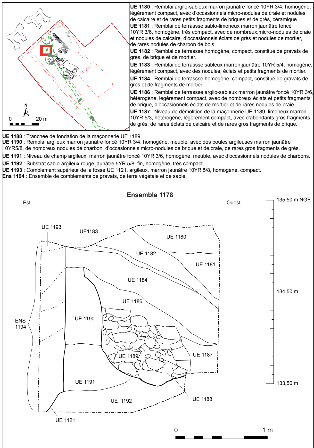
Fig. 64 : Mont-Saint-Eloi, relevé de la coupe ENS 1178.
