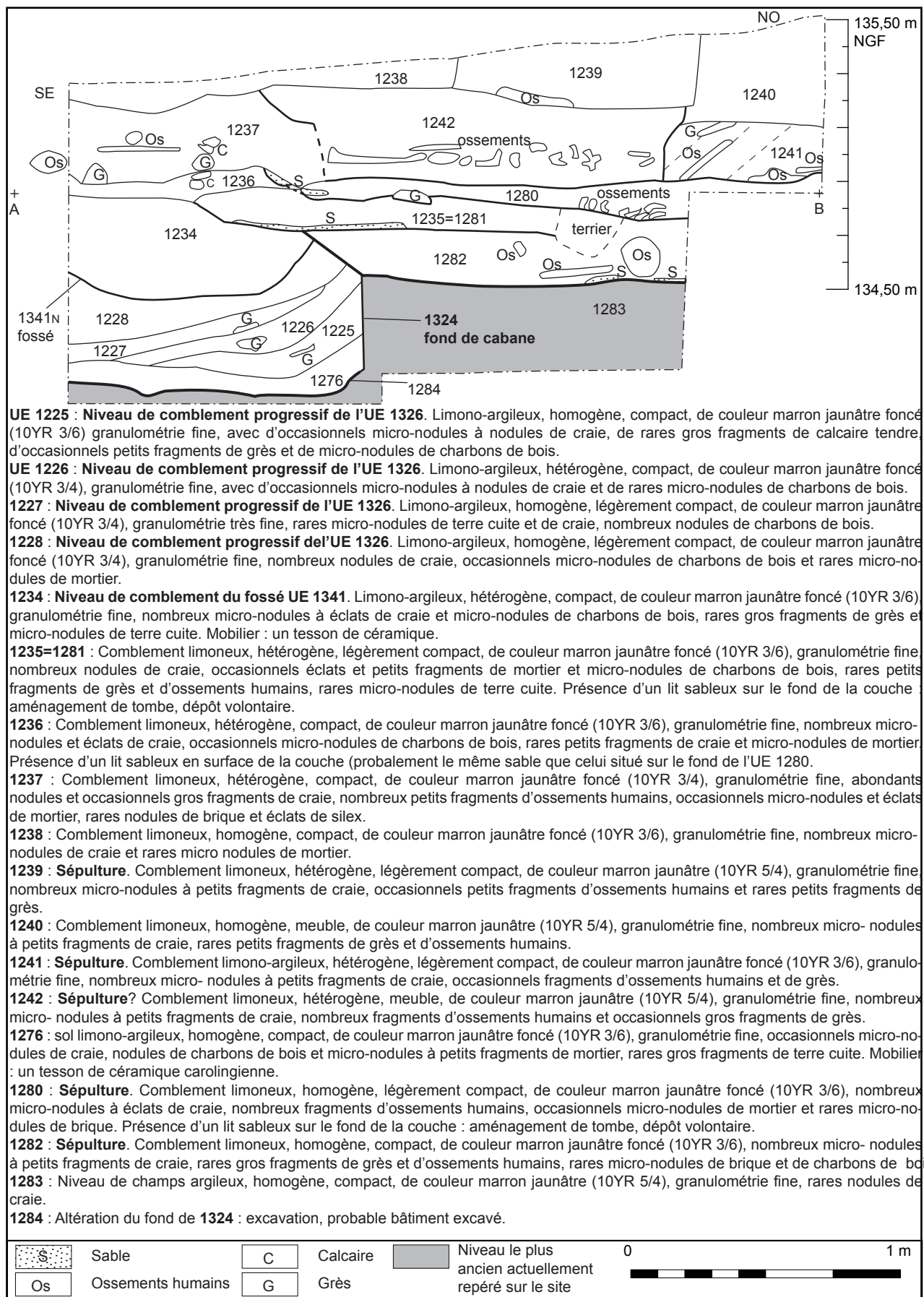
Fig. 29 : Mont-Saint-Eloi, relevé de la coupe UE 1205, avec l'excavation UE 1324, scellée par les niveaux de cimetières.
