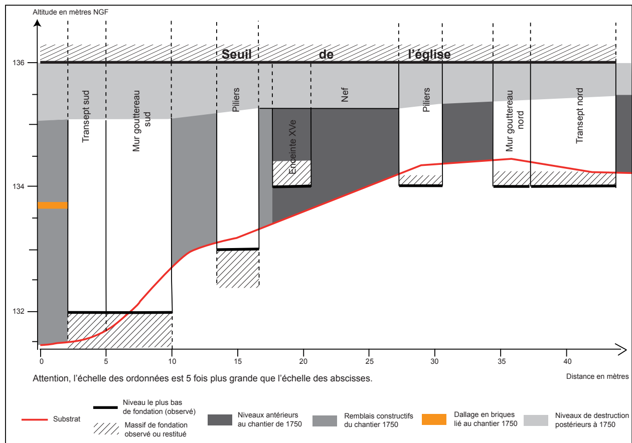
Fig. 102 : Mont-Saint-Eloi, coupe schématique d'ouest en est de la butte, des fondations de l'église classique et du rehaussement par des remblais du terrain lors du chantier de construction.
