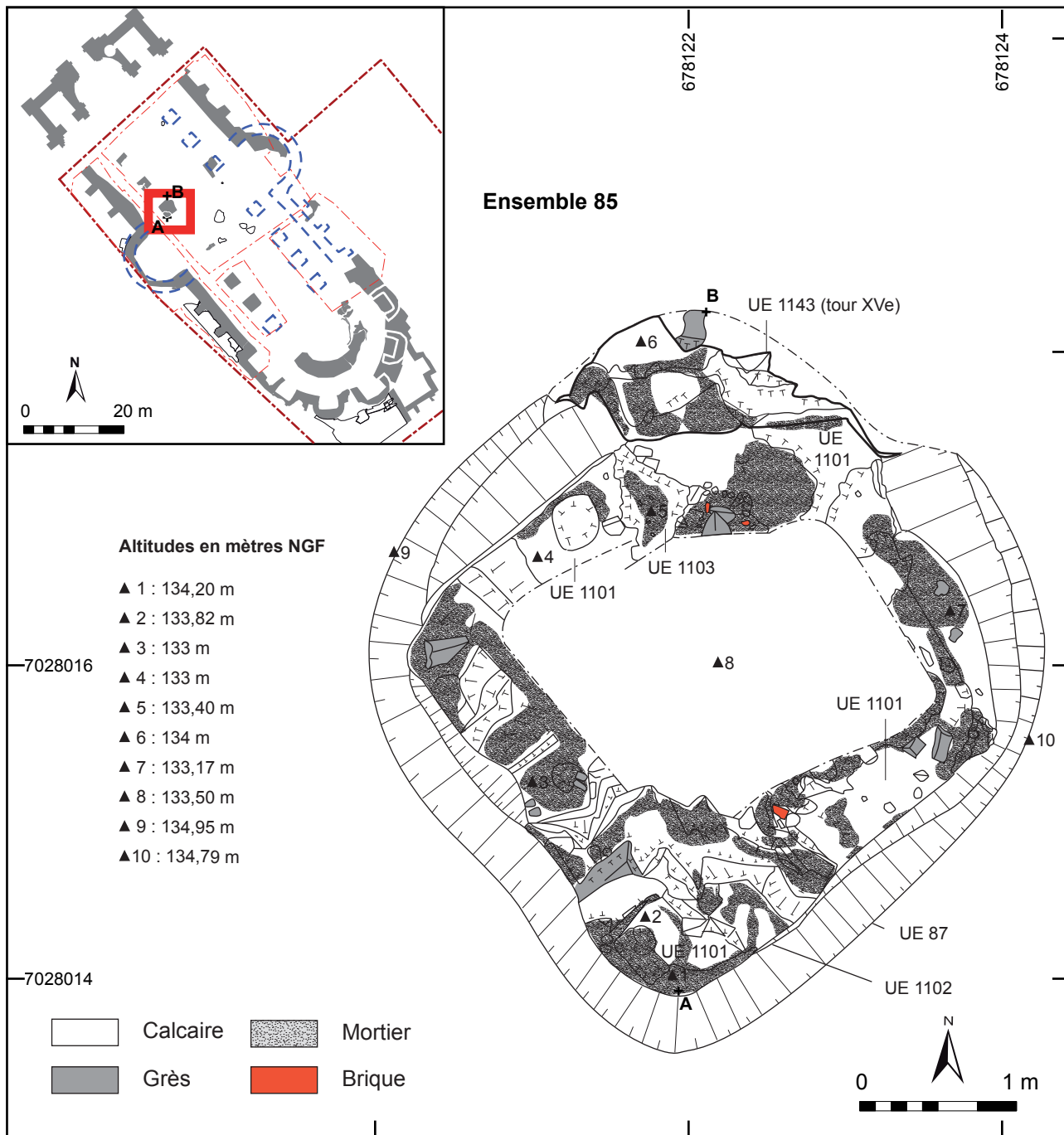
Fig. 115 : Mont-Saint-Eloi, relevé en plan du pilier 4 (UE 85)
