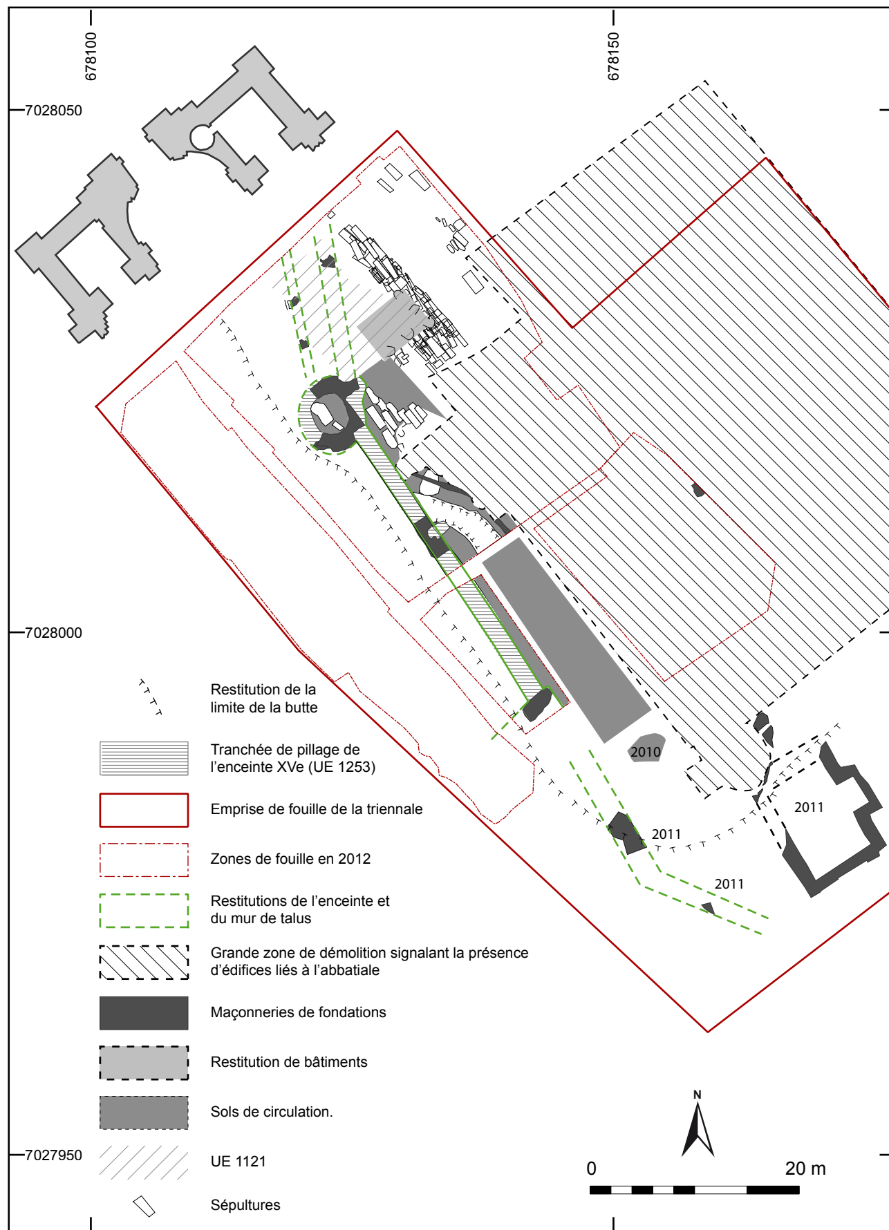
Fig. 27 : Mont-Saint-Eloi, plan général des vestiges appartenant à la période II.
