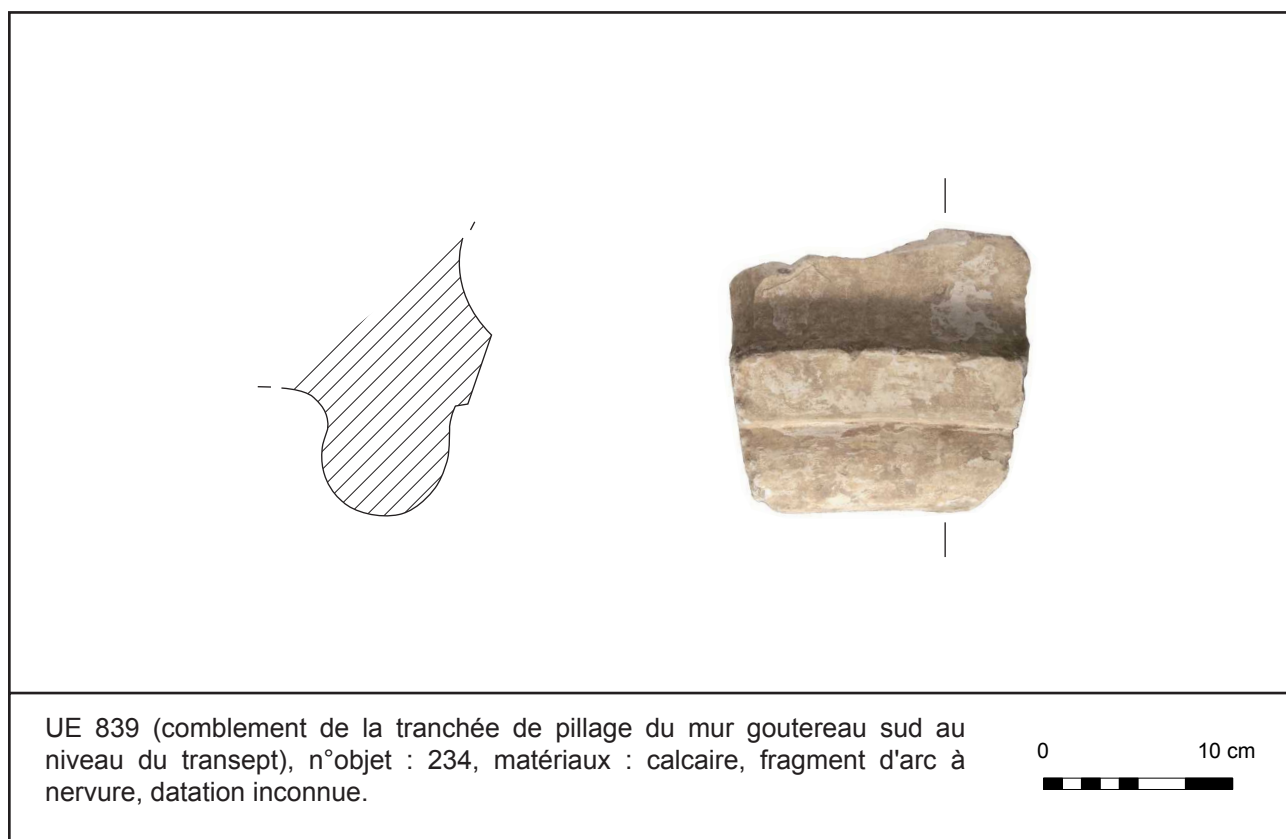
Fig. 126 : Mont-Saint-Eloi, couverture : voûtement.
