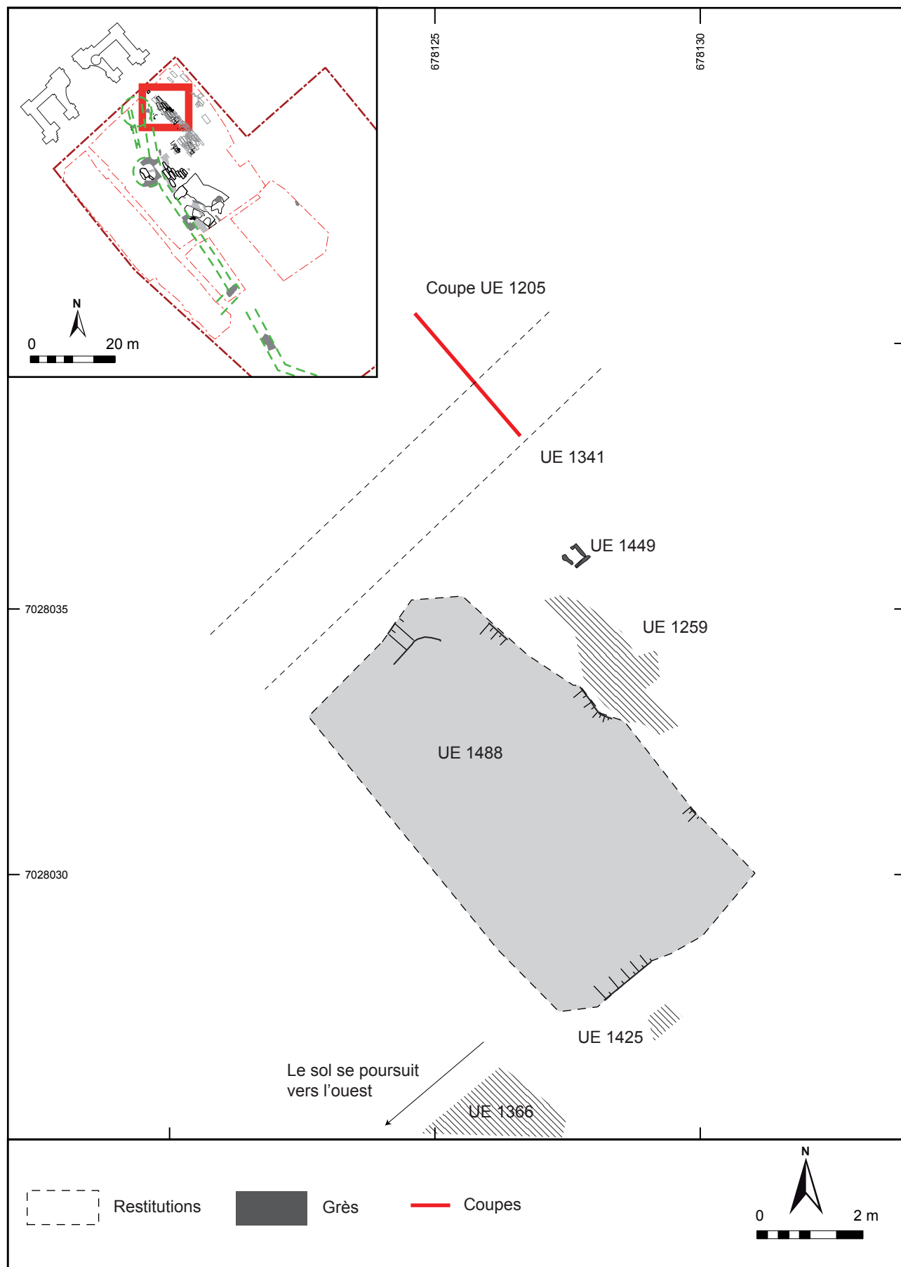
Fig. 33 : Mont-Saint-Eloi, plan général des vestiges appartenant à la période II-phase D-1.
