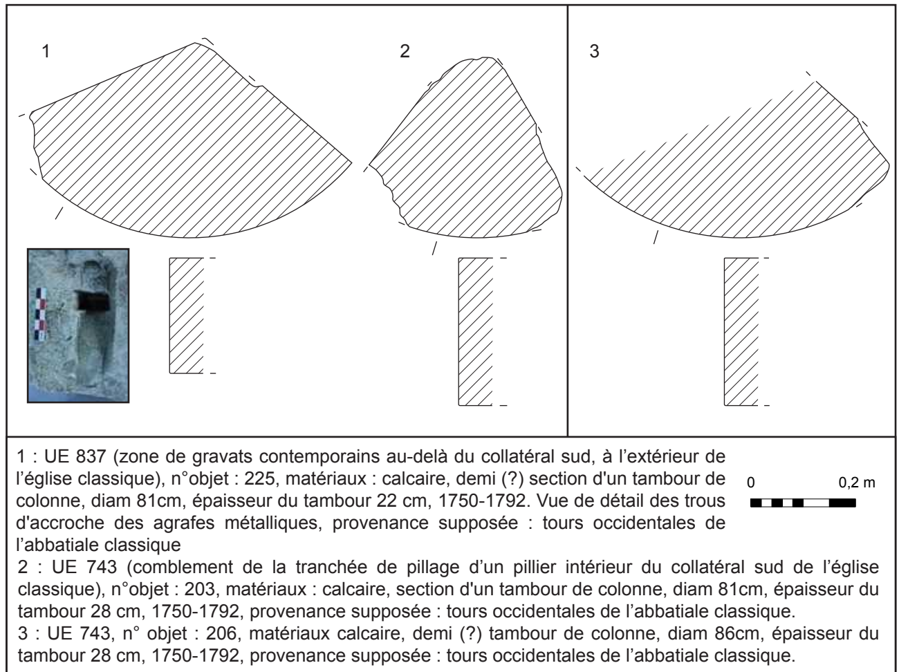
Fig. 123 : Mont-Saint-Eloi, support : tambour de colonne d'un diamètre de 81 cm. à 86 cm.
