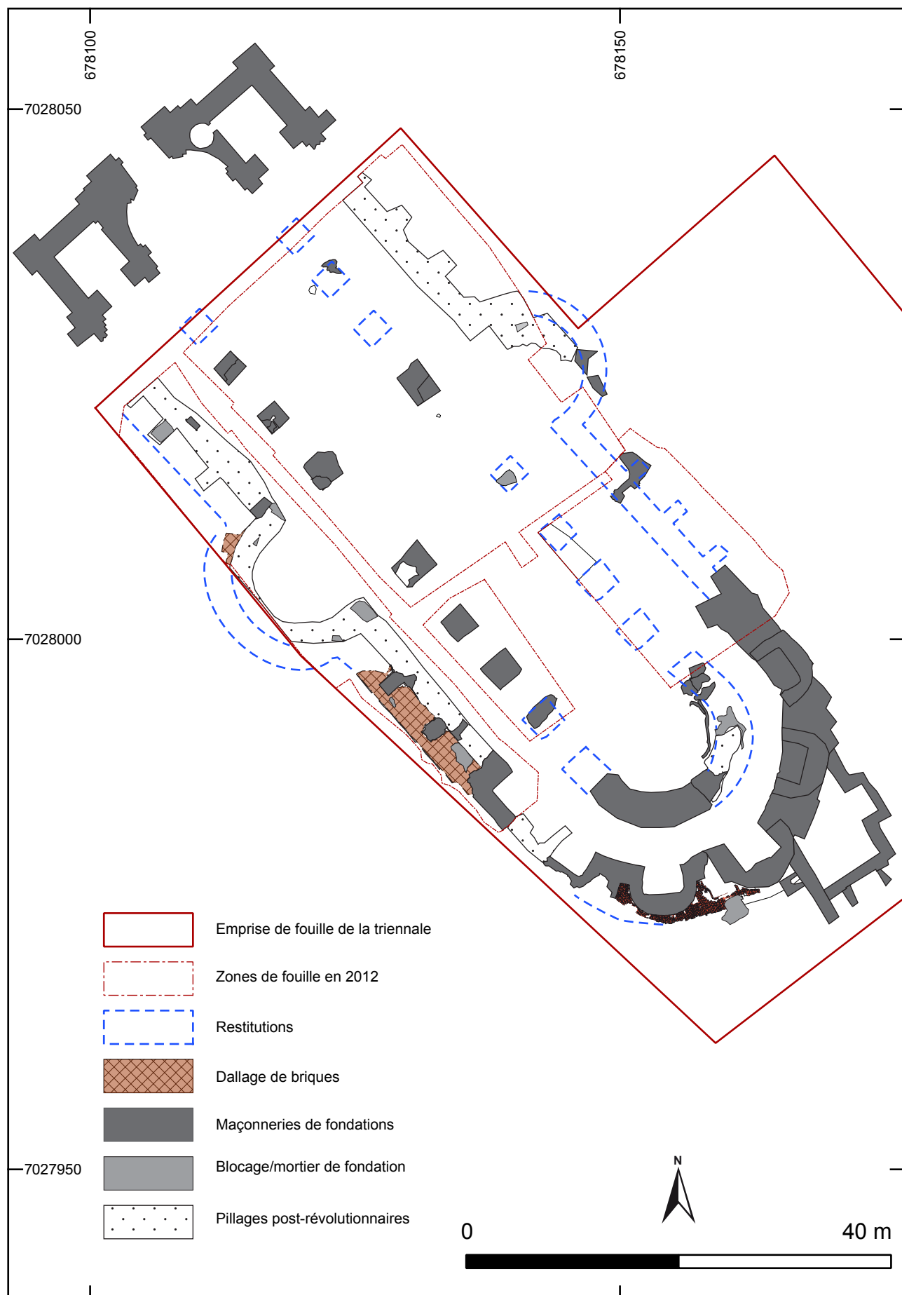
Fig. 101 : Mont-Saint-Eloi, plan général de l'abbatiale classique.
