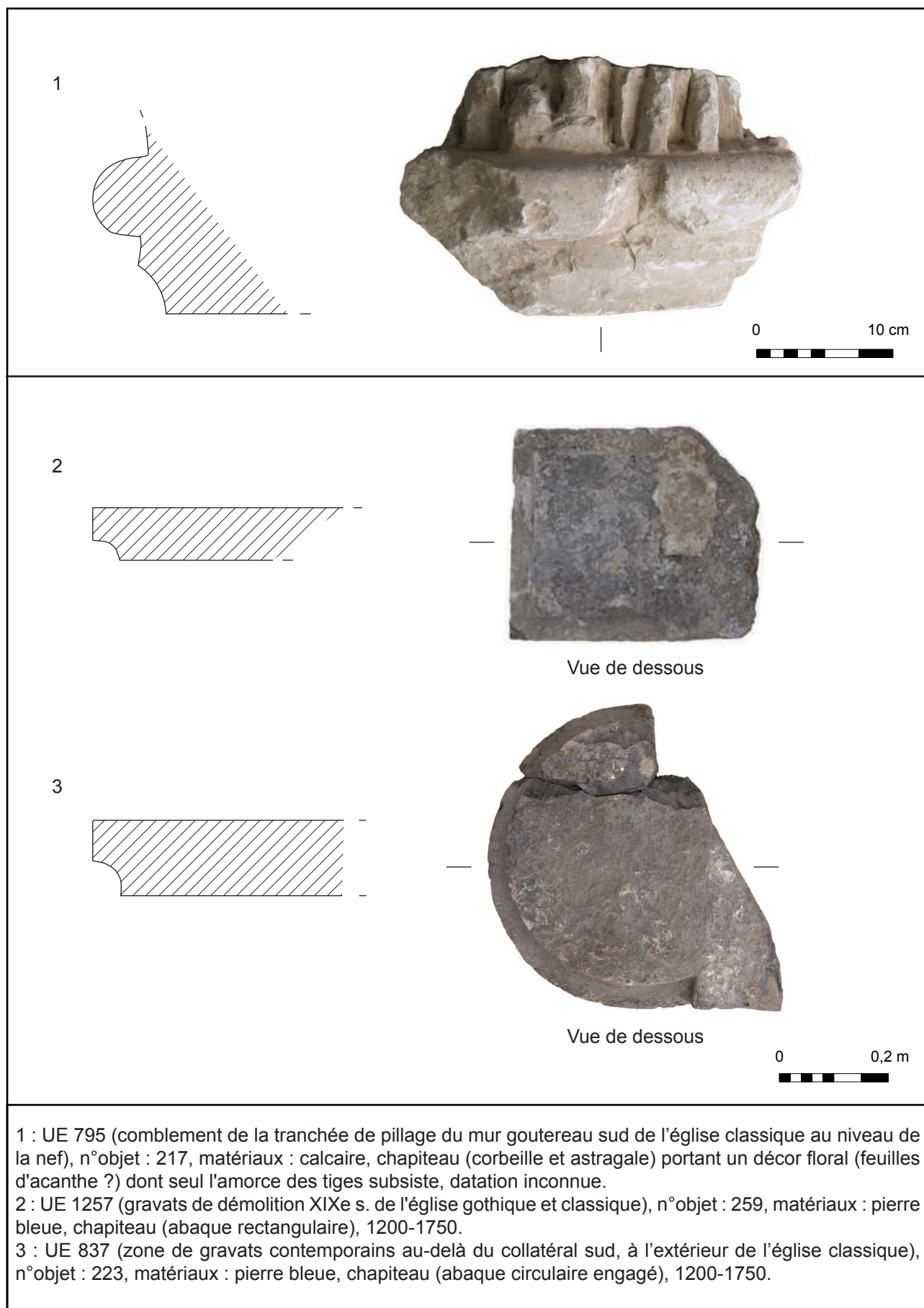
Fig. 125 : Mont-Saint-Eloi, support, chapiteaux : corbeille et abaqes.
