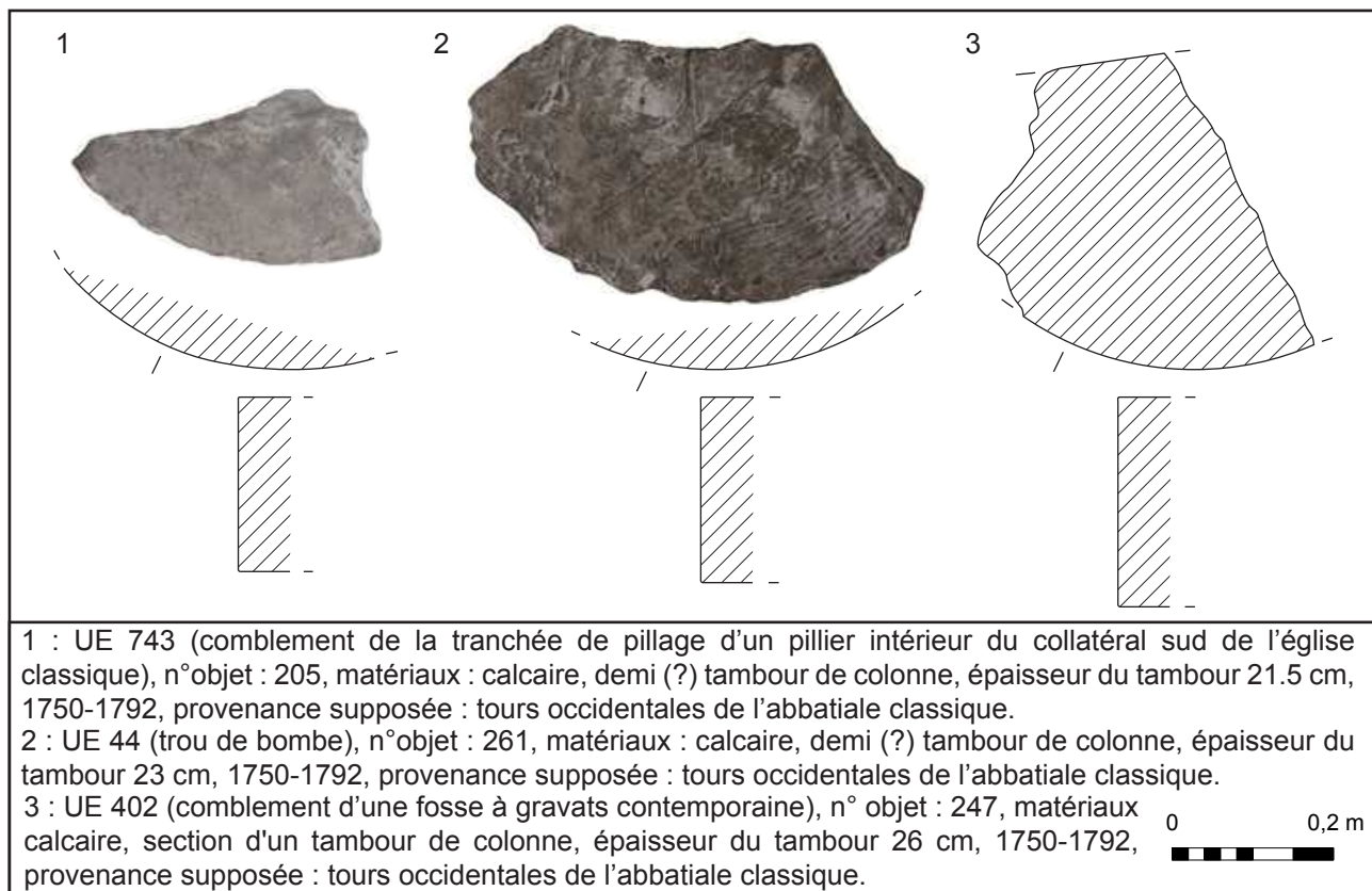
Fig. 121 : Mont-Saint-Eloi, support : tambour de colonne d'un diamètre approximatif de 75 cm.
