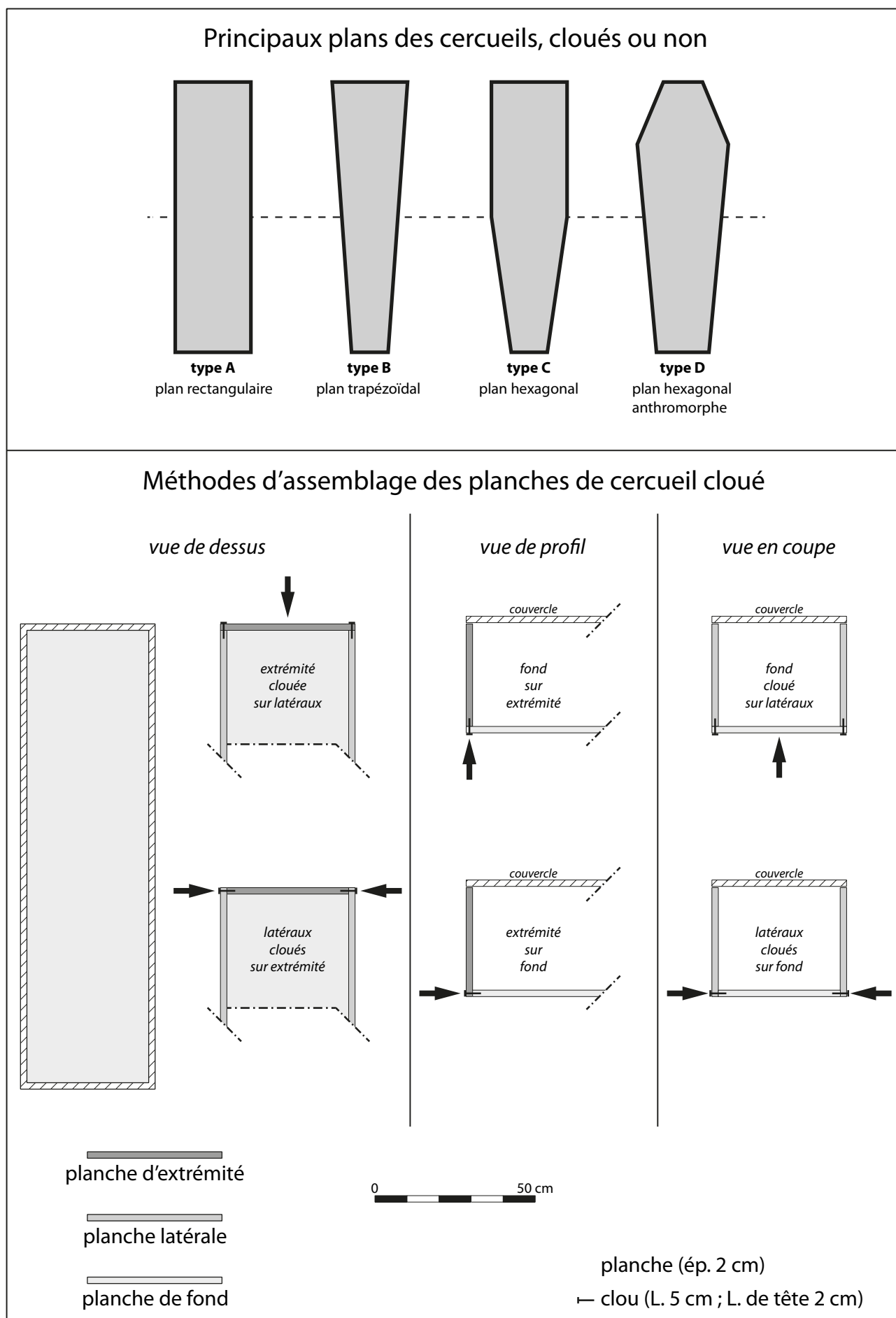
Fig. 75 : Mont-Saint-Eloi, plans des cercueils et méthodes d'assemblage des planches de cercueil cloué.
