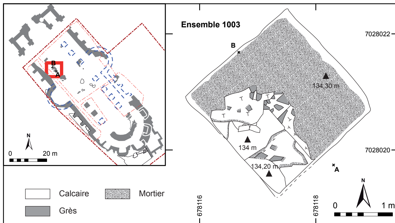
Fig. 113 : Mont-Saint-Eloi, relevé du pilier 3 (UE 1003).
