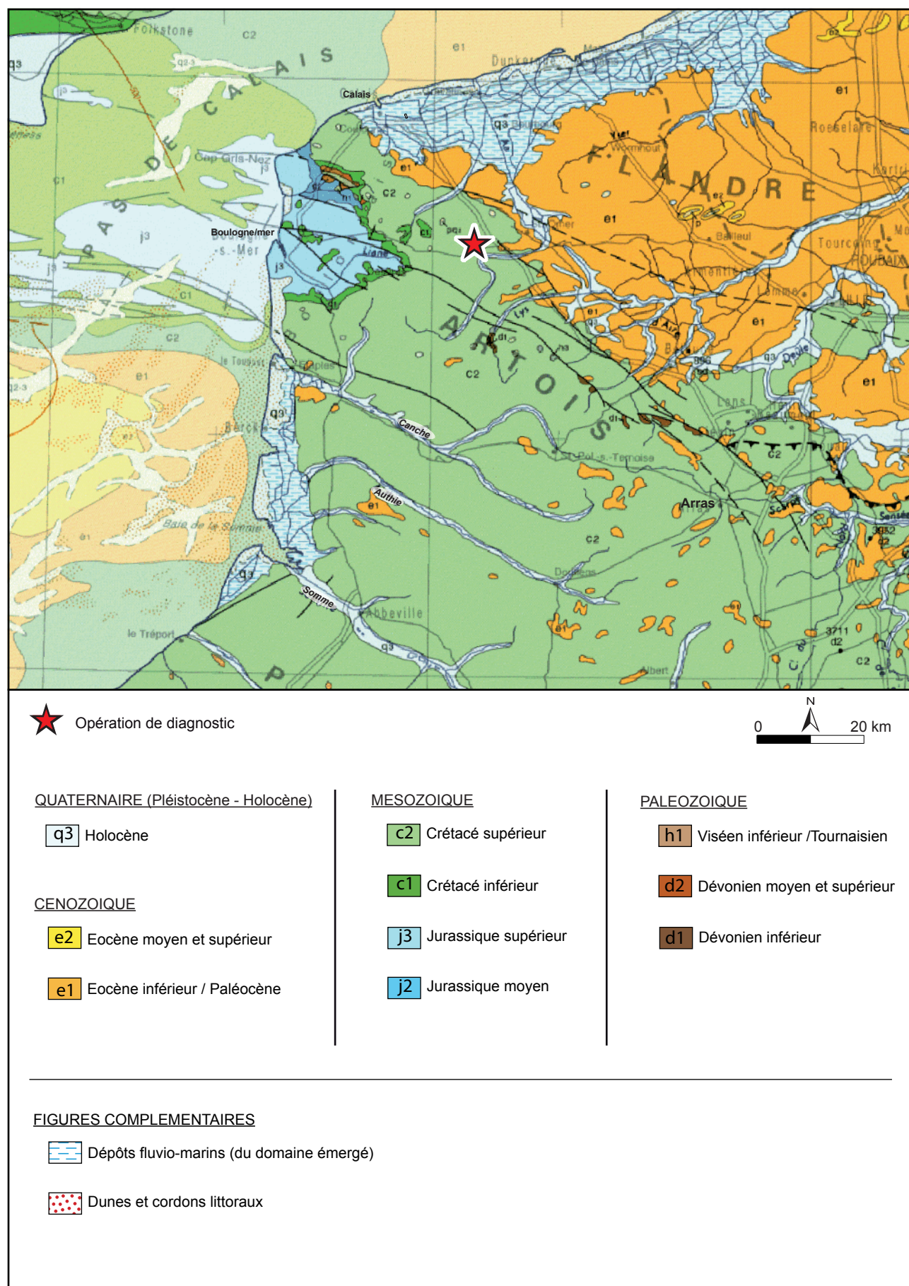
Fig. 5 : Quelmes, Dicloye, extrait de la carte géologique au millionième (Chantraine et al. 1996 ; BRGM-Infoterre 2018), M. Meurisse-Fort - DA, CD 62.
