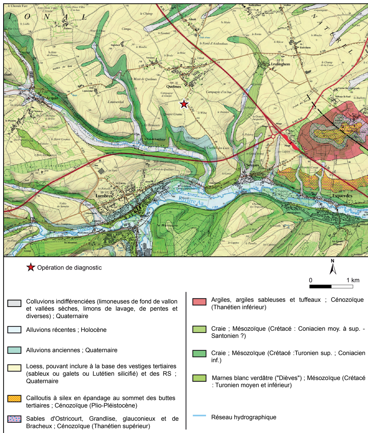
Fig. 6 : Quelmes, Dicloye, extrait de la carte géologique au 1/50 000 harmonisée (Lacquement et al. 2004 ; BRGM-Infoterre 2018), M. Meurisse-Fort - DA, CD 62.
