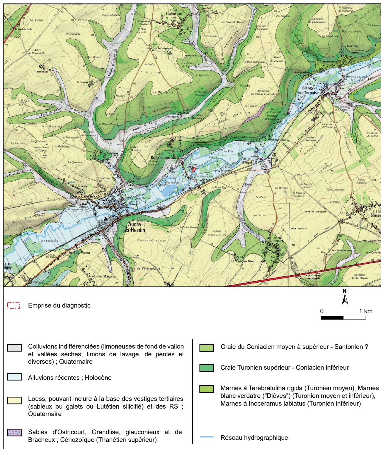
Fig. 6 : Rollancourt, 4 rue du Moulin, extrait de la carte géologique au 1/50 000 harmonisée (Lacquement et al. 2004 ; BRGM-Infoterre 2018)
