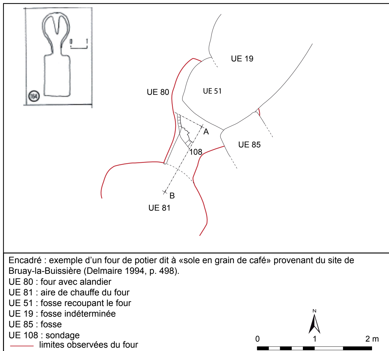
Fig. 19 : Bailleulmont, rue du château, Représentation en plan du four UE 80 et du sondage UE 108, L DALMAU - CDA - CG62
