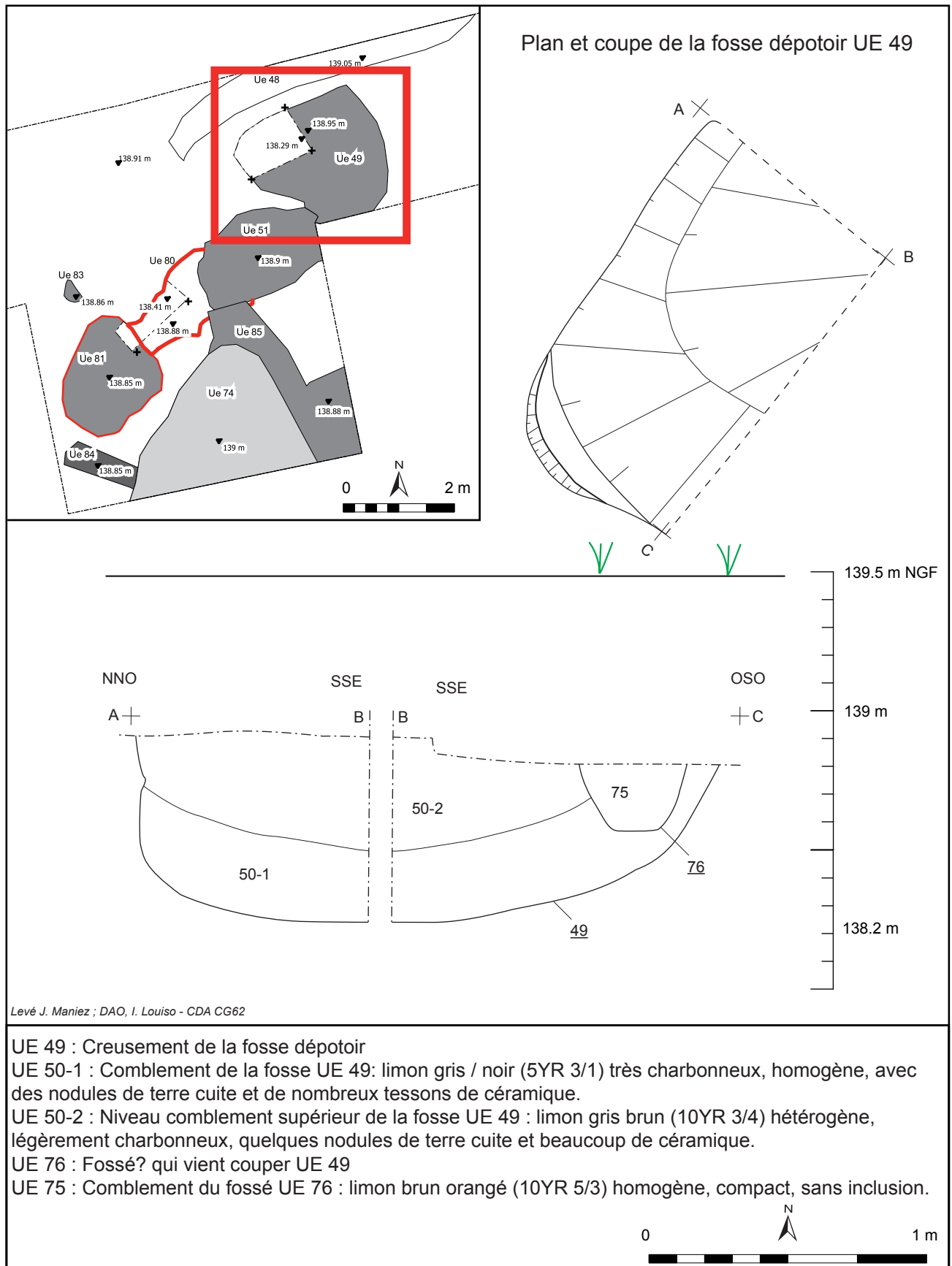
Fig. 24 : Bailleulmont, rue du château, Plan et coupe de la fosse dépotoir UE 49, L. DALMAU - CDA - CG62
