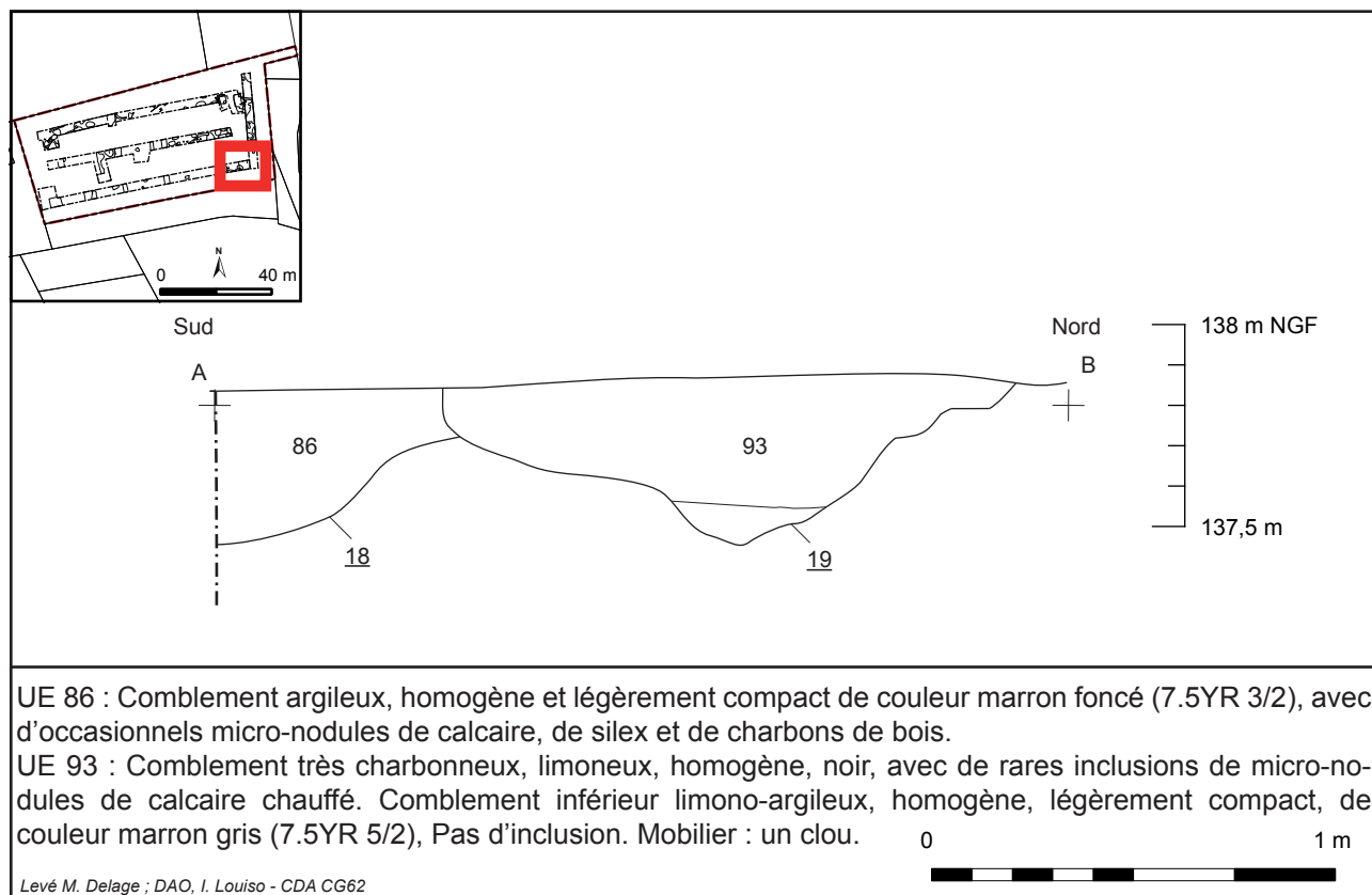
Fig. 58 : Bailleulmont, rue du château, Coupe nord-sud des structures en creux UEs 18 et 19, L. DALMAU - CDA - CG62
