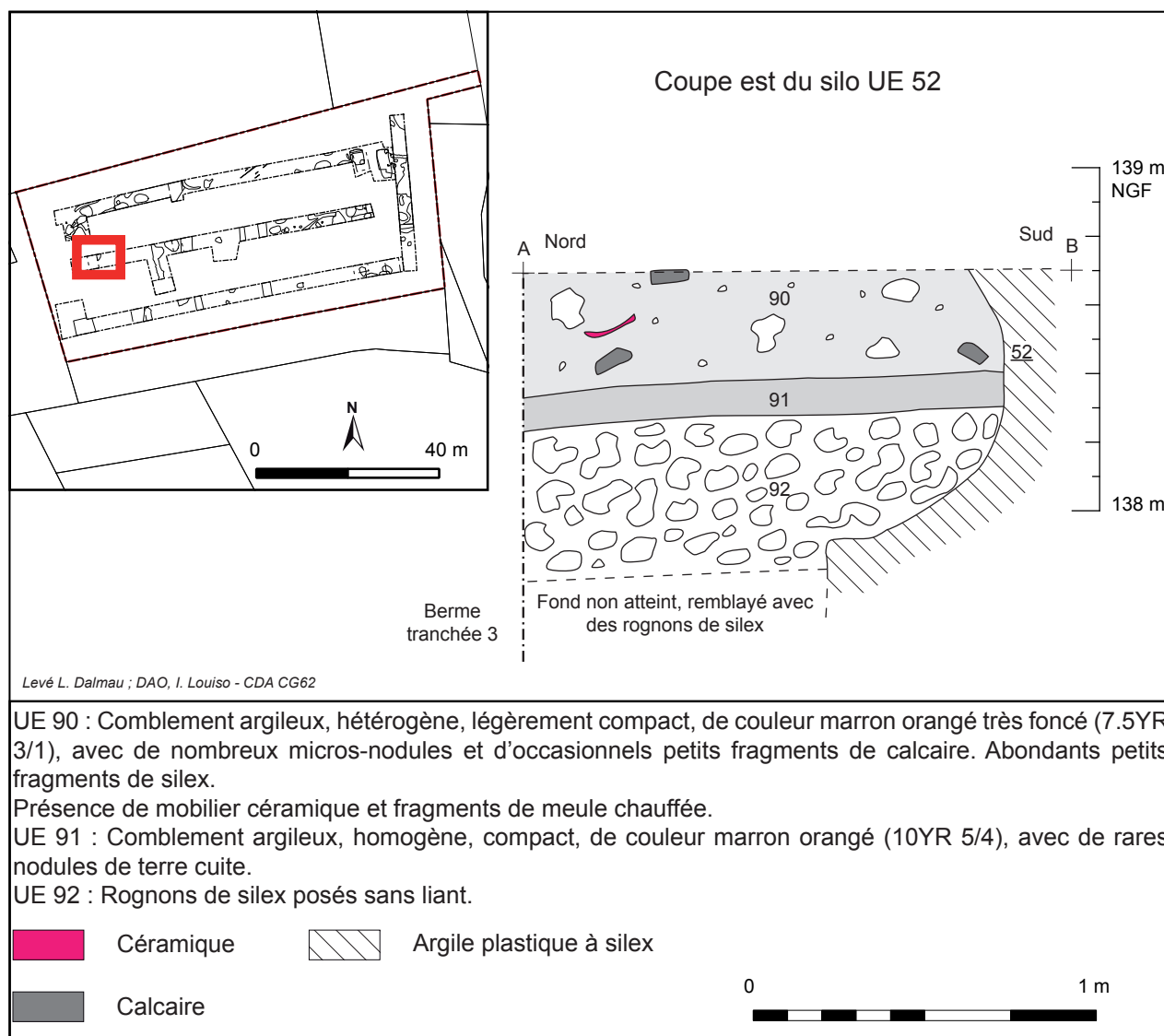
Fig. 60 : Bailleulmont, rue du château, Coupe est du silo UE 52, L. DALMAU - CDA - CG62
