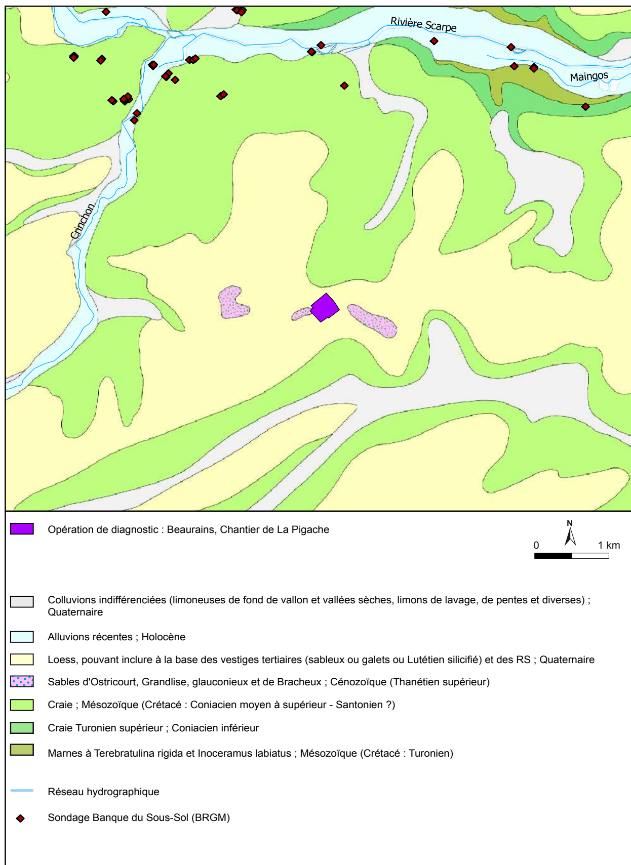
Fig. 6 : Beaurains, Chantier de la Pigache, extrait de la carte géologique au 1/50 000 harmonisée (BRGM- Infoterre 2011; Lacquement et al. 2004)
