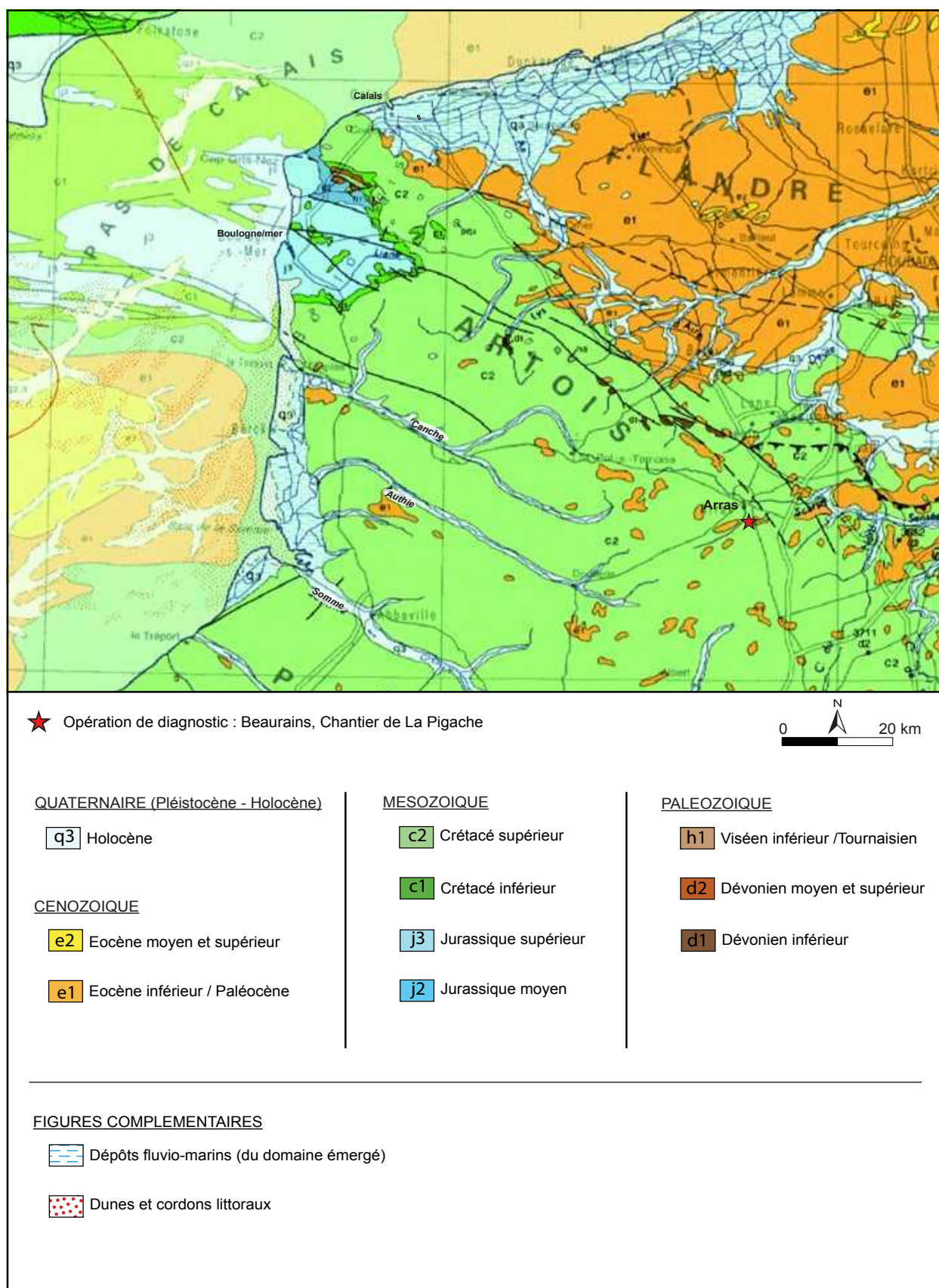
Fig. 5 : Beaurains, Chantier de la Pigache, extrait de la carte géologique au millionième (BRGM- Infoterre 2011; Chantraine et al. 1996)
